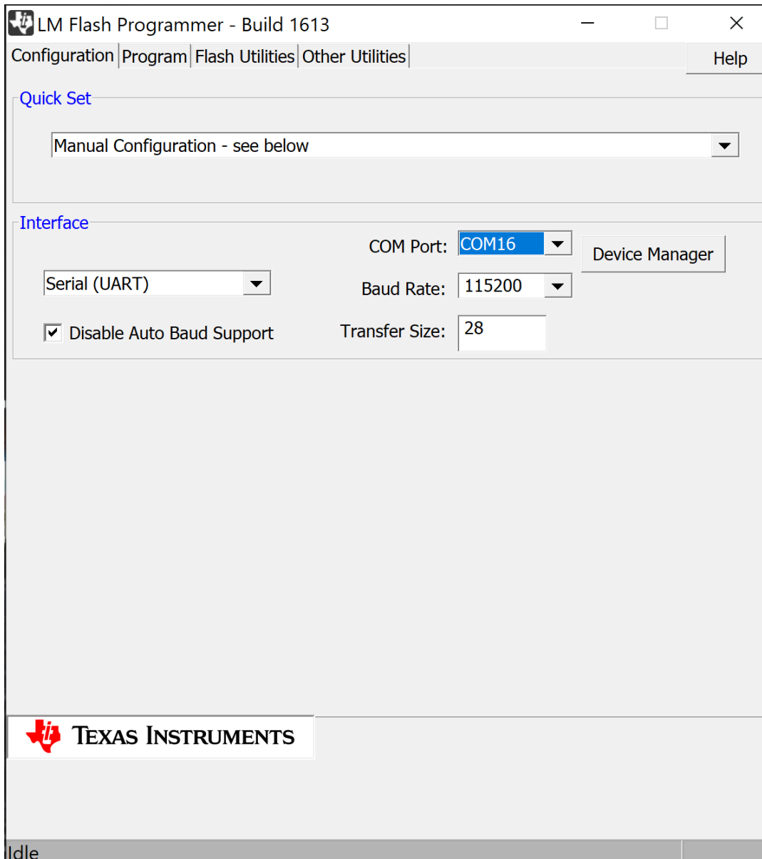
图 6-1. 配置 LM Flash Programmer
