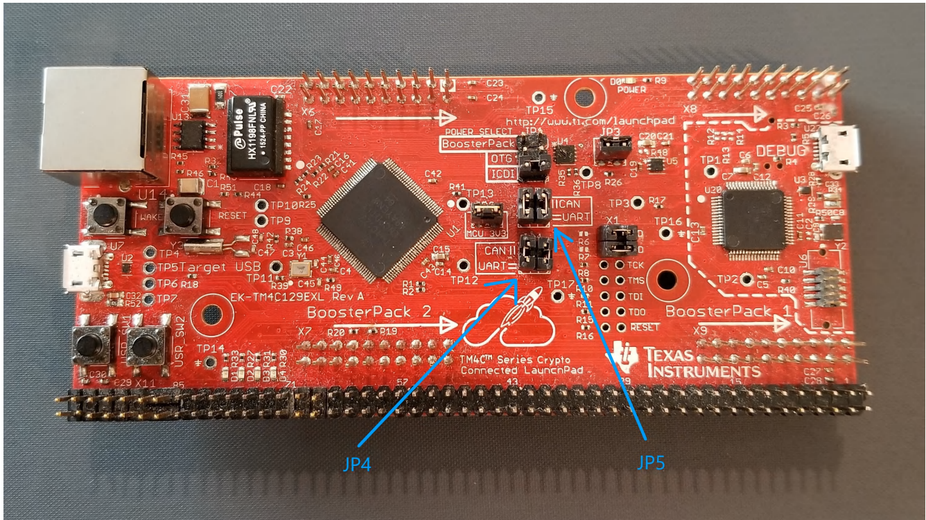
图 2-1. CAN 的 EK-TM4C1294XL 跳线位置
