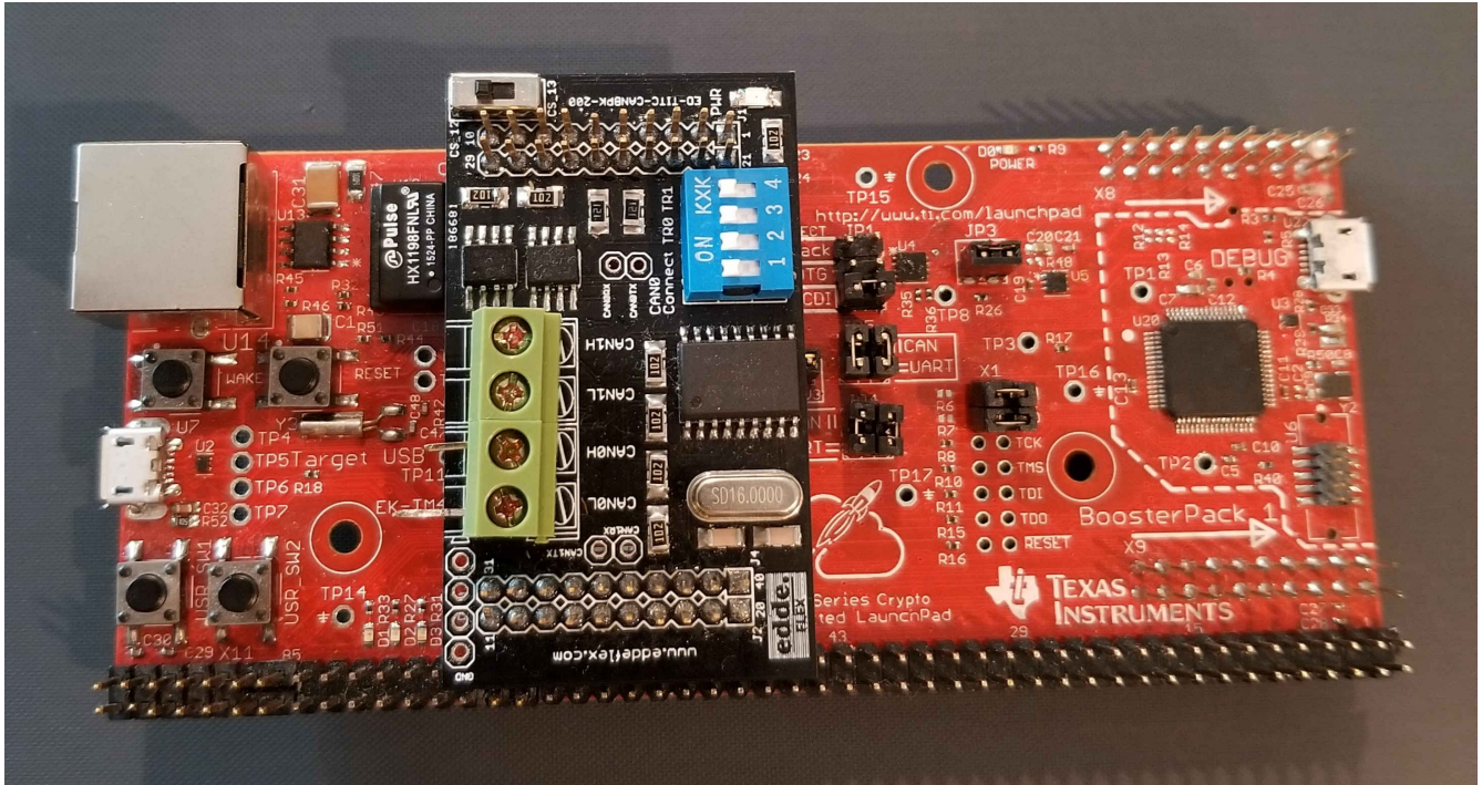
图 2-2. 带有 Edde Flex CAN BoosterPack 的 EK-TM4C1294XL
