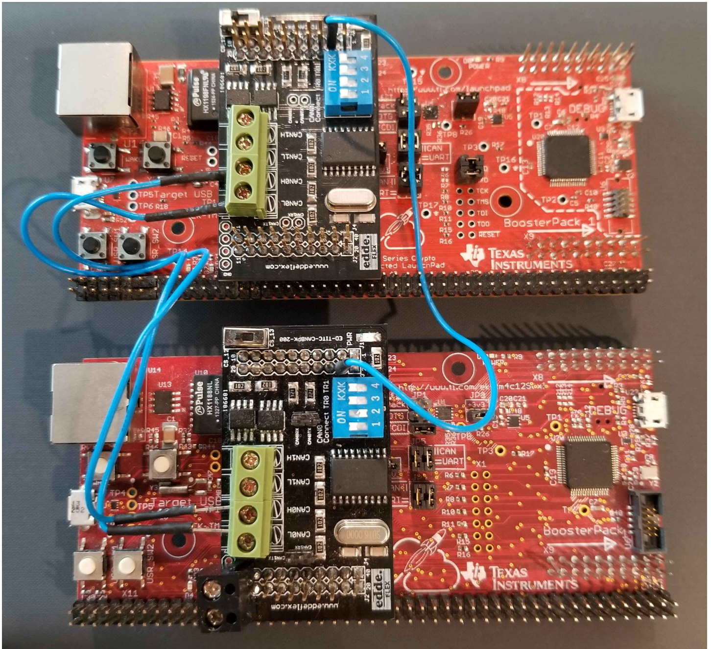
图 2-3. 双 EK-TM4C1294XL CAN 网络
