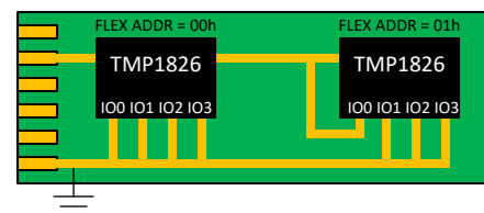
图 2. 使用 IO 调节存储器
