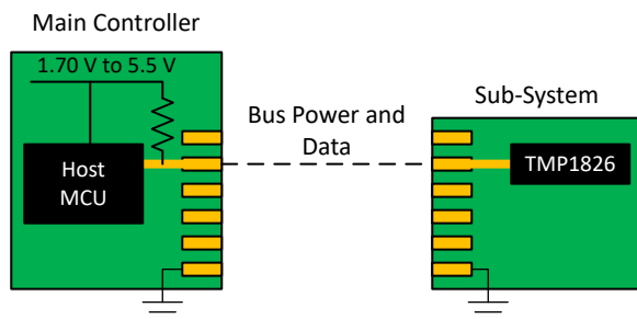
图 1. TMP1826 背板连接
