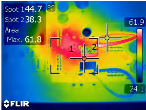
图 4-33. 单相降压中的热条件 ( V_{IN}=24V 且负载电流为 9A)
