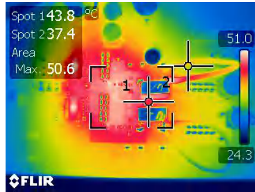
图 4-34. 双相降压中的热条件 ( V_{IN}=24V 且负载电流为 9A)
