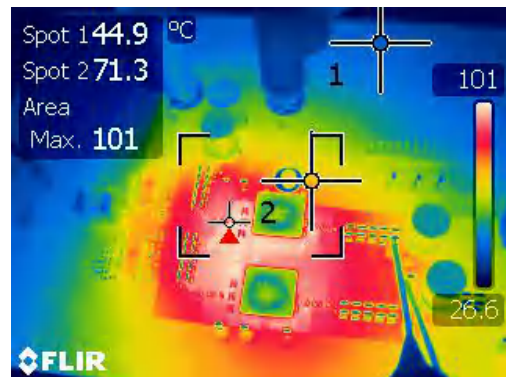
图 4-16. 降压/升压区域中的热条件 ( V_{IN}=16V 且负载电流为 18A)
