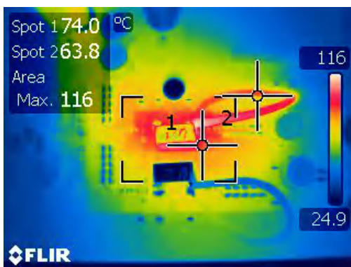
图 4-21. 单相升压中的热条件 ( V_{IN}=8V 且负载电流为 6A )
