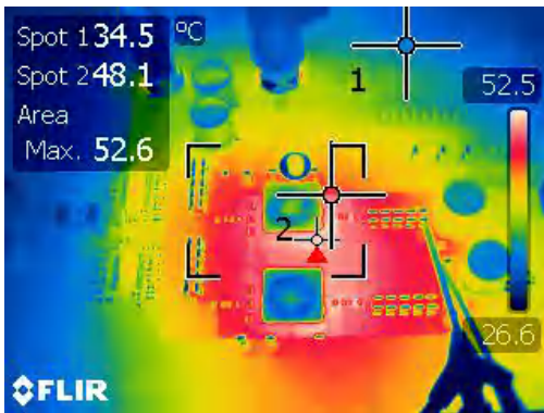
图 4-13. 升压区域中的热条件 ( V_{IN}=10V 且负载电流为 8A)
