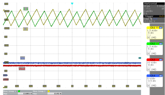
图 4-4. 升压区域中的电感器电流 ( V_{IN}=8V 且负载电流为 10A)
