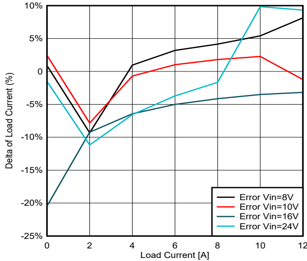
图 4-1. 负载电流误差
