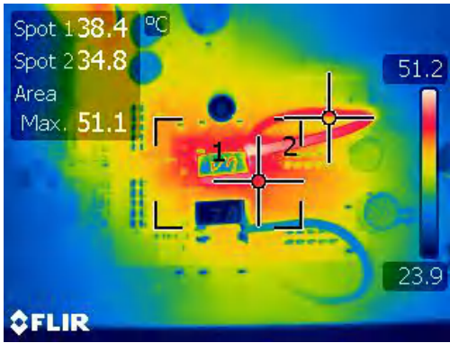
图 4-23. 单相升压中的热条件 ( V_{IN}=10V 且负载电流为 4A)
