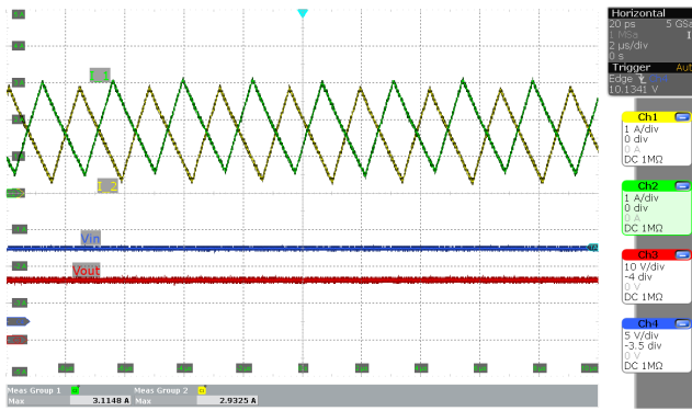
图 4-5. 升压区域中的电感器电流 ( V_{IN}=10V 且负载电流为 2A )
