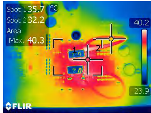
图 4-24. 双相升压中的热条件 ( V_{IN}=10V 且负载电流为 4A)
