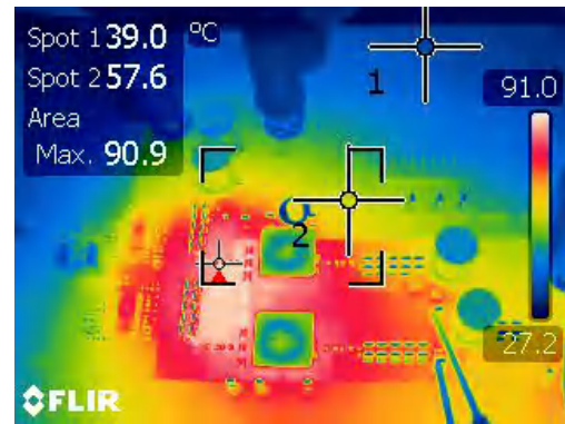
图 4-18. 降压区域中的热条件 ( V_{IN}=24V 且负载电流为 18A )
