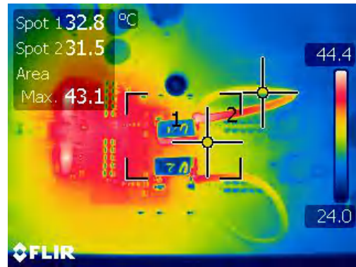
图 4-32. 双相降压中的热条件 ( V_{IN}=24V 且负载电流为 4A)
