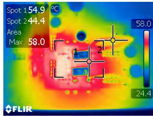
图 4-30. 双相降压/升压中的热条件 ( V_{IN}=16V 且负载电流为 9A)
