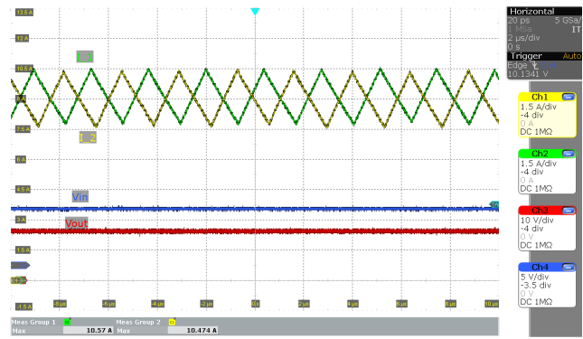
图 4-6. 升压区域中的电感器电流 ( V_{IN}=10V 且负载电流为 10A )
