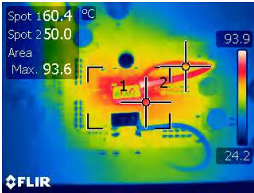
图 4-25. 单相升压中的热条件 ( V_{IN}=10V 且负载电流为 7A)
