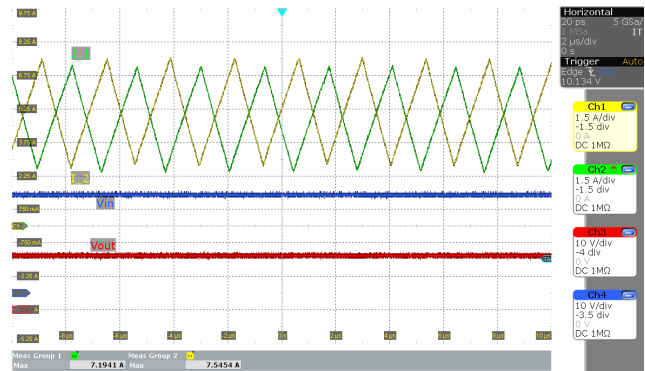
图 4-10. 降压区域中的电感器电流 ( V_{IN}=30V 且负载电流为 10A )
