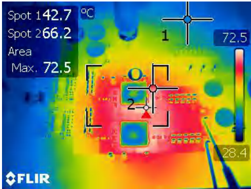
图 4-11. 升压区域中的热条件 ( V_{IN}=8V 且负载电流为 8A)
