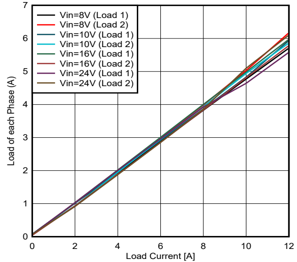
图 4-2. 两相负载分配
