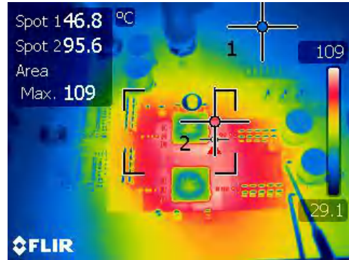
图 4-12. 升压区域中的热条件 ( V_{IN}=8V 且负载电流为 12A)
