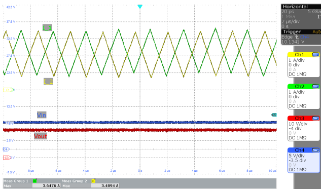
图 4-3. 升压区域中的电感器电流 ( V_{IN}=8V 且负载电流为 2A)
