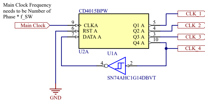
图 2-4. 多相位时钟发生器
