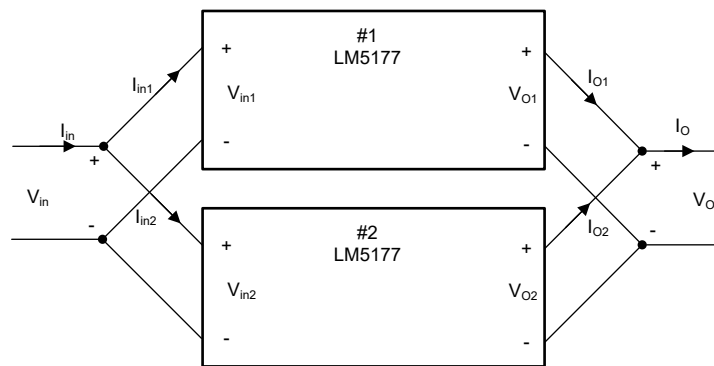
图 2-1. 两个并联 LM5177 转换器作为电源
