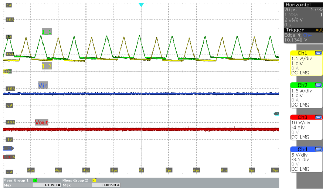
图 4-7. 降压/升压区域中的电感器电流 ( V_{IN}=16V 且负载电流为 2A )
