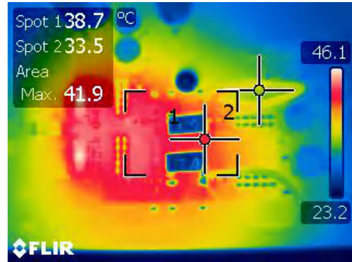
图 4-28. 双相降压/升压中的热条件 ( V_{IN}=16V 且负载电流为 4A)
