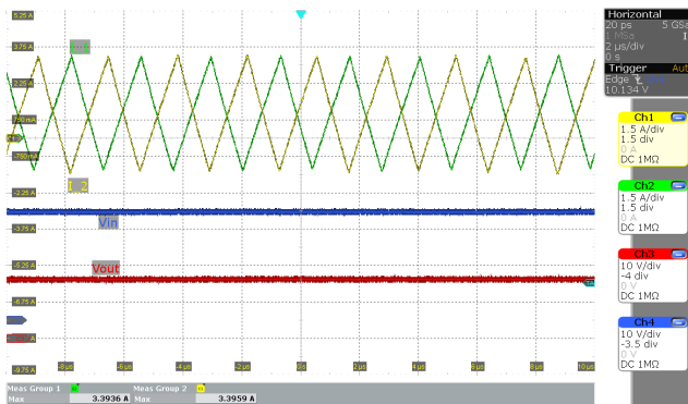
图 4-9. 降压区域中的电感器电流 ( V_{IN}=30V 且负载电流为 2A )
