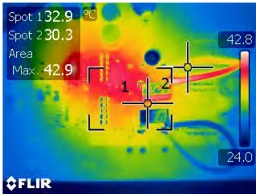
图 4-31. 单相降压中的热条件 ( V_{IN}=24V 且负载电流为 4A)
