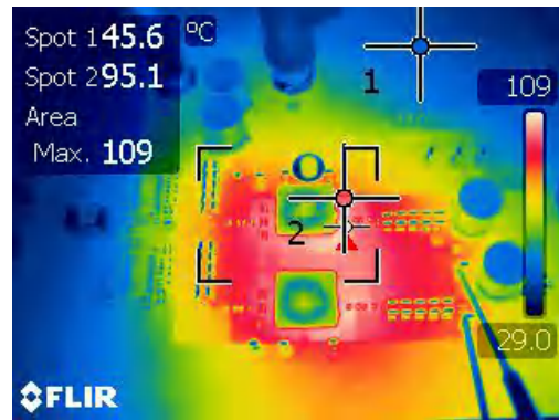
图 4-14. 升压区域中的热条件 ( V_{IN}=10V 且负载电流为 14A)
