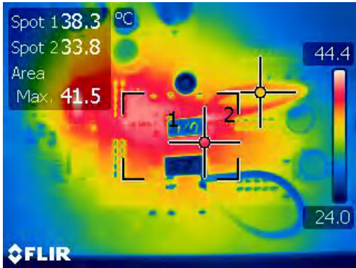
图 4-27. 单相降压/升压中的热条件 ( V_{IN}=16V 且负载电流为 4A)
