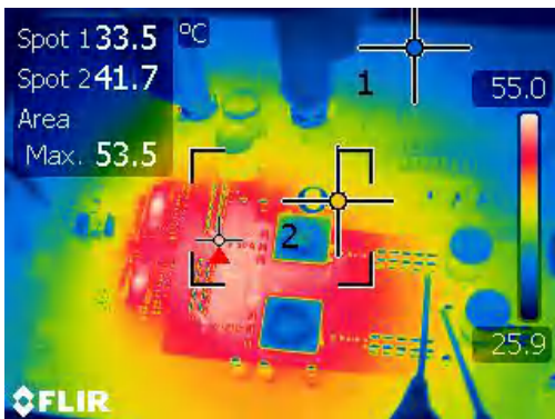
图 4-15. 降压/升压区域中的热条件 ( V_{IN}=16V 且负载电流为 8A)
