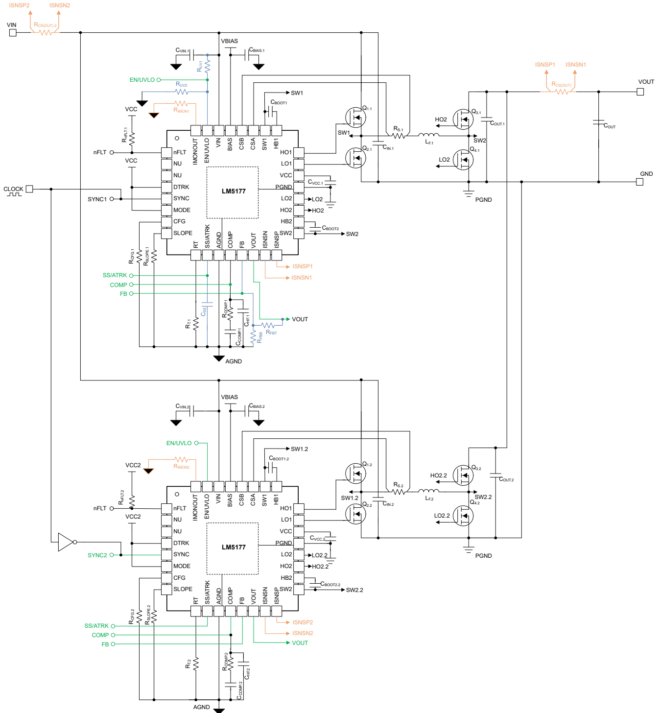
图 3-1. 两个 LM5177 并联运行的方框图
