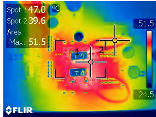
图 4-26. 双相升压中的热条件 ( V_{IN}=10V 且负载电流为 7A)
