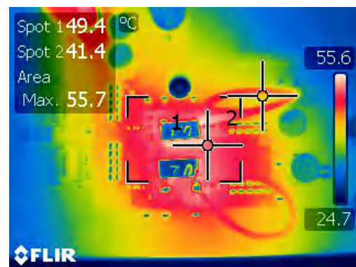
图 4-22. 双相升压中的热条件 ( V_{IN}=8V 且负载电流为 6A )
