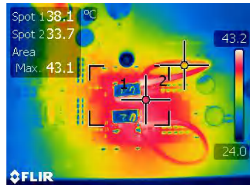
图 4-20. 双相升压中的热条件 ( V_{IN}=8V 且负载电流为 4A )
