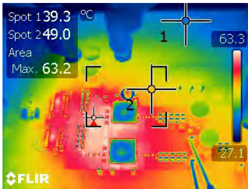
图 4-17. 降压区域中的热条件 ( V_{IN}=24V 且负载电流为 8A )
