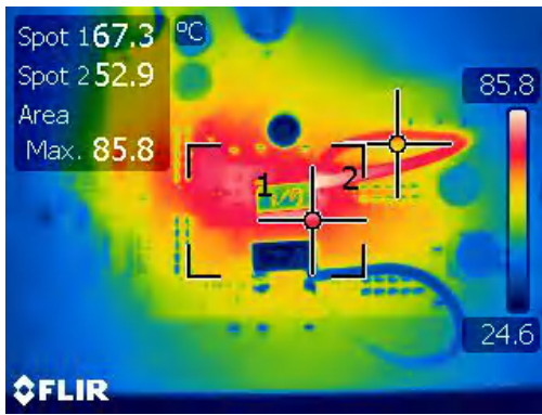
图 4-29. 单相降压/升压中的热条件 ( V_{IN}=16V 且负载电流为 9A)
