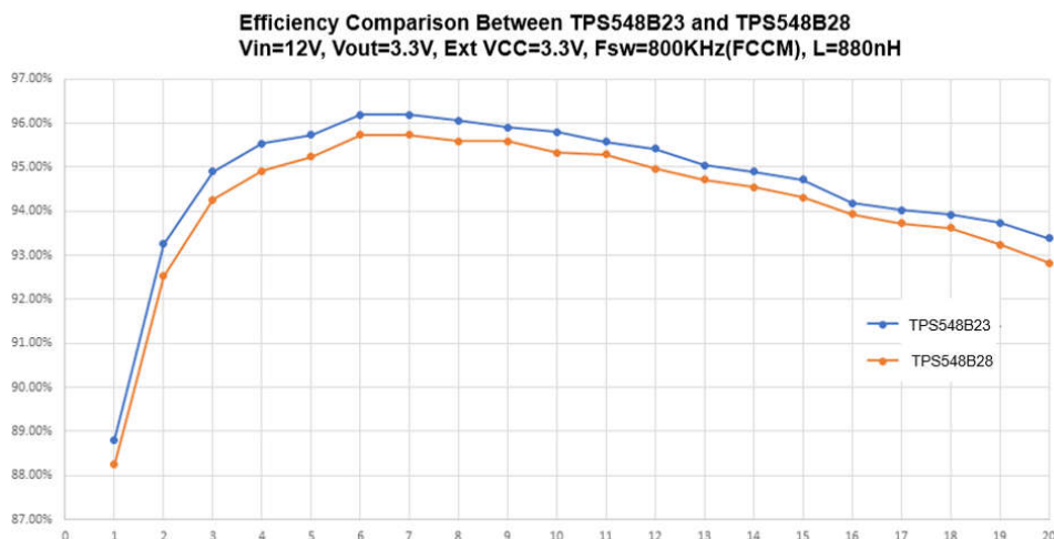
图 1. TPS548B23 与 TPS548B28 的效率比较
