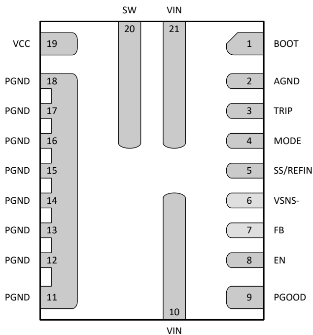
图 4. TPS548B28 封装底视图 - 非对称引脚排列
