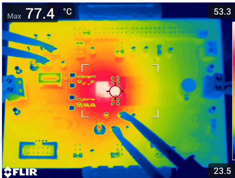
图 2. TPS548B23EVM 在 12Vin、1Vout、800kHz、20A 时的热成像图
