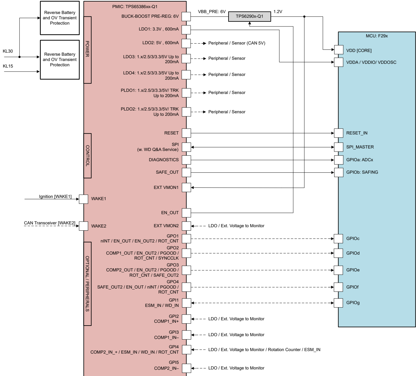
图 2-1. TIPA-050073 电源连接
