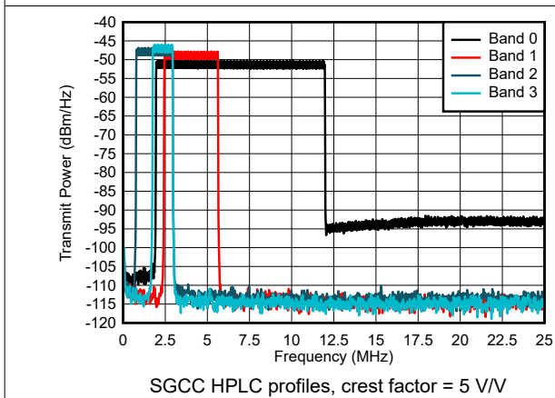
图 5-3. Out-of-Band Suppression
