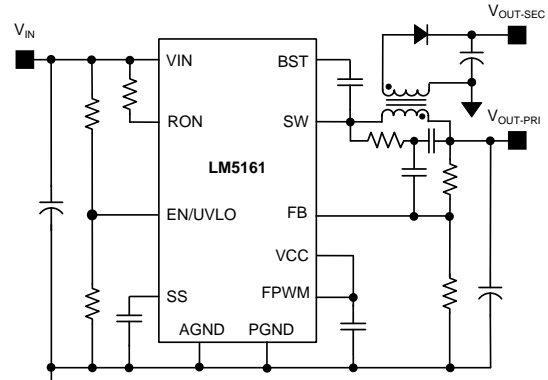
典型 Fly-Buck 应用电路
