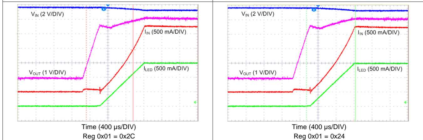
图 72. Boost Edge Triggered Flash
