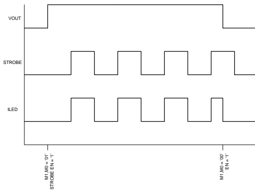
图 30. IR Mode Pass Only
