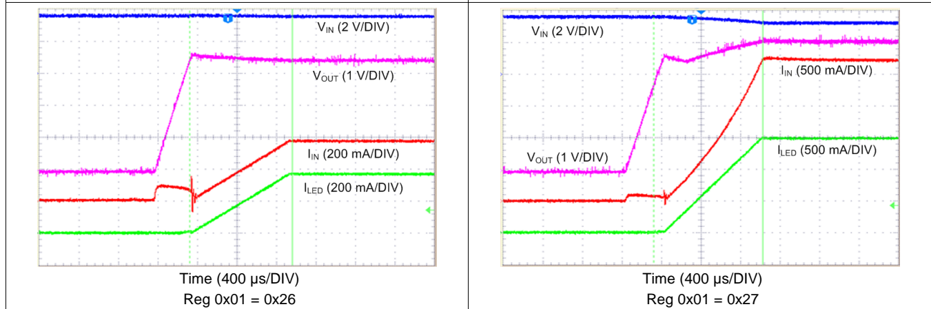
图 70. Boost I 2 C Torch
