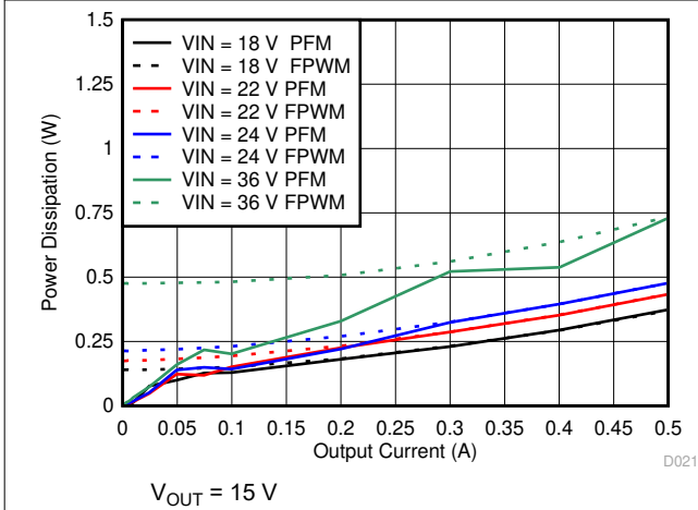
图 7-9. Power Dissipation
