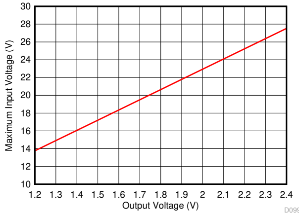
图 7-1. Maximum Input Voltage for V_{OUT} < 2.5\text{V}
