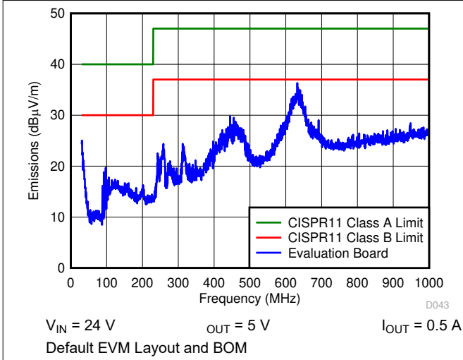
图 7-7. Radiated EMI
