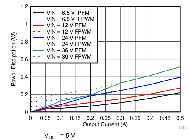
图 7-11. Power Dissipation
