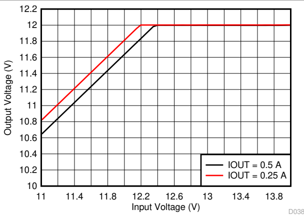
图 7-3. Dropout Voltage
