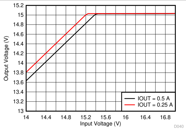
图 7-4. Dropout Voltage
