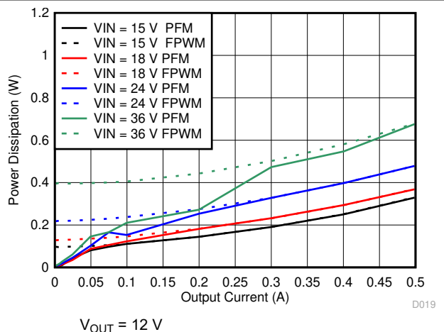
图 7-10. Power Dissipation
