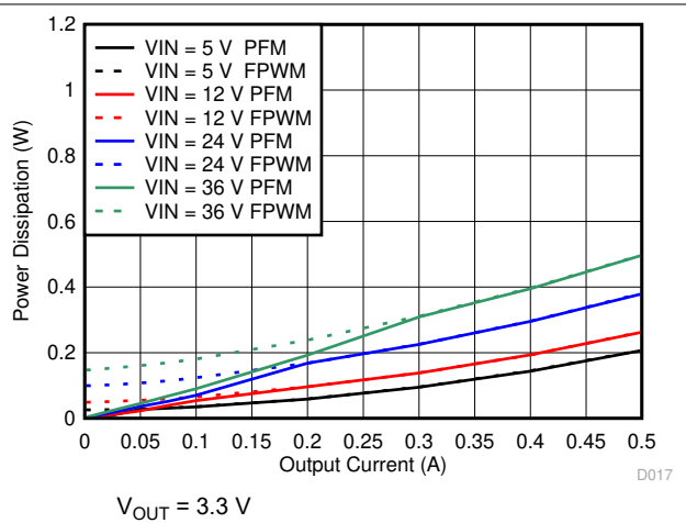
图 7-12. Power Dissipation
