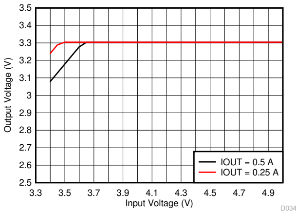
图 7-3. Dropout Voltage
