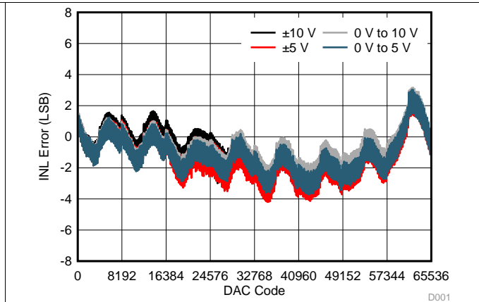
图 4. VOUT INL vs Code (DC/DC Enabled)
