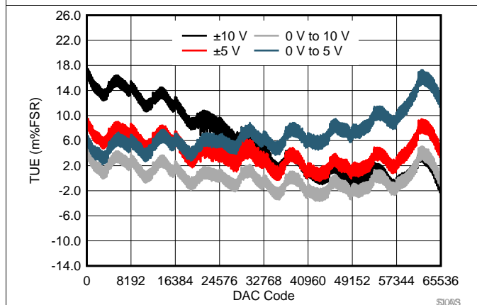
图 7. VOUT TUE vs Code (DC/DC Enabled)
