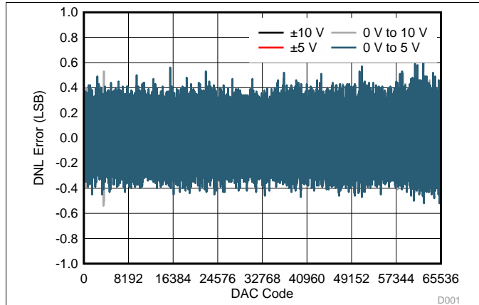
图 3. VOUT DNL vs Code (DC/DC Enabled)
