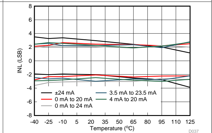
图 41. IOUT INL vs Temperature
