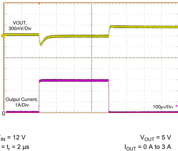
图 9-23. Load Transient
