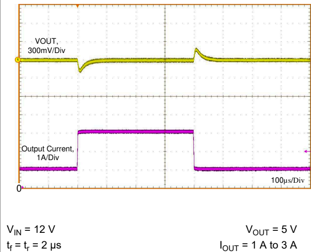
图 9-24. Load Transient
