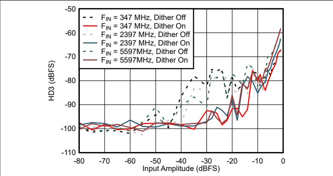
图 6-62. DES Mode: HD3 vs Input Amplitude and Dither
