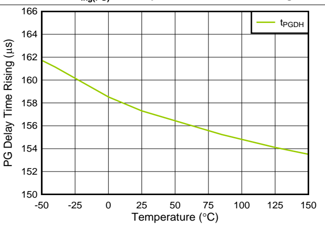
图 18. t_{PGDH} vs Temperature
