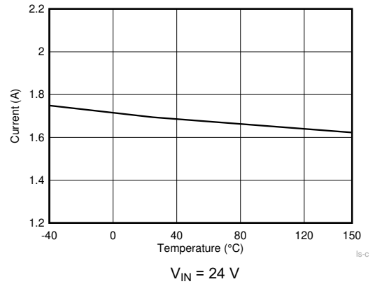
图 8-4. Low Side Current Limit
