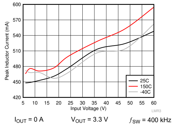
图 8-6. I_{PEAK-MIN}
