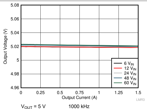
图 10-29. Load Regulation
