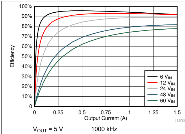
图 10-28. Efficiency
