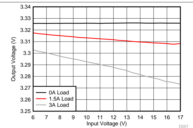
图 19. Line Regulation
