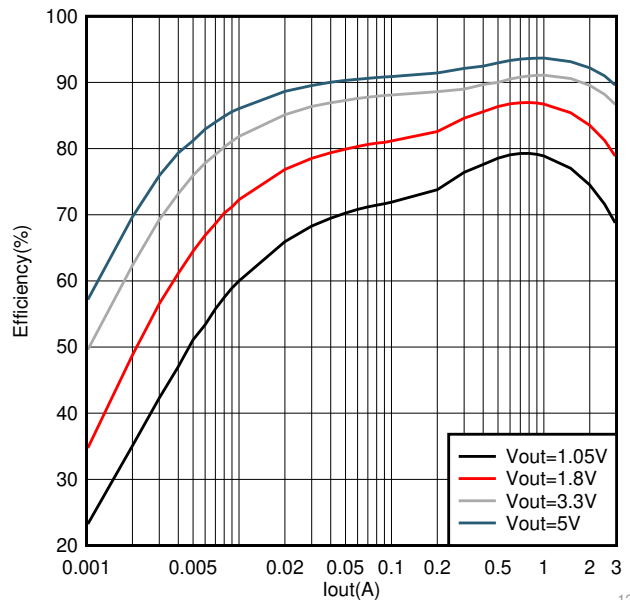
TPS563231 效率
