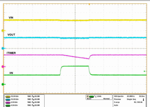
图 9-5. Transient Overload
