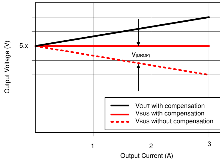
图 10-8. 压降
