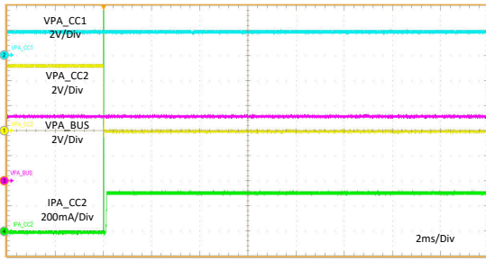
图 11-27. PA_CC2 热短接至 GND
