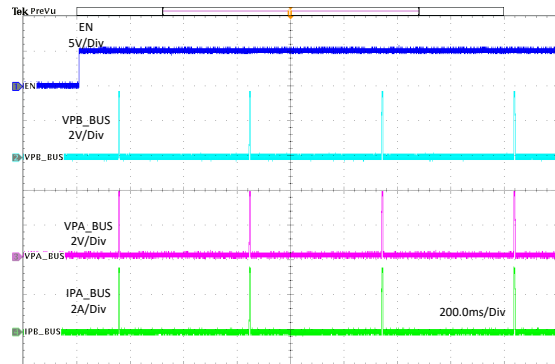
EN 至高电平 PA_BUS = 1\Omega PB_BUS = 1\Omega
