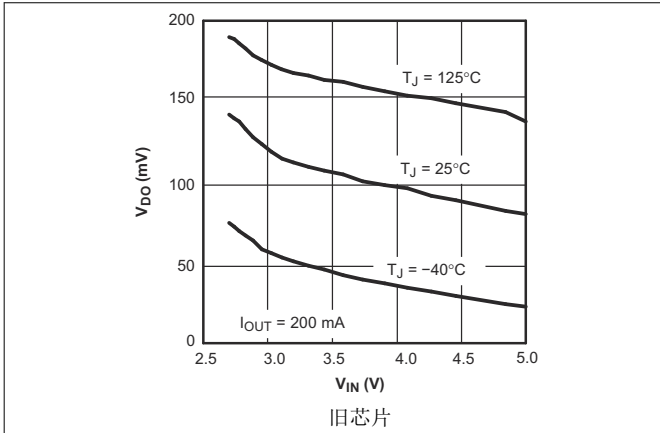
图 5-31. TPS793 压降电压与输入电压间的关系
