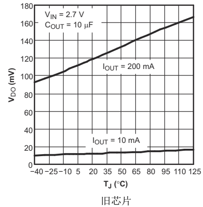
图 5-14. TPS793 压降电压与结温间的关系
