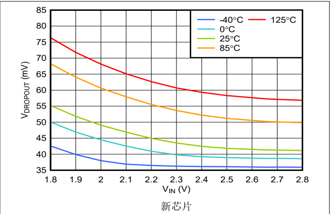
图 5-32. TPS793 压降电压与输入电压间的关系
