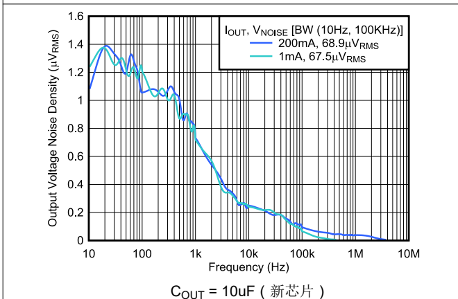
图 5-11. TPS793 输出频谱噪声密度与频率间的关系
