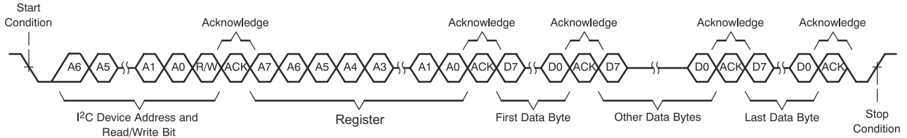
图 7-65. I 2 C Multiple-Byte Write Transfer
