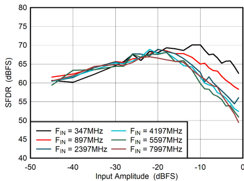
图 6-59. DES Mode: SFDR vs Input Amplitude
