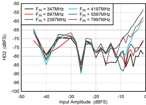
图 6-61. DES Mode: HD2 vs Input Amplitude
