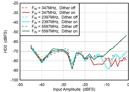
图 6-62. DES Mode: HD2 vs Input Amplitude and Dither
