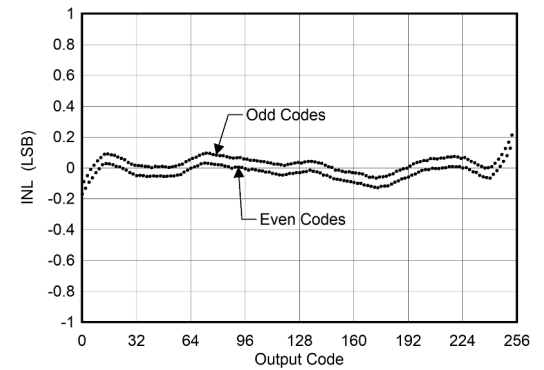
图 6-4. INL vs ADC Code
