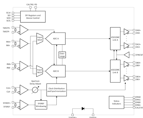
ADC08DJ5200RF 方框图
