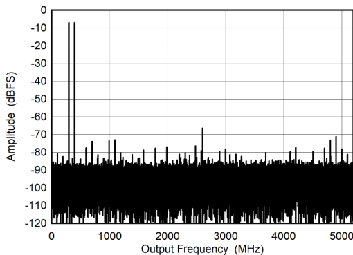
图 6-11. DES Mode: Two Tone FFT at 347 MHz
