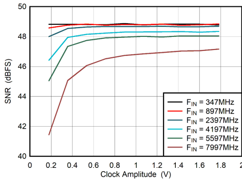
图 6-81. DES Mode: SNR vs Clock Amplitude
