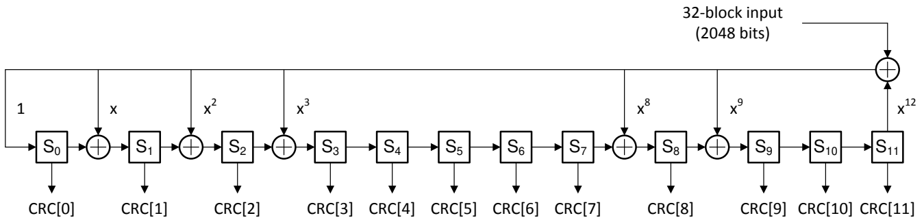
图 7-10. CRC-12 Parity Bit Generator
