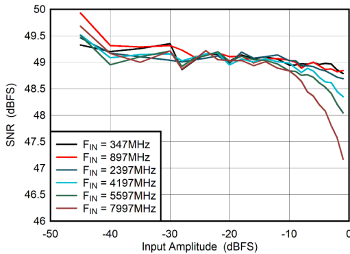
图 6-57. DES Mode: SNR vs Input Amplitude
