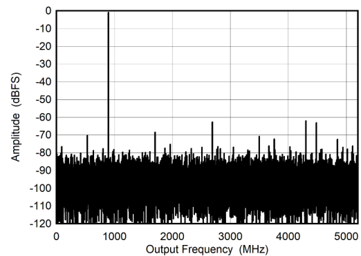
图 6-6. DES Mode: Single Tone FFT at 897 MHz
