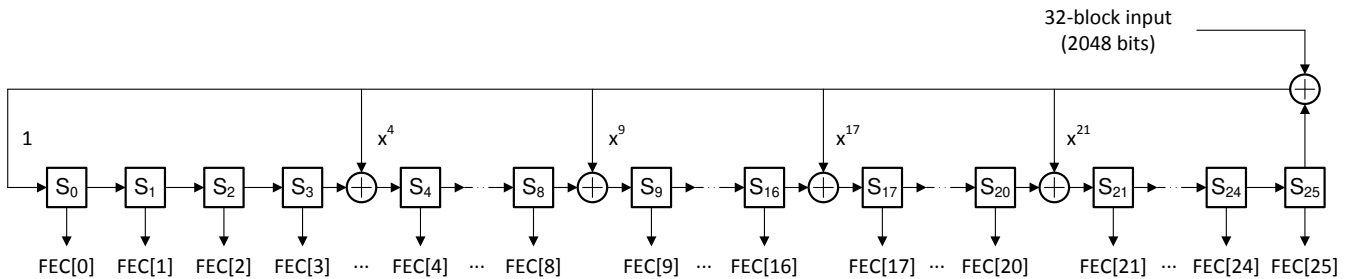
图 7-11. FEC Parity Bit Generator
