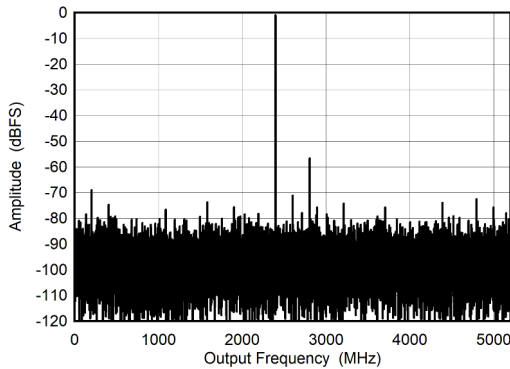
图 6-7. DES Mode: Single Tone FFT at 2397 MHz
