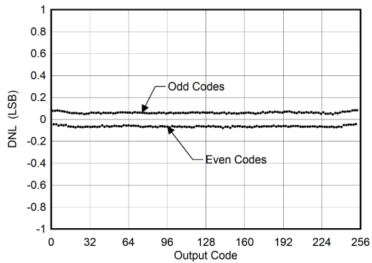
图 6-3. DNL vs ADC Code
