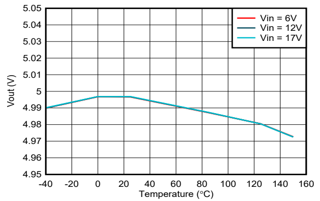
图 7-4. Output Voltage Accuracy - VSET Selected
