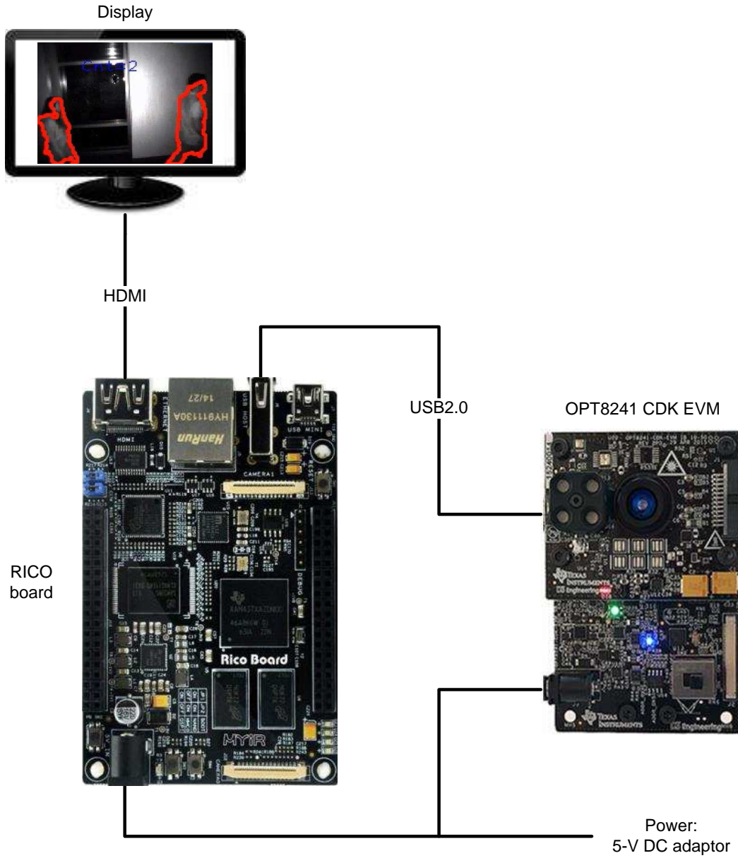
图 15. Hardware Setup
