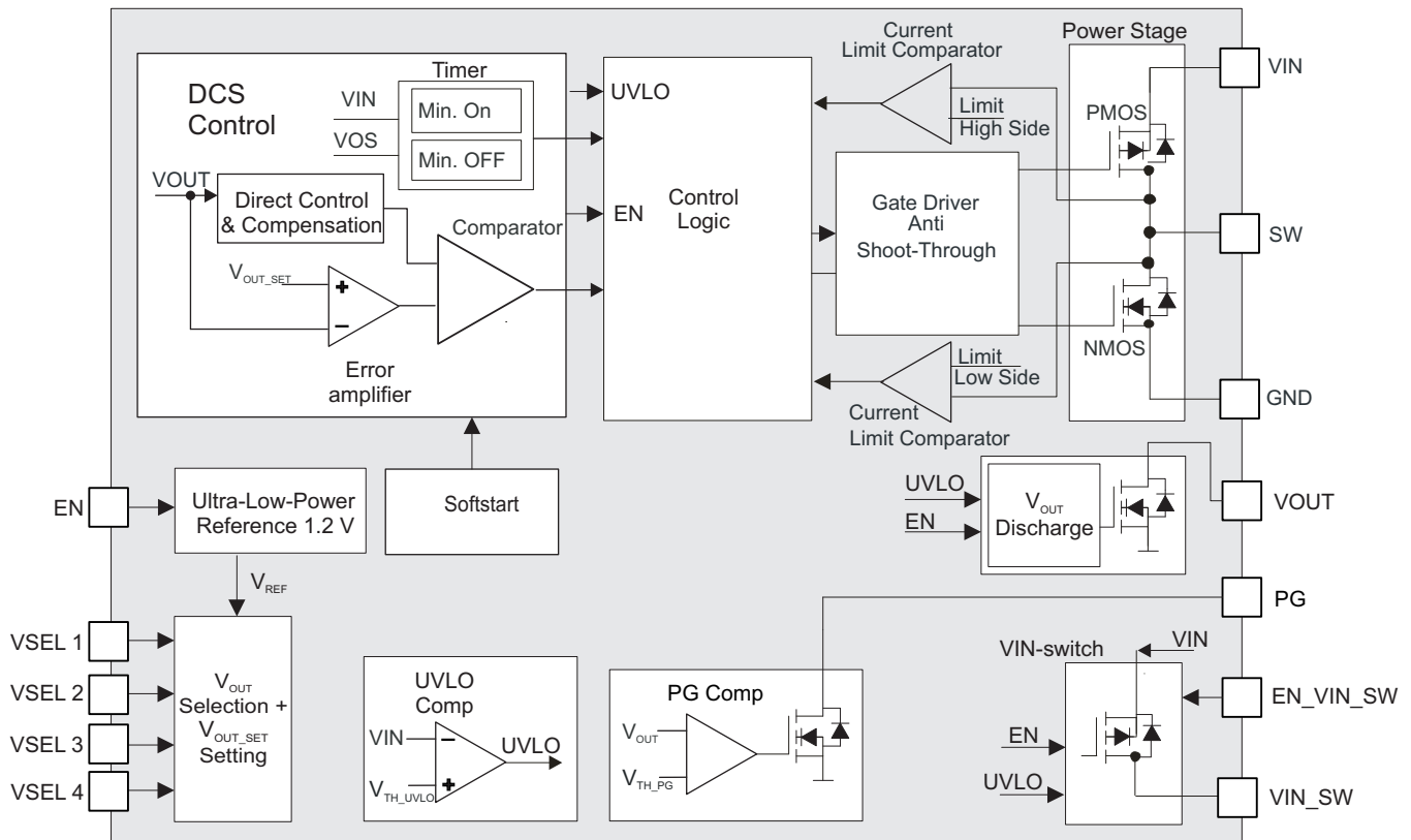
图 3. TPS62745 Block Diagram
