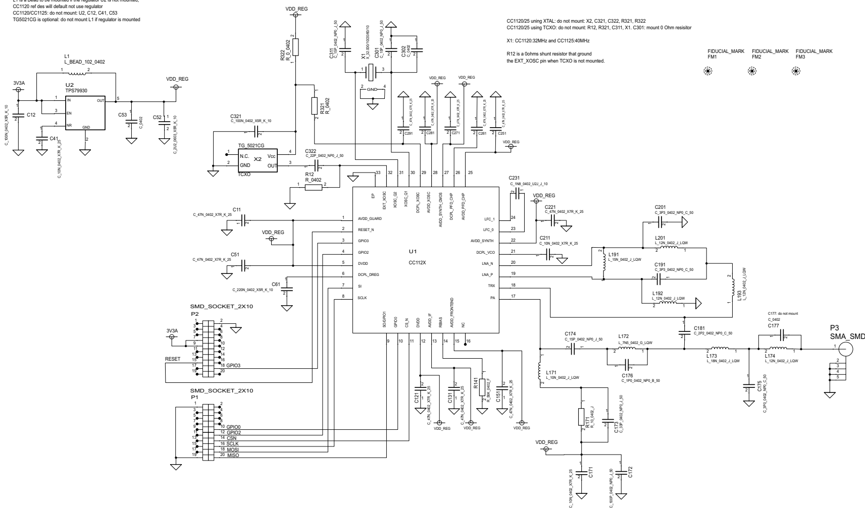
图 14. TIDC-DSSS868WMBUS-DC Schematic
