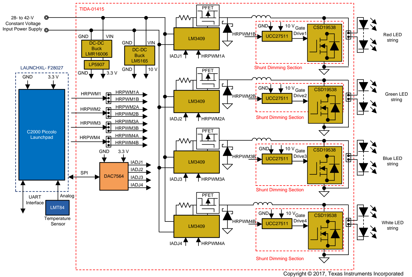
图 4. TIDA-01415 Block Diagram
