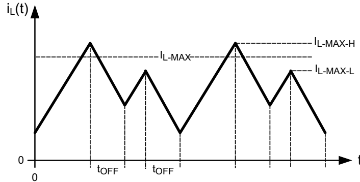
图 13. Inductor Current i_L(t) Showing I_{L-MAX} Offset
