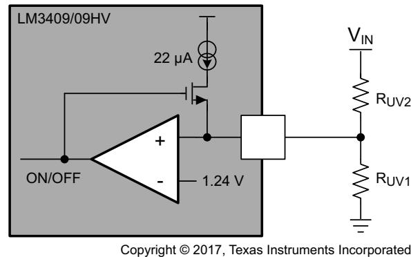
图 11. UVLO Circuit of LM3409
