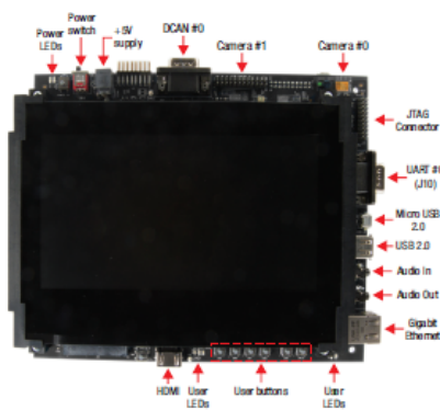
图 7. AM437x GP EVM Top View
