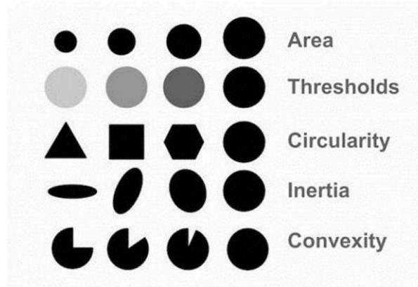
图 12. Blob Parameters[9]
