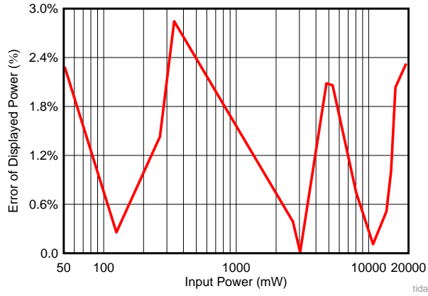
图 21. Input Power Accuracy
