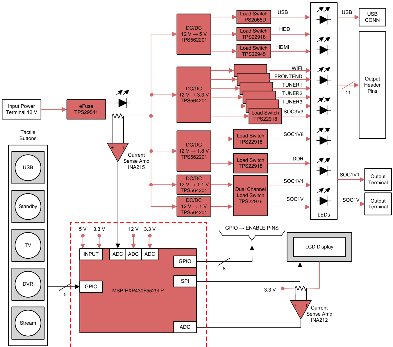
图 1. TIDA-01451 Block Diagram
