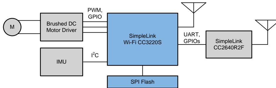
图 1. TIDC-01005 Block Diagram
