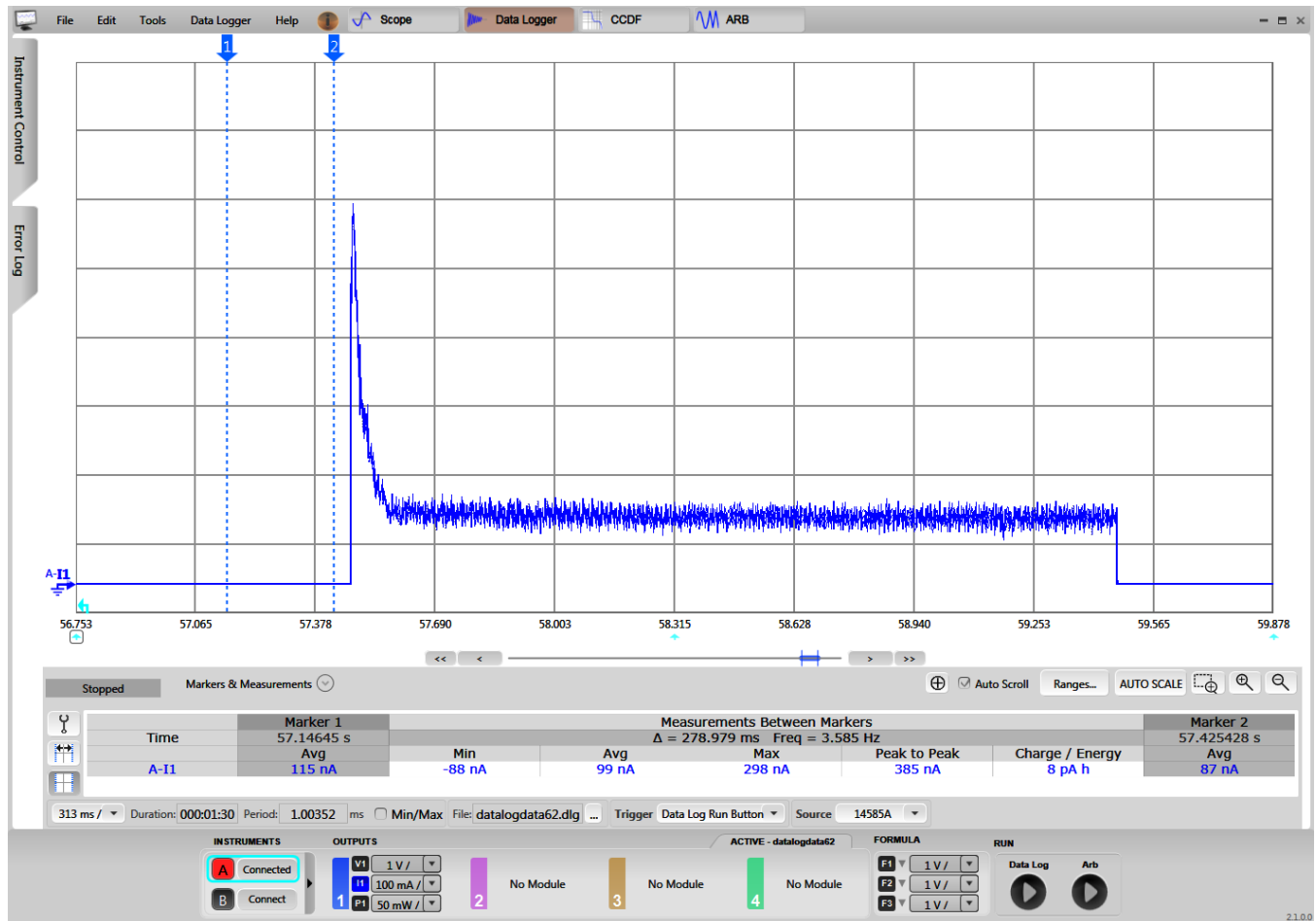
图 32. DRV8837 Sleep Current
