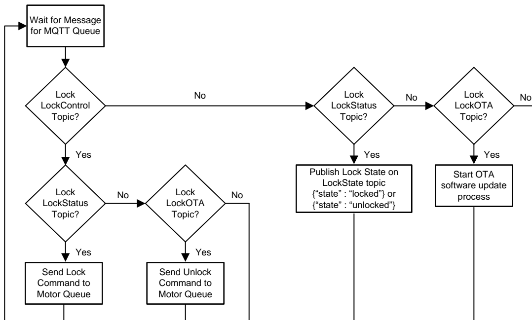
图 9. MQTT Message Handling
