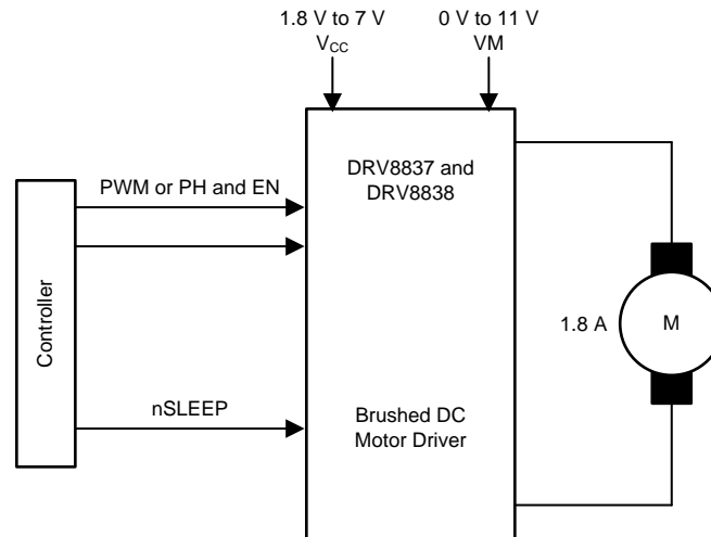
图 2. DRV8837 Simplified Diagram
