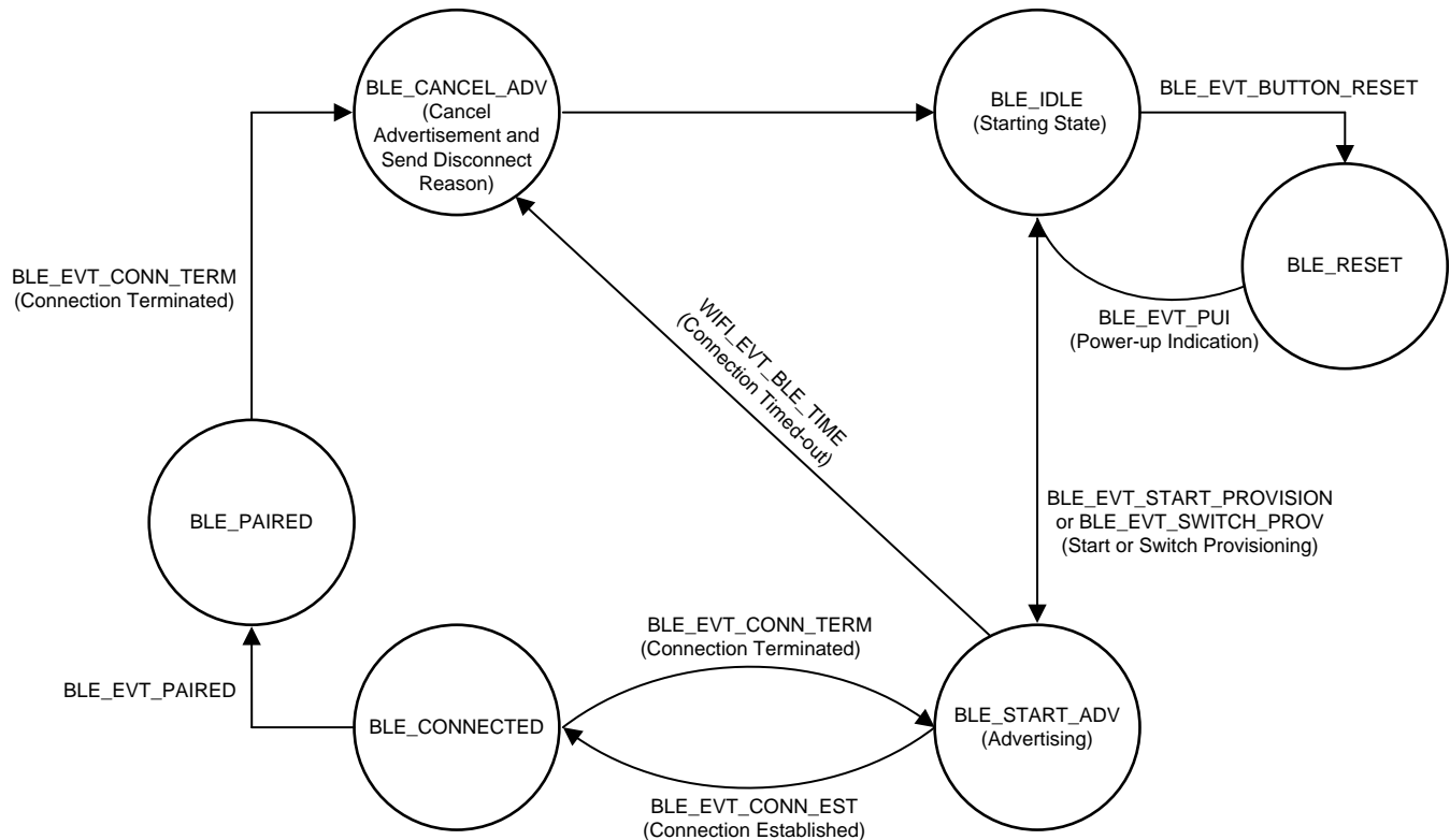
图 7. BLE Provisioning State Machine
