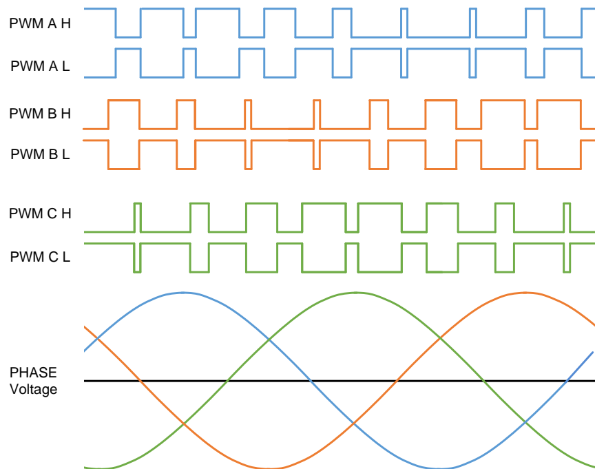
图 2. 生成理想的 PWM 到正弦相电压
