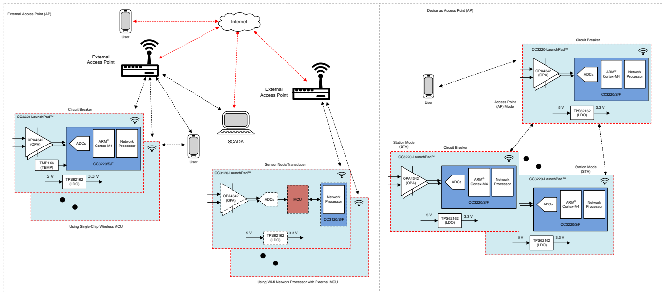
图 2. TIDA-010007 Block Diagram
