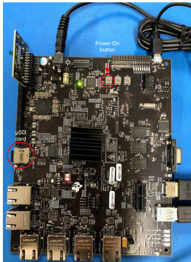
图 9. AM574x IDK EVM
