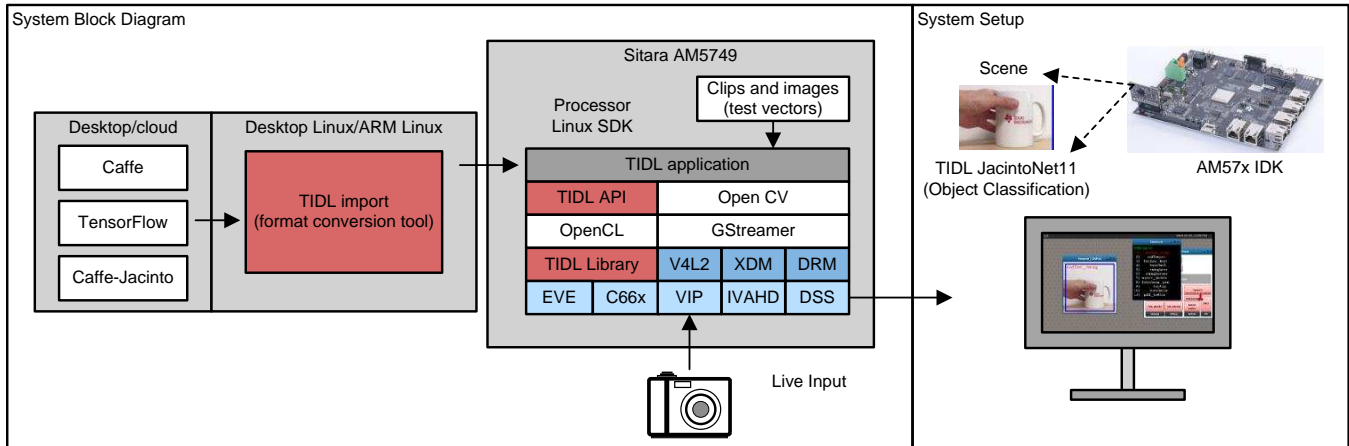
图 2. TIDEP-01004 Block Diagram
