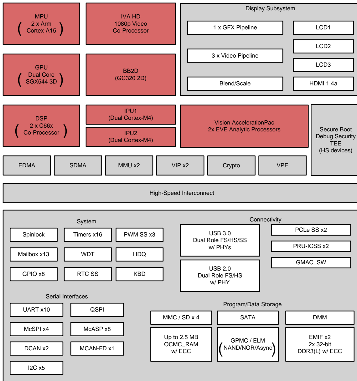
图 1. AM574x Block Diagram
