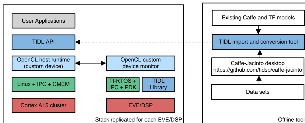
图 8. TIDL Software Stack
