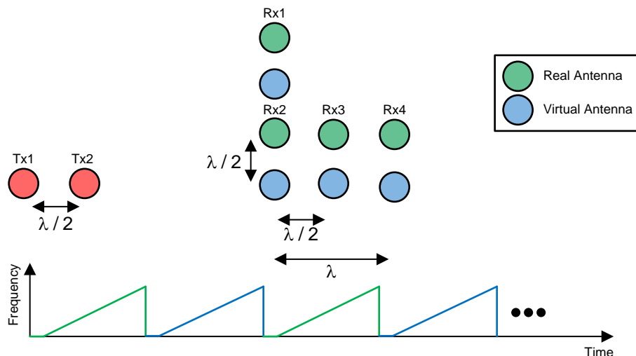
图 3. ODS EVM-Antenna Configuration
