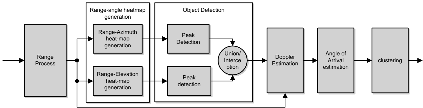
图 1. Block Diagram
