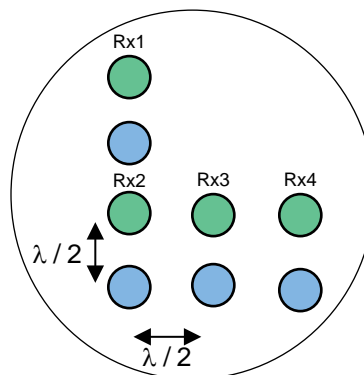
图 7. Angle Spectrum
