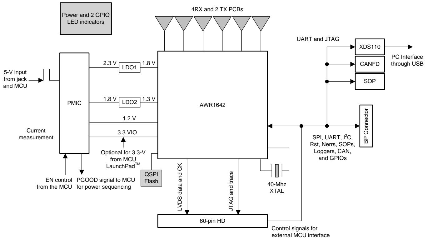
图 2. AWR1642 EVM Block Diagram
