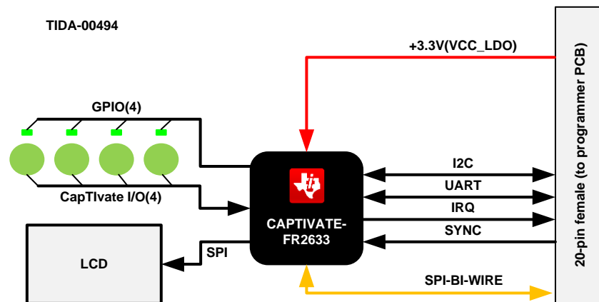
图 1. TIDA-00494 Block Diagram
