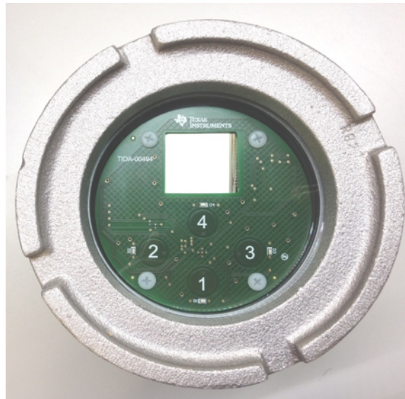
图 15. TIDA-00494 Final Test Setup
