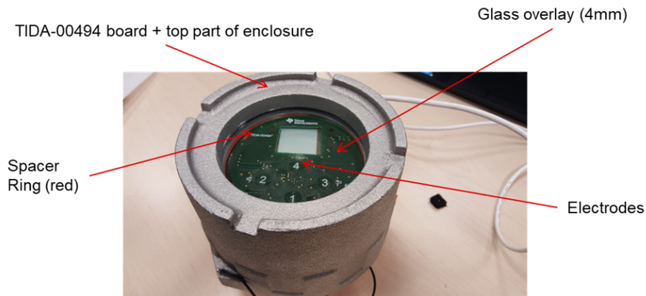
图 26. Test Setup
