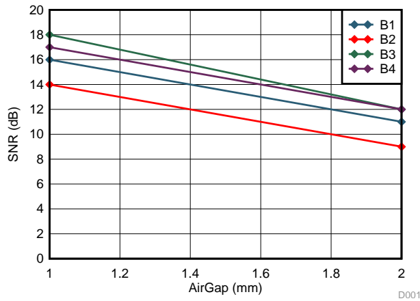
图 19. Finger Touch—SNR
