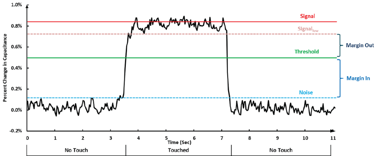
图 28. Signal-Margin-Definition
