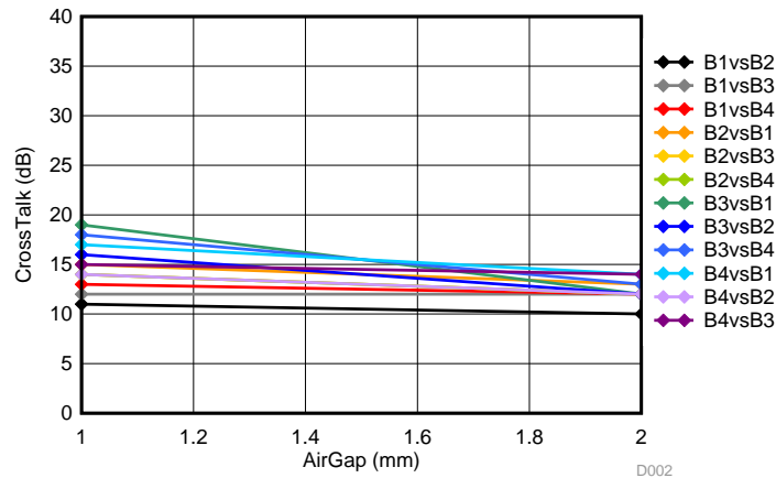
图 20. Finger Touch Crosstalk
