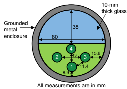
图 6. Button Configuration
