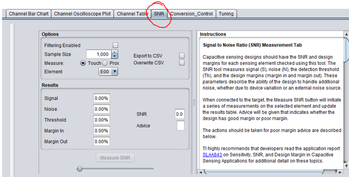
图 27. SNR Tool
