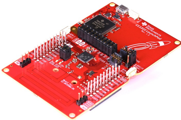
图 7. LAUNCHXL-CC1310
