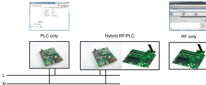
图 18. Hybrid RF/PLC Test Setup
