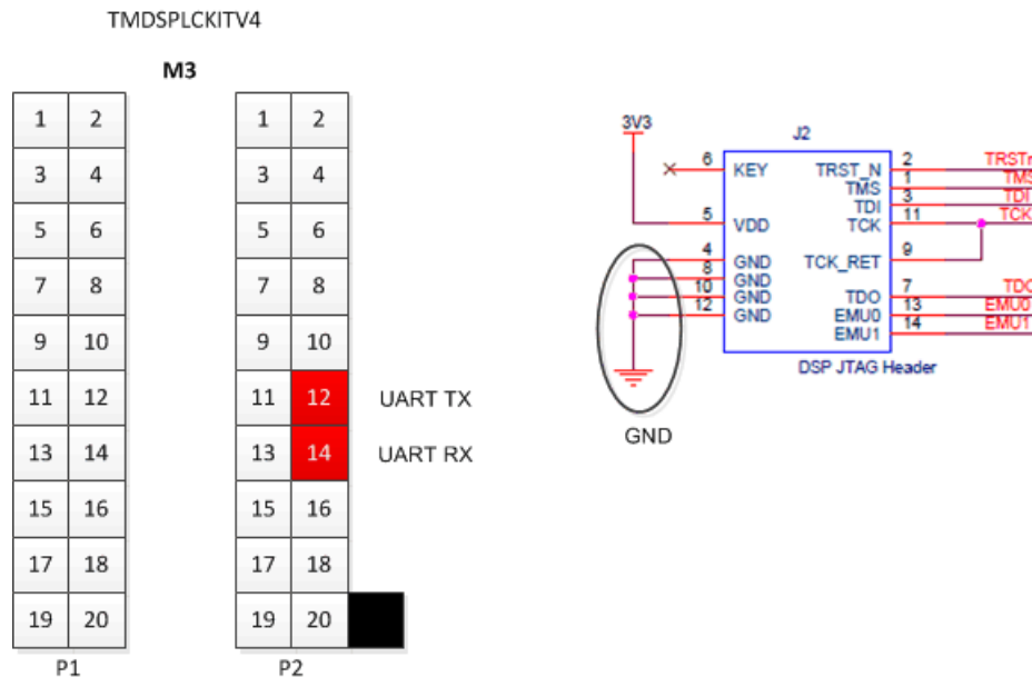
图 9. UART Pins on TMDSPCKITV4
