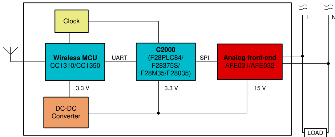
图 3. Block Diagram
