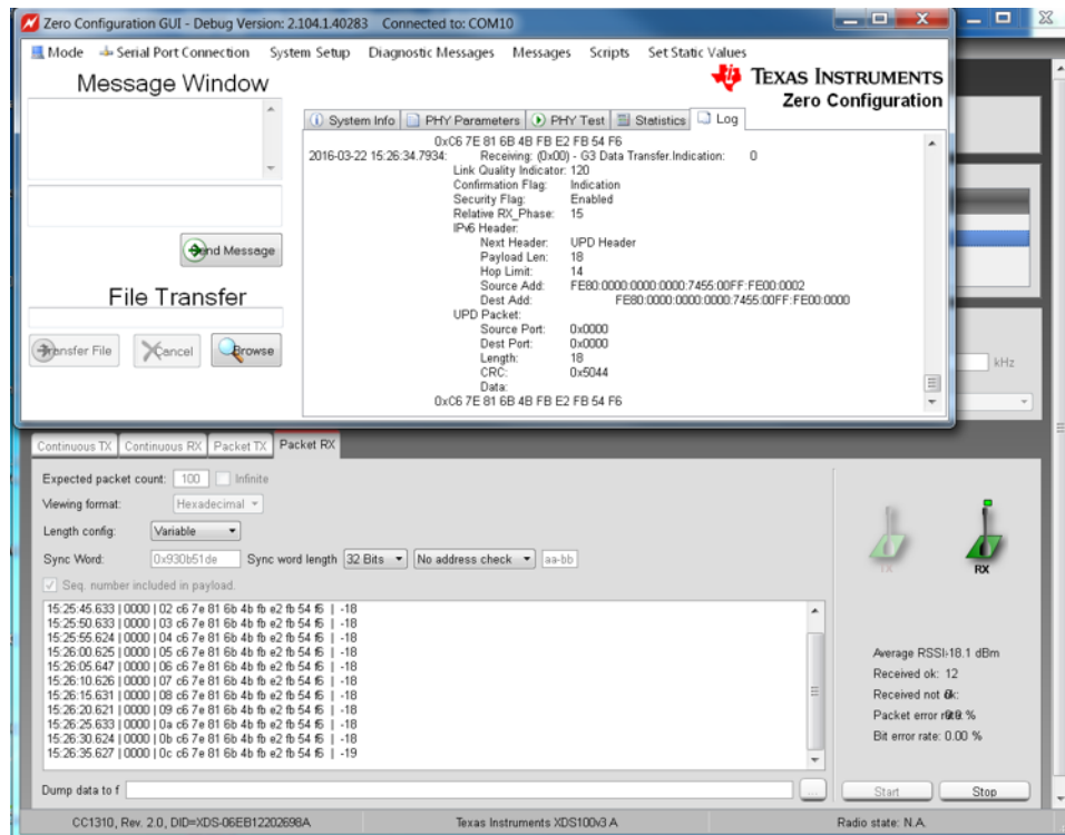
图 27. Simultaneous Transmissions
