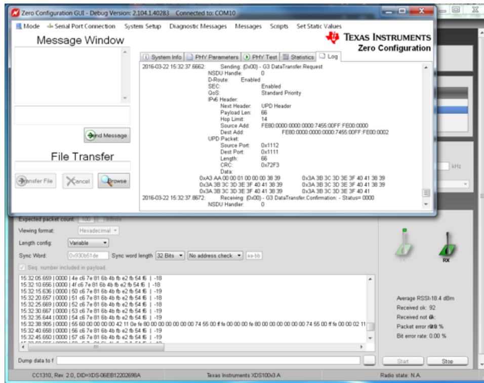
图 28. PLC-to-RF Repeater
