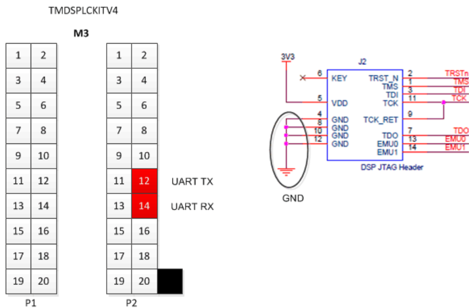
图 8. UART Pins on TMDSPCKITV4
