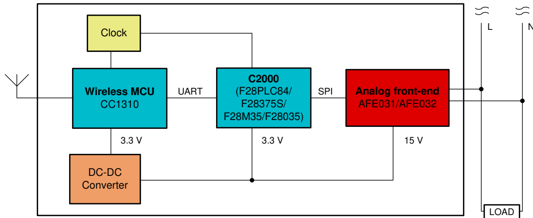
图 2. Block Diagram
