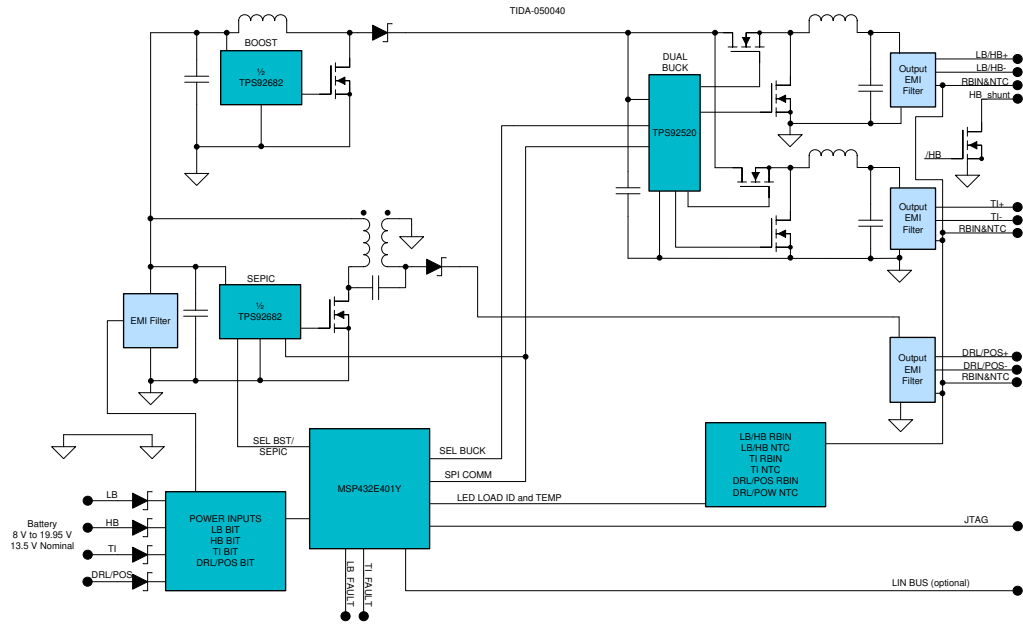
图 2-1. TIDA050040 Block Diagram
