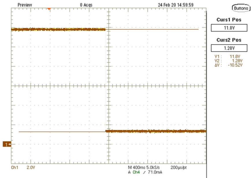
图 3-16. Turn Indicator Fault Output
