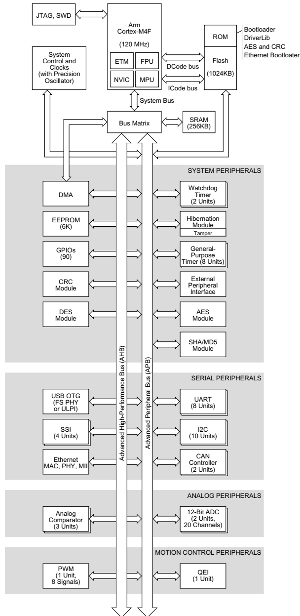
图 2-4. MSP432E401Y Functional Block Diagram
