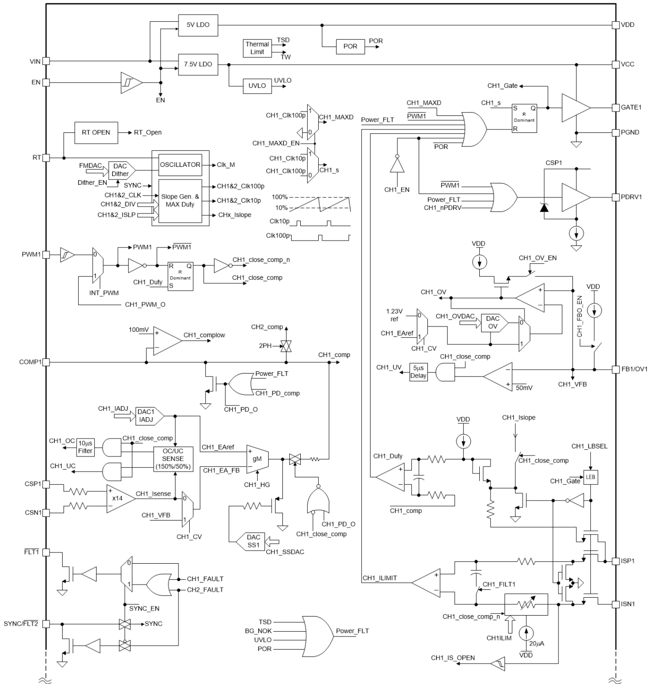
图 2-2. TPS92682-Q1 Functional Block Diagram
