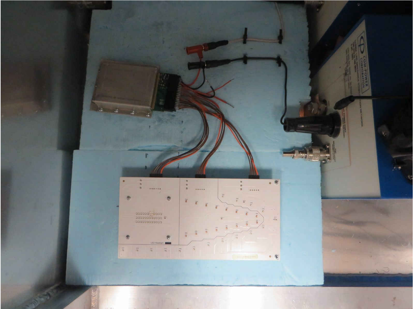
图 3-2. CISPR 25 Class 5 test setup
