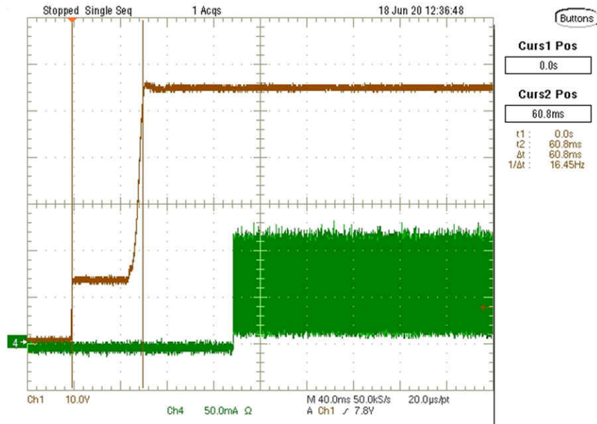
图 3-5. Boost Turn on Delay
