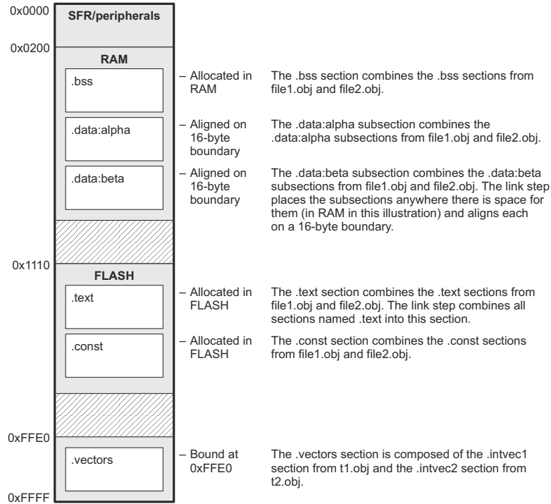
图 8-2. SECTIONS 指令定义的段的放置
