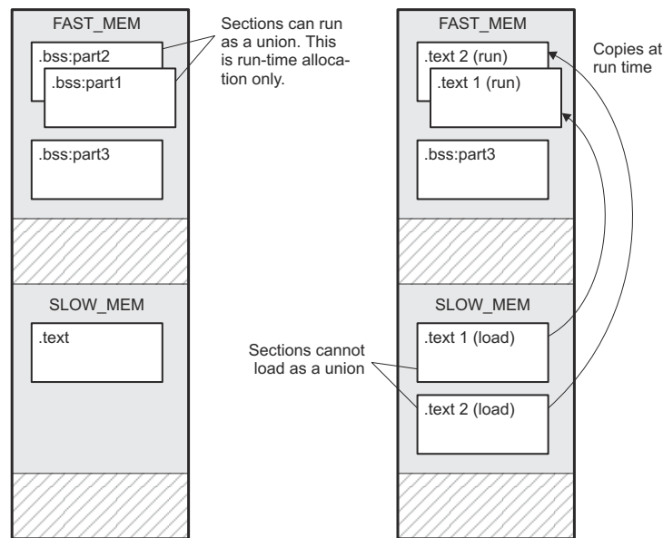
图 8-4. 存储器分配如 UNION 语句和 分离 UNION 段的加载地址所示
