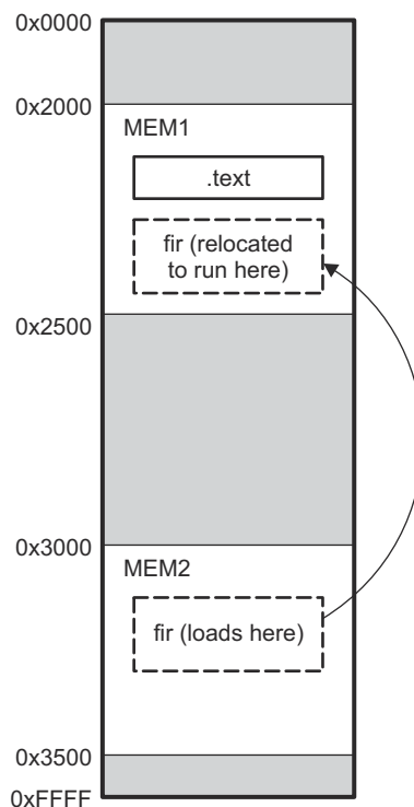
图 8-3. 在运行时将一个函数从慢速存储器移动到快速存储器 的运行时执行
