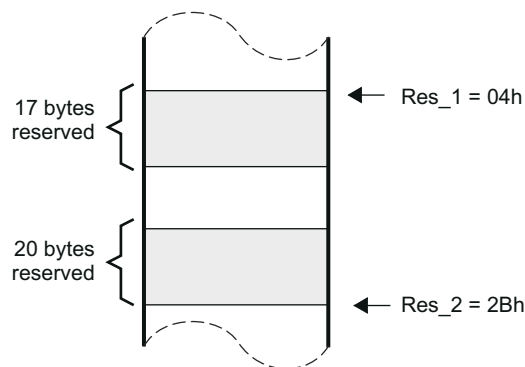
图 5-4. .space 和 .bes 指令
