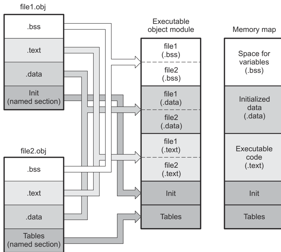
图 2-4. 组合输入段以构成可执行对象模块
