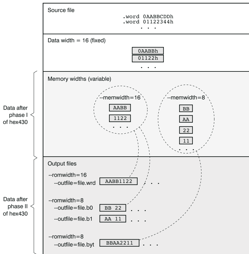
图 12-4. 数据、存储器和 ROM 宽度
