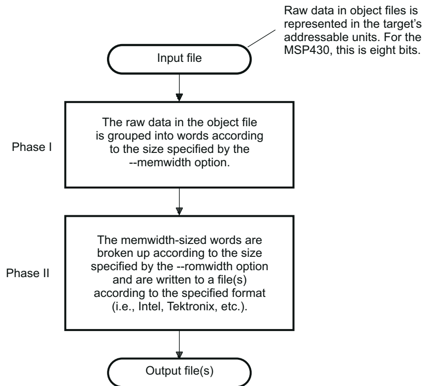
图 12-2. 十六进制转换实用程序处理流程
