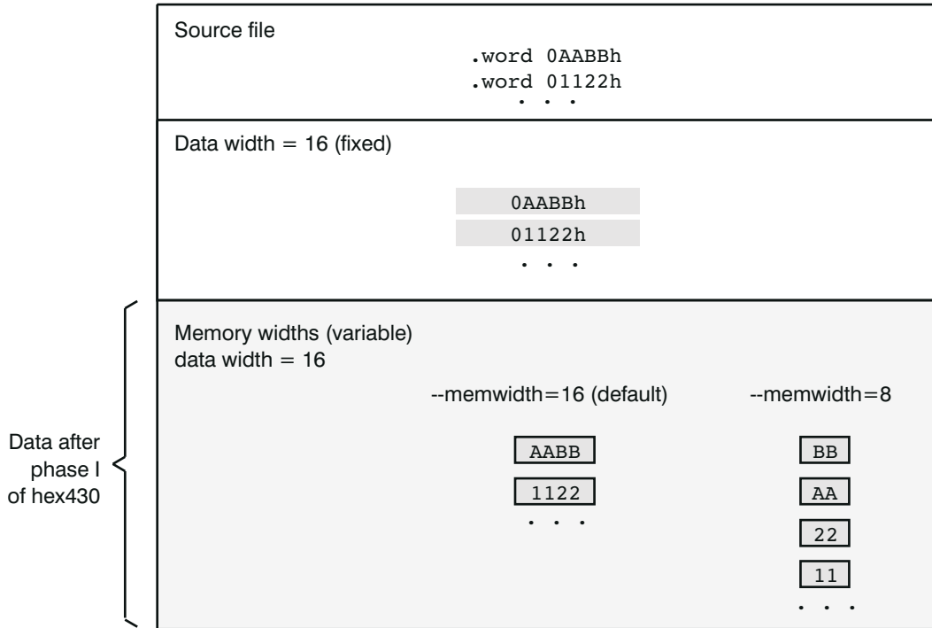
图 12-3. 目标文件数据与存储器宽度
