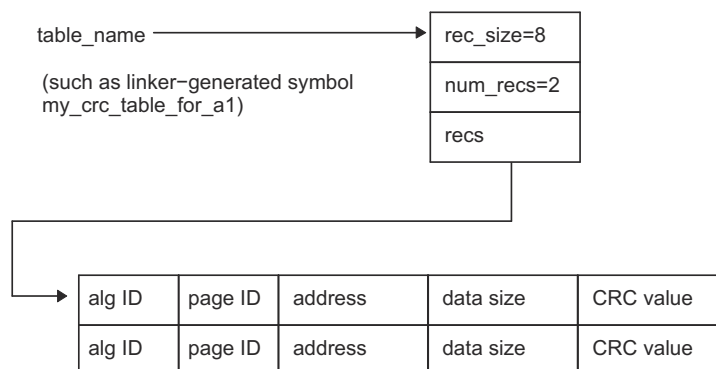
图 8-7. CRC_TABLE 概念模型
