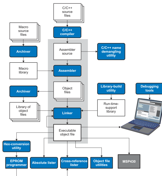
图 8-1. MSP430 软件开发流程中的链接器
