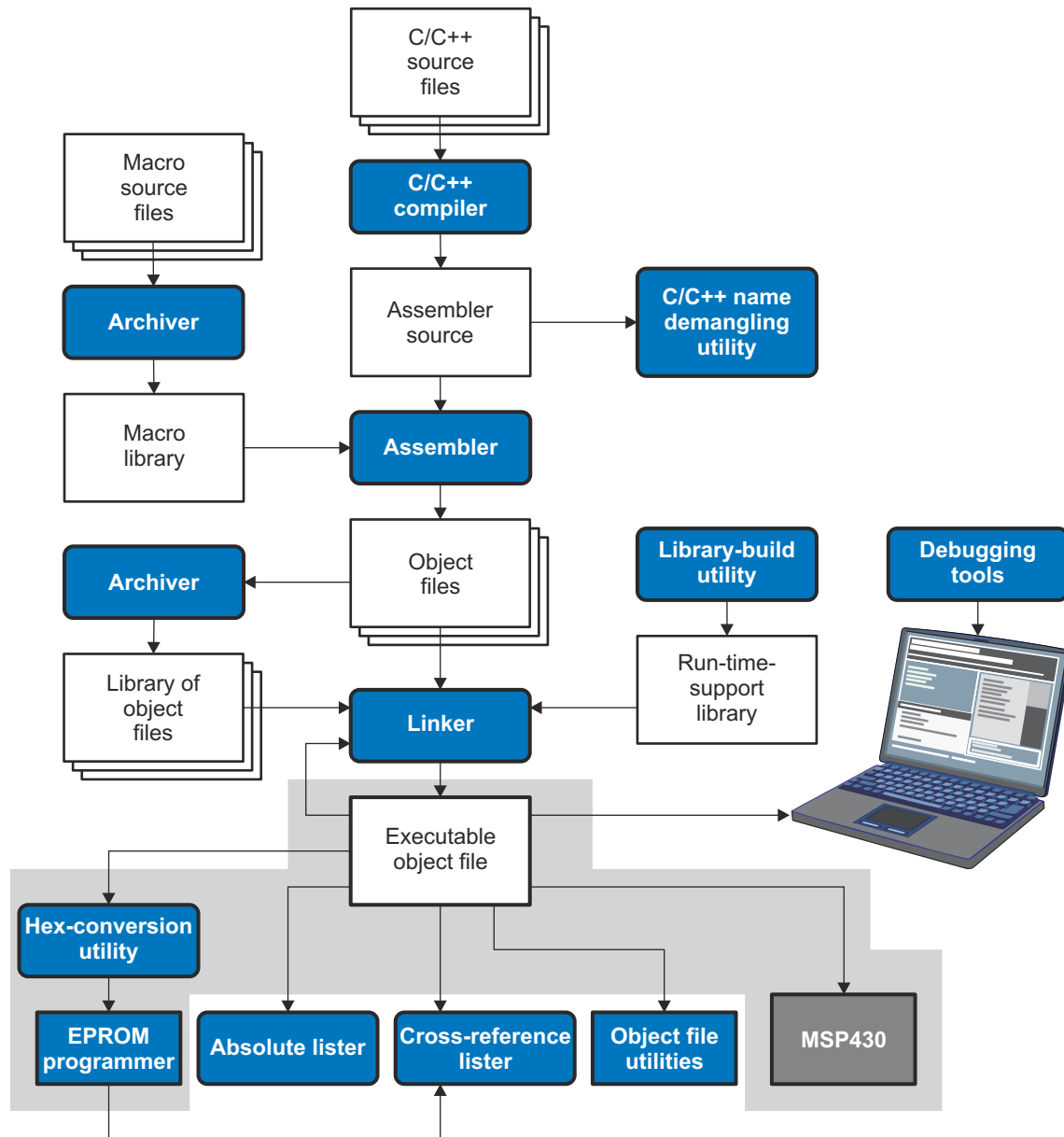
图 12-1. MSP430 软件开发流程中的十六进制转换实用程序
