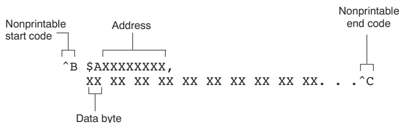
图 12-6. ASCII 十六进制对象格式
