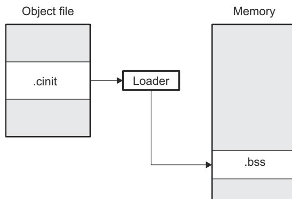
图 3-3. 加载时初始化
