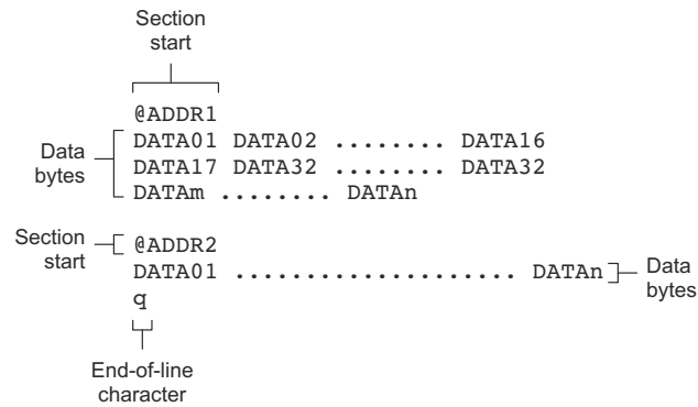
图 12-11. TI-TXT 目标格式
