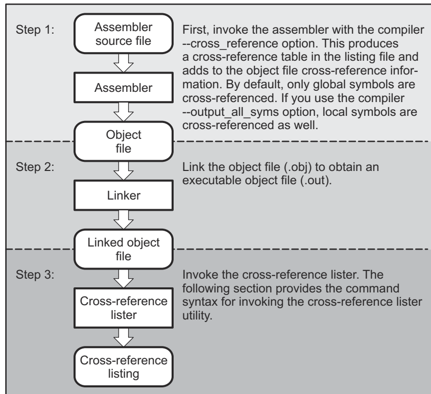
图 10-1. 交叉参考列表器开发流程
