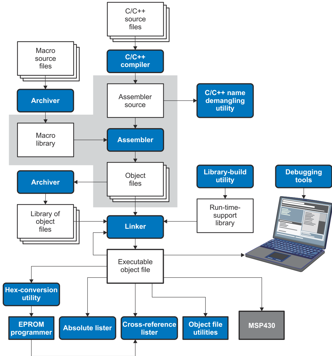
图 4-1. MSP430 软件开发流程中的汇编器
