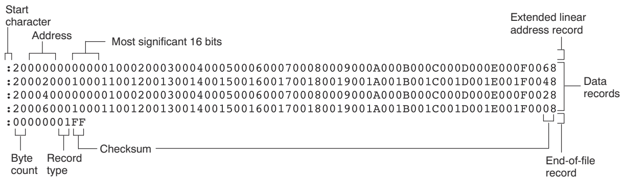
图 12-7. Intel 十六进制目标格式
