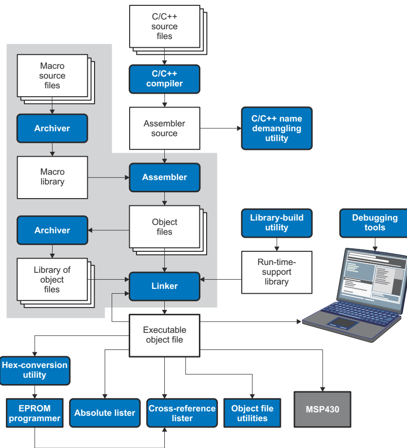
图 7-1. MSP430 软件开发流程中的归档器
