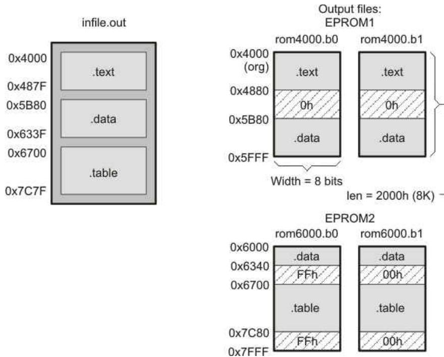
图 12-5. infile.out 文件分区成四个输出文件
