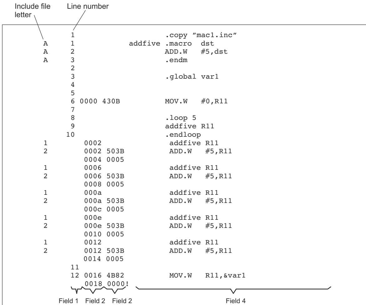
图 4-2. 汇编列表示例
