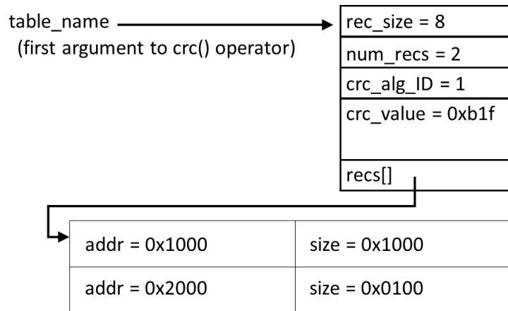
图 8-8. 存储器范围的 CRC 存储格式
