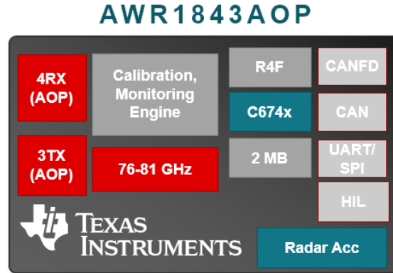
图 2-3. AWR1843AOP Block Diagram
