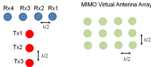
图 2-4. AWR1843AOP Antenna Virtual Array
