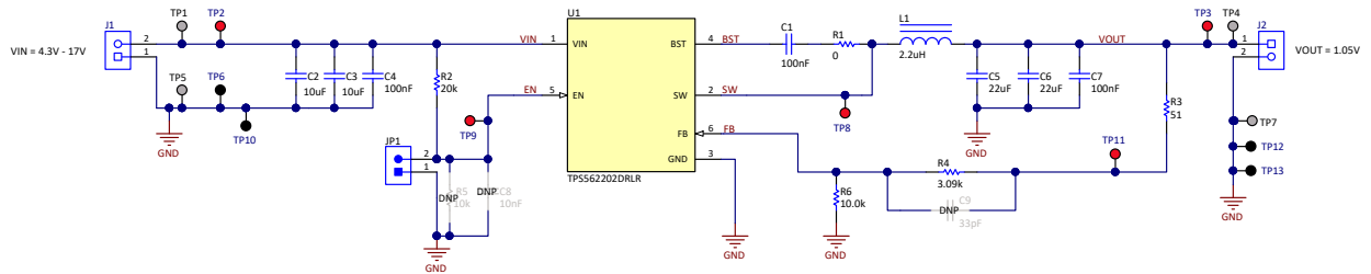
图 6-1. TPS562202EVM 原理图
