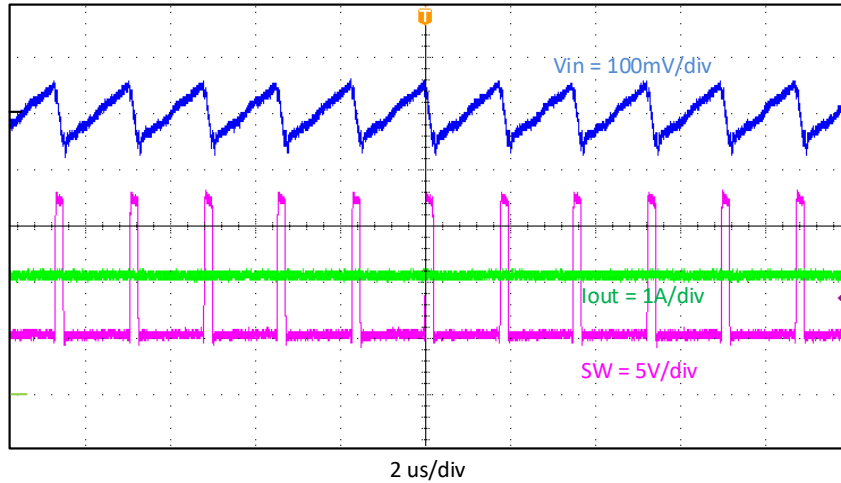
图 4-8. 输入电压纹波, I_{OUT} = 2A
