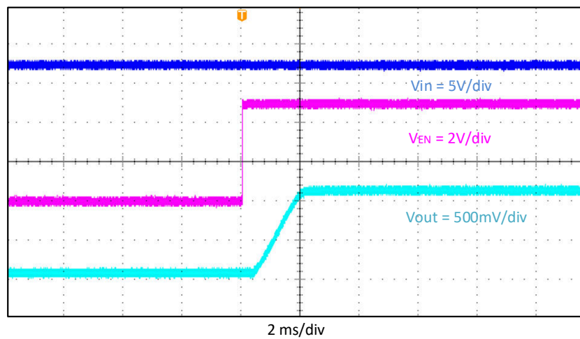
图 4-3. 相对于 EN、 I_{OUT} = 2A 的启动
