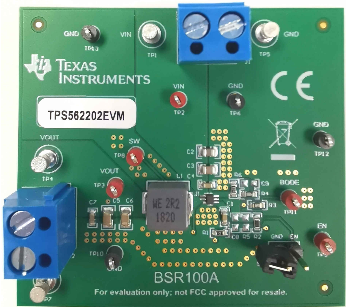
图 5-4. TPS562202EVM 电路板顶视图
