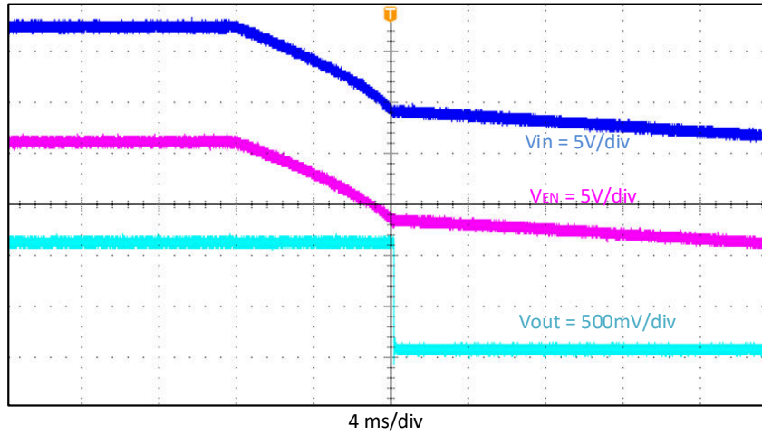
图 4-4. 相对于 V_{IN} 、 I_{OUT} = 2A 的关断
