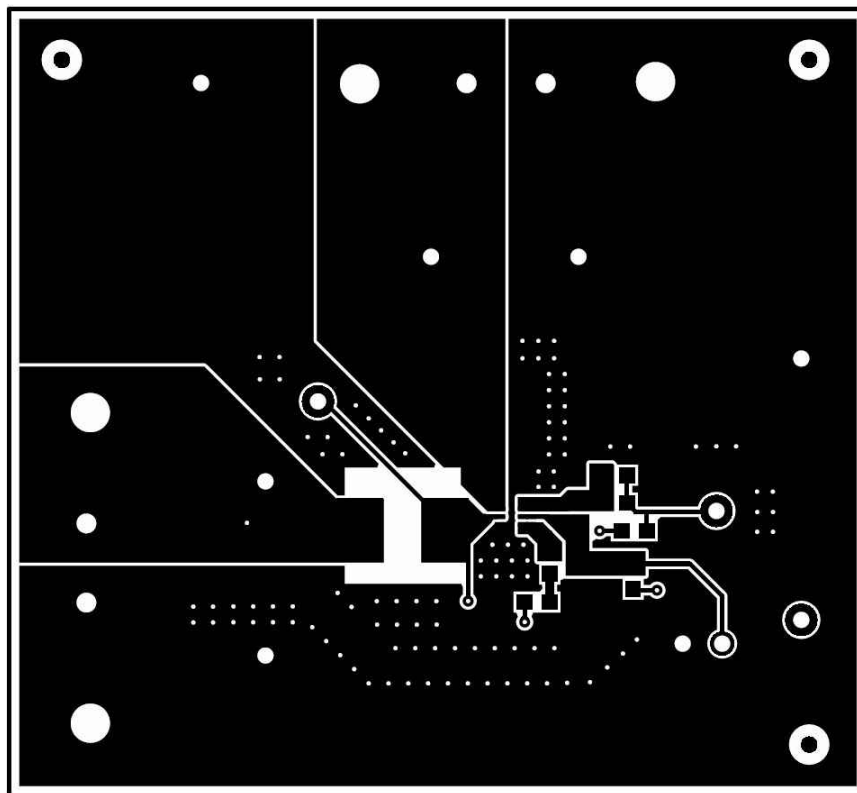
图 5-2. TPS562202EVM 顶层
