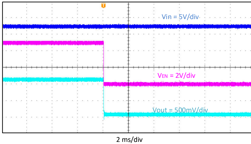
图 4-5. 相对于 EN、 I_{OUT} = 2A 的关断
