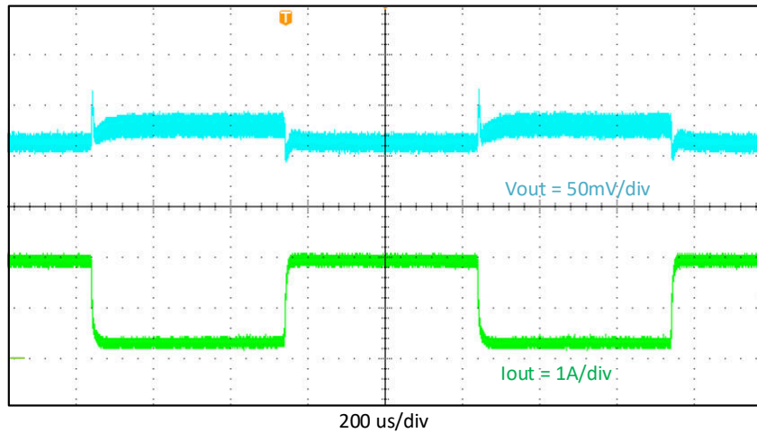
图 4-9. 负载瞬态响应, 10% 至 90% (0.2A - 1.8A) 负载阶跃
