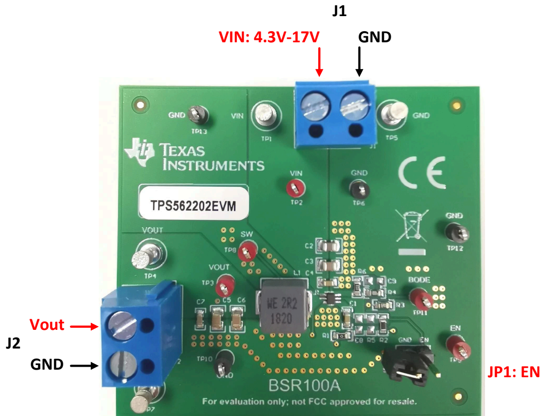
图 4-1. TPS562202EVM 连接器和跳线布置
