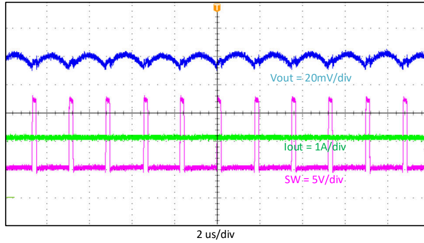
图 4-6. 输出电压纹波, I_{OUT} = 2A
