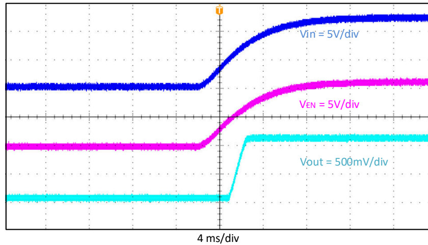
图 4-2. 相对于 V_{IN} 、 I_{OUT} = 2A 的启动
