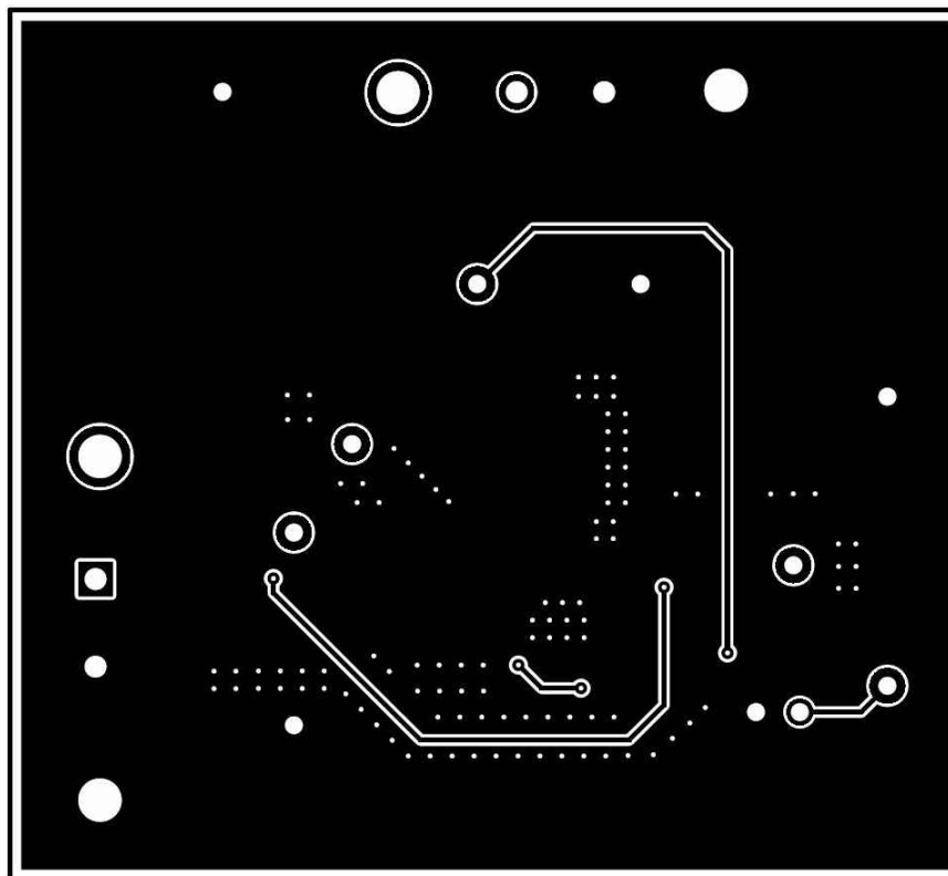
图 5-3. TPS562202EVM 底层
