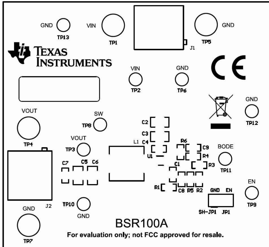
图 5-1. TPS562202EVM 顶层装配图
