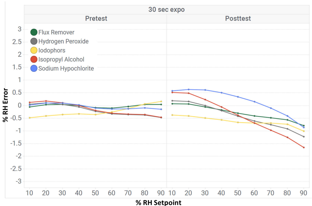
图 2-1. 短时间暴露：一次性暴露
