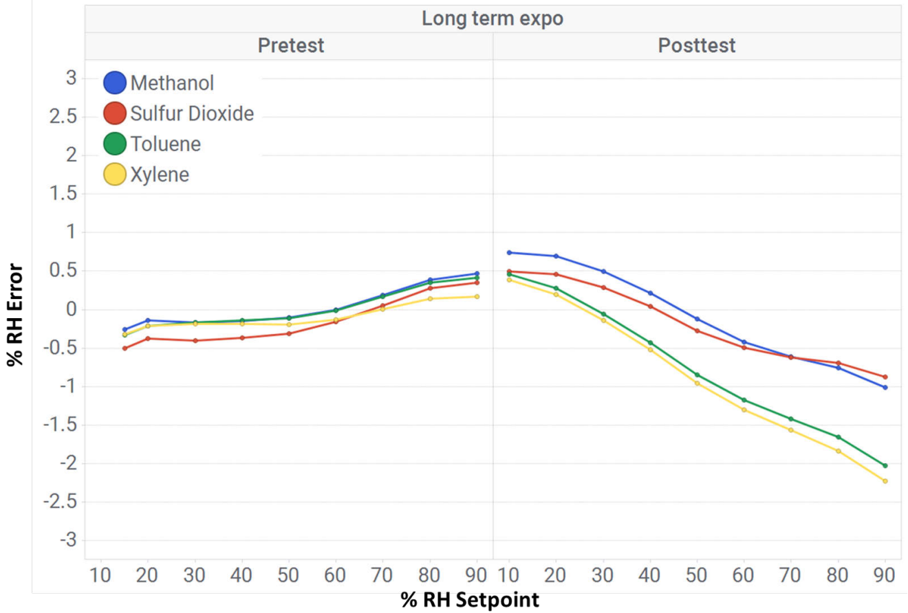
图 2-4. 长时间暴露结果
