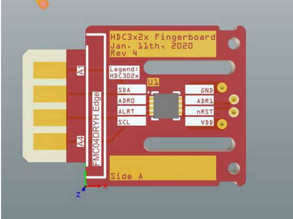
图 3-7. HDC3020 指板
