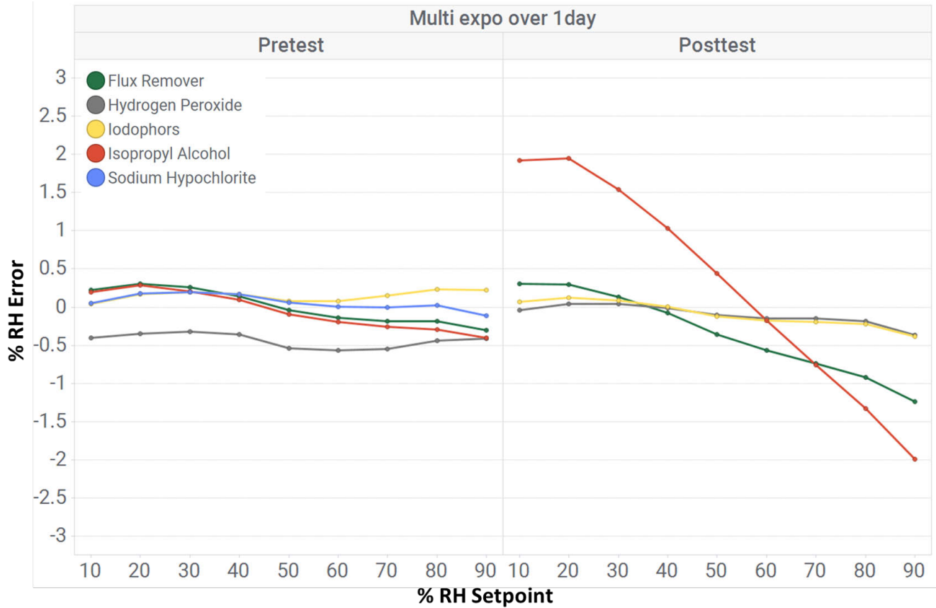
图 2-2. 短时间暴露：多次暴露
