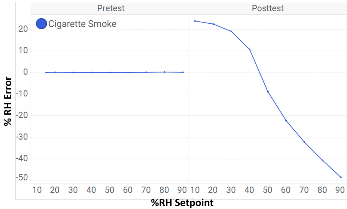
图 2-5. 长时间暴露于香烟烟雾中
