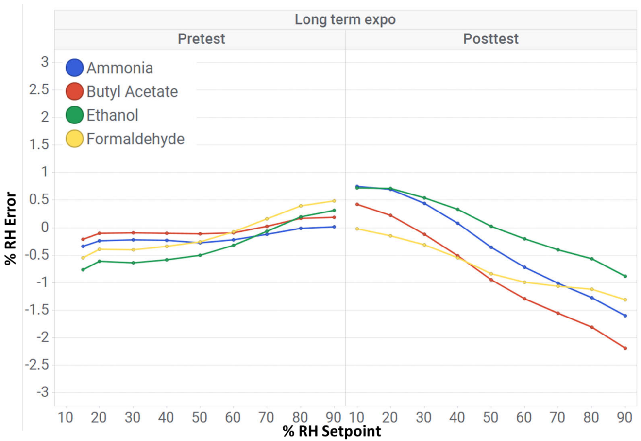
图 2-3. 长时间暴露结果
