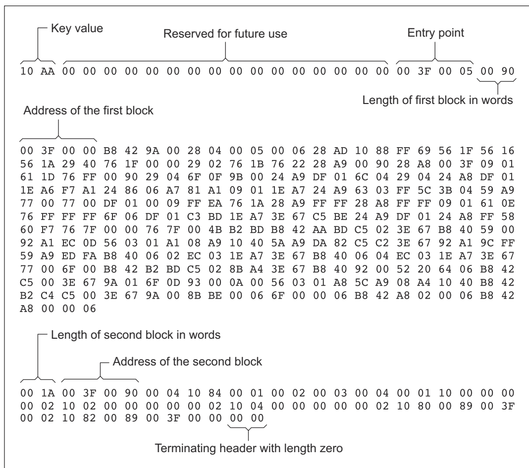
图 12-7. C28x 16 位并行引导 GP I/O 的示例十六进制转换器输出文件
