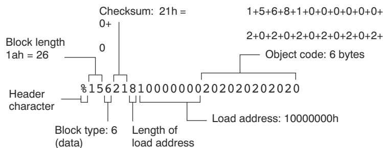
图 12-12. 扩展的 Tektronix 目标格式
