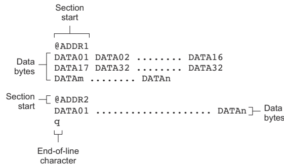
图 12-14. TI-TXT 目标格式
