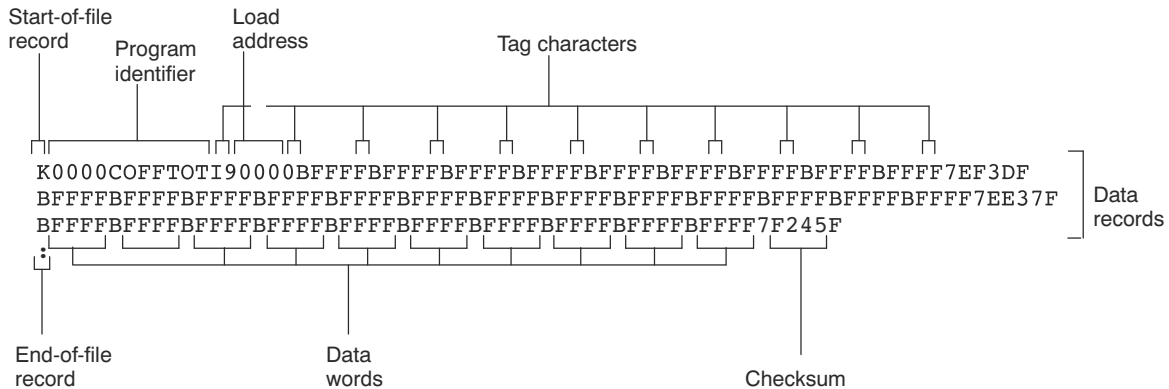
图 12-13. TI-Tagged 目标格式
