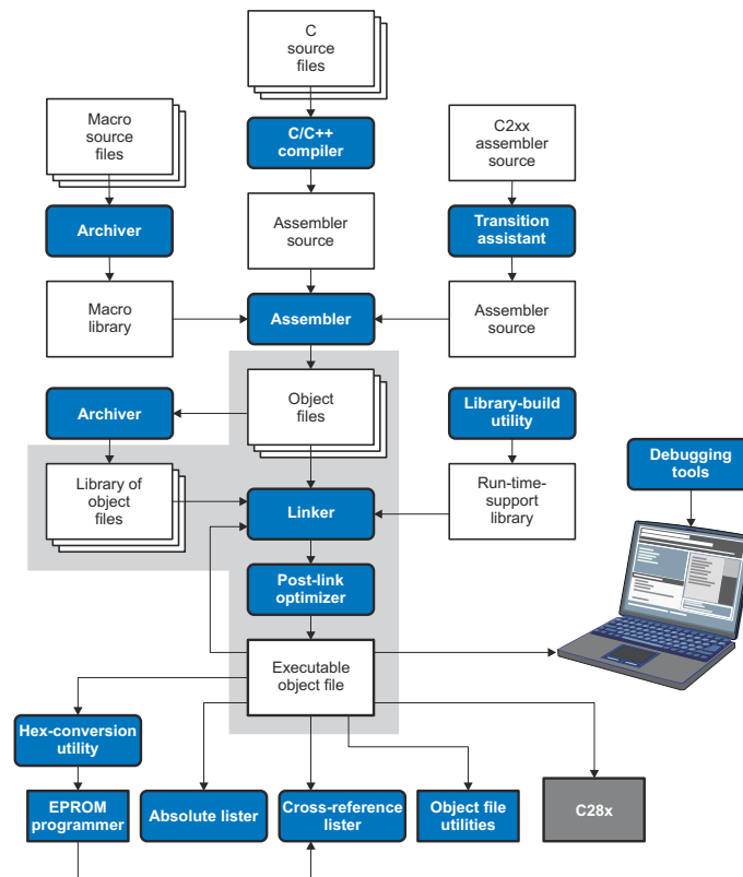
图 8-1. TMS320C28x 软件开发流程中的链接器
