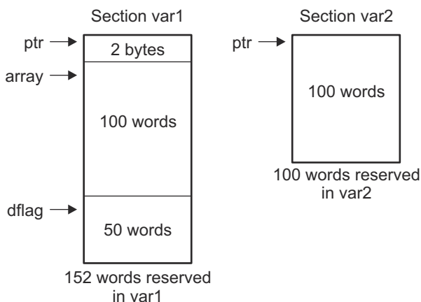
图 5-7. .usect 指令
