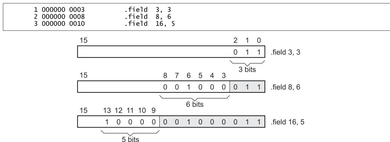
图 5-1. .field 指令
