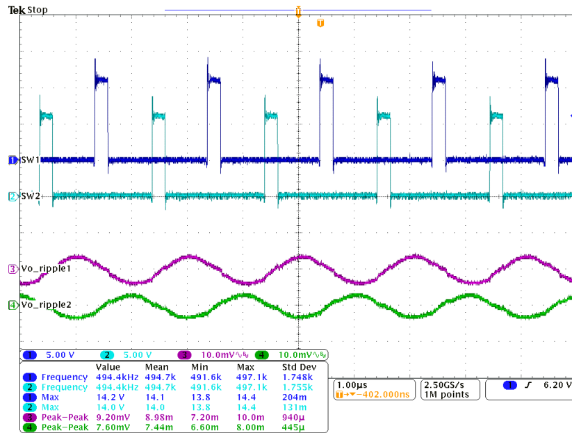
图 7-5. 在 1.2V 输出下且 V_{IN} 为 12、输出为 0A 时的输出纹波和开关节点
