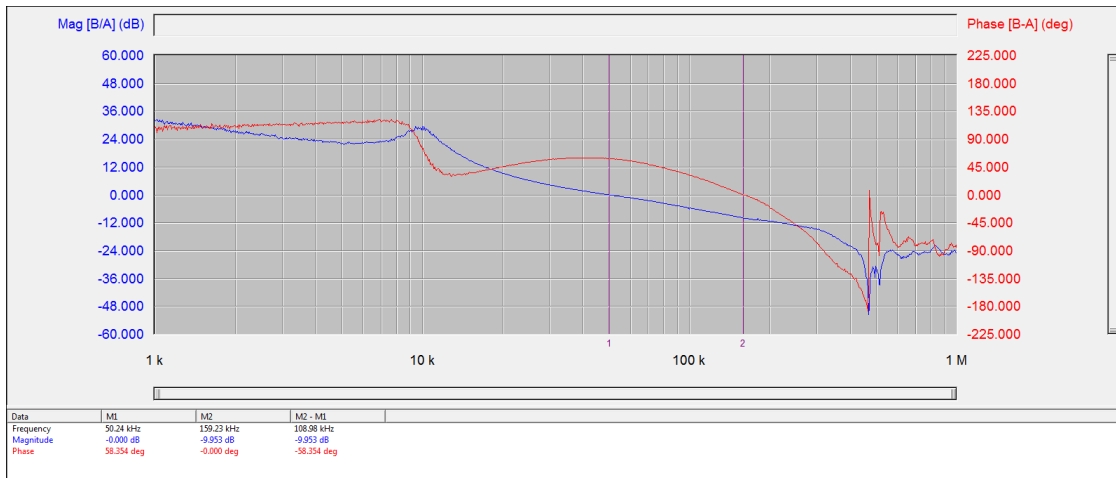
图 7-13. 在 1.2V 输出下且 V_{IN} 为 12、输出为 70A 时的波特图
