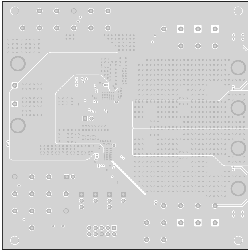
图 8-5. TPS546C23EVM2-746 EVM 内层 1 (顶视图)
