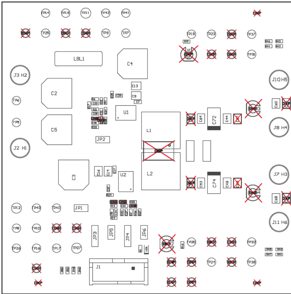
图 8-2. TPS546C23EVM2-746 EVM 顶层装配图 (顶视图)
