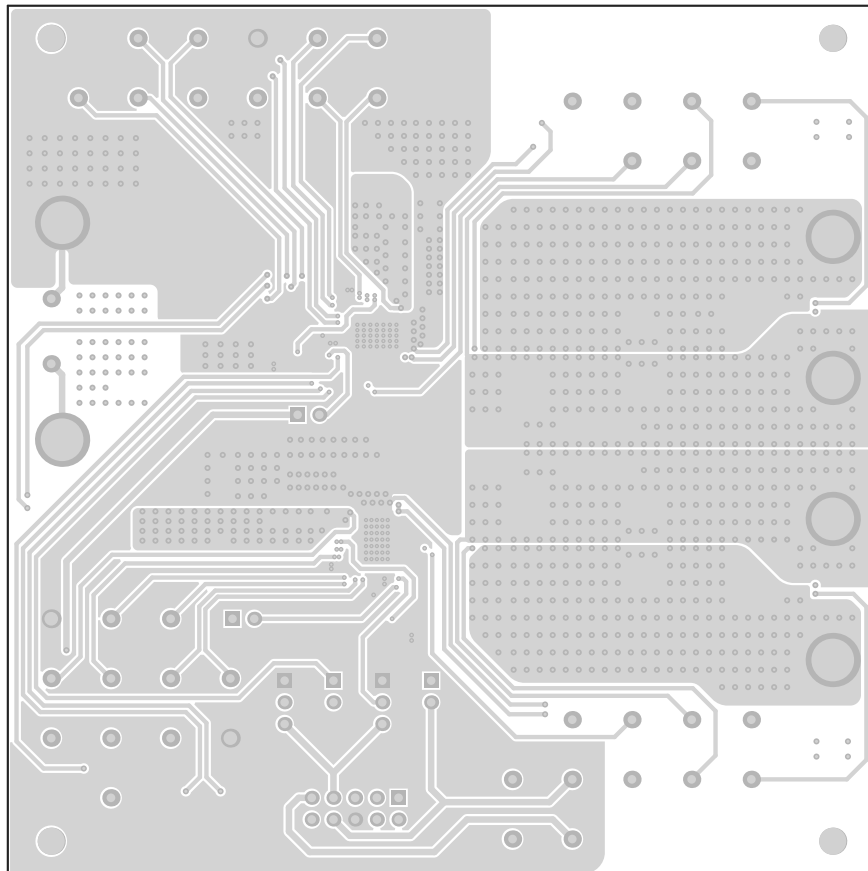
图 8-6. TPS546C23EVM2-746 EVM 内层 2 ( 顶视图 )
