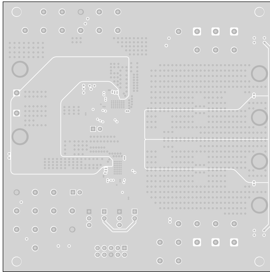
图 8-7. TPS546C23EVM2-746 EVM 内层 3 ( 顶视图 )
