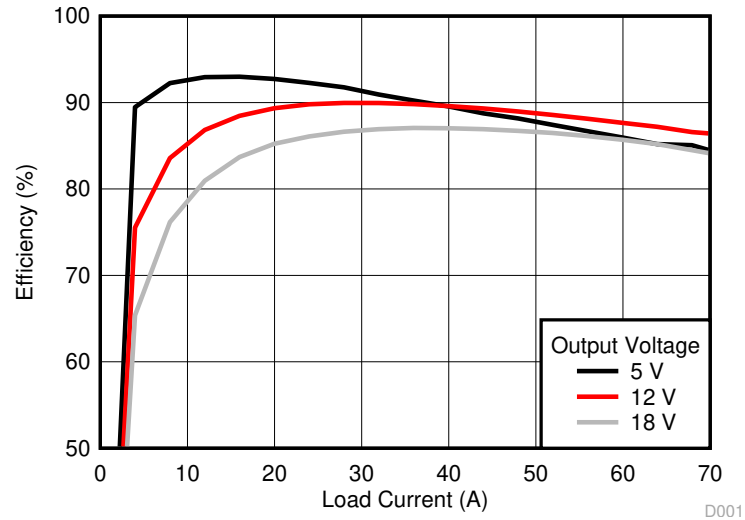
图 7-1. 在输出下的效率与线路/负载间的关系
