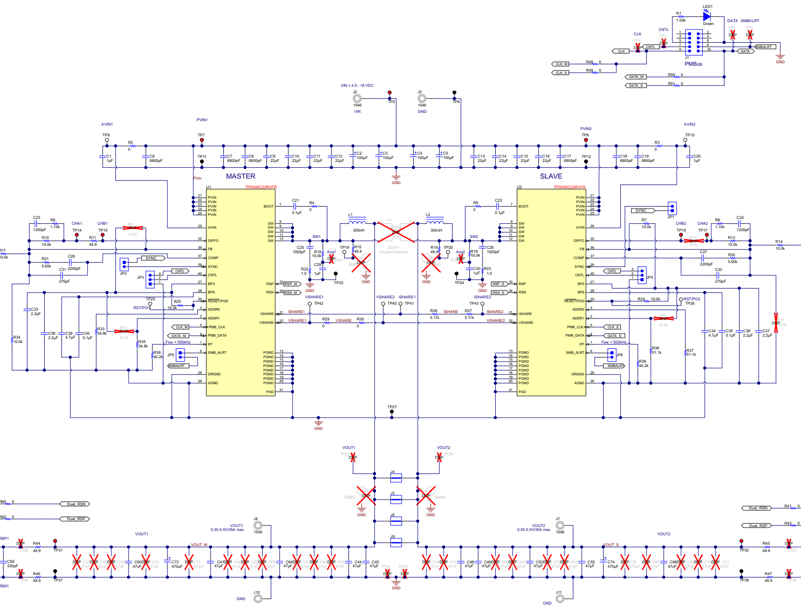
图 3-1. TPS546C23EVM2-746 原理图
