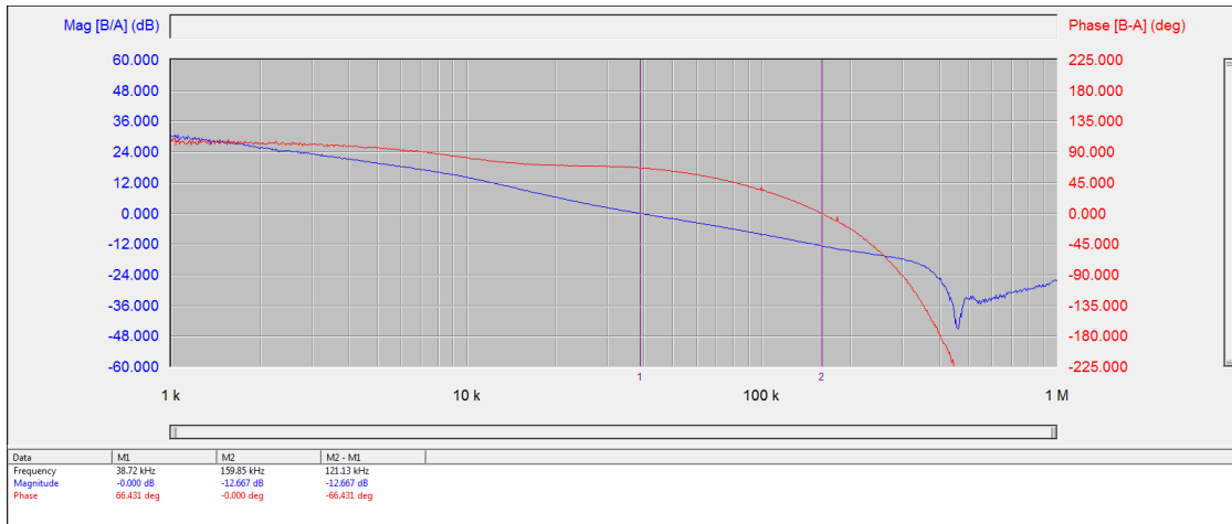
图 7-12. 在 1.2V 输出下且 V_{IN} 为 12、输出为 0A 时的波特图
