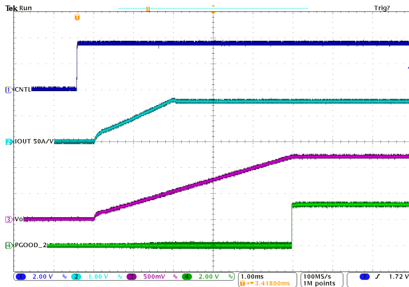
图 7-7. 通过控制实现启动，在 1.2V 输出下且 V_{IN} 为 12、输出为 0A ( 将 TON_RISE 修改为 5ms )
