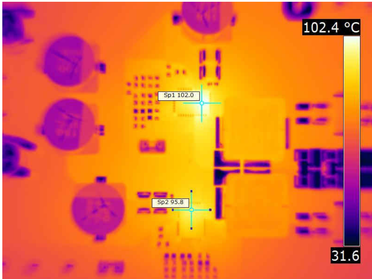
图 7-14. 热像图
