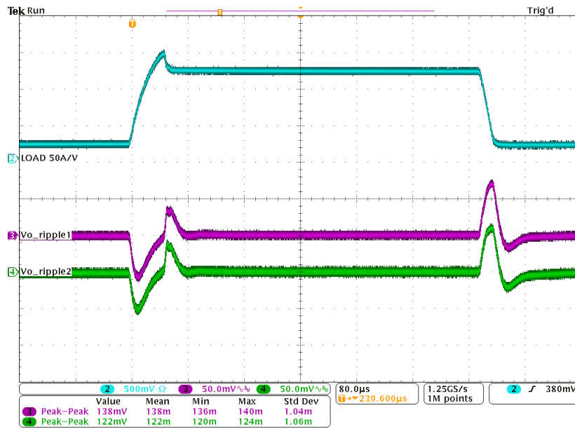
图 7-4. 在 1.2V 输出下且 V_{IN} 为 12 时的瞬态响应, 瞬态电流为 10A 至 60A, 0.2A/ \mu s
