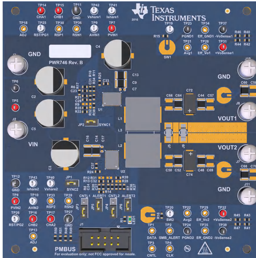
图 8-1. TPS546C23EVM2-746 EVM 3D (顶视图)
