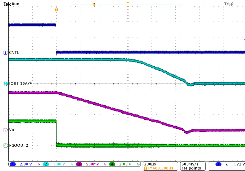
图 7-9. 通过控制实现软停止, 在 1.2V 输出下且 V_{IN} 为 12、输出为 0A (将 TON_RISE 修改为 5ms)
