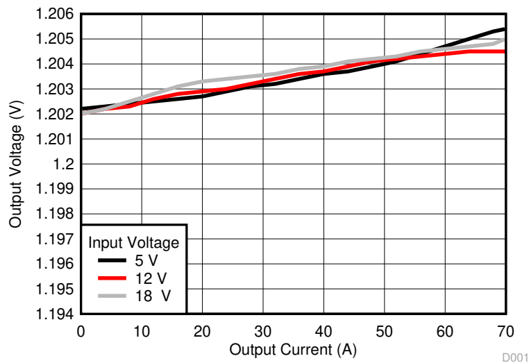
图 7-2. 在输出下的负载调节
