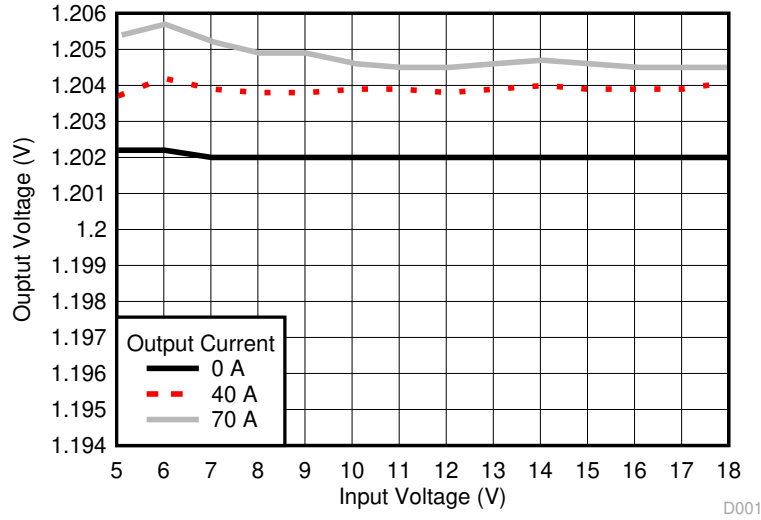
图 7-3. 在 1.2V 输出下的线路调节 (不同电路板)
