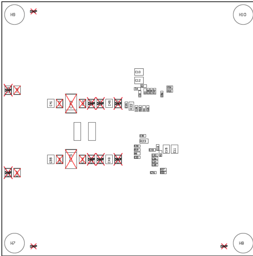
图 8-3. TPS546C23EVM2-746 EVM 底层装配图 (底视图)
