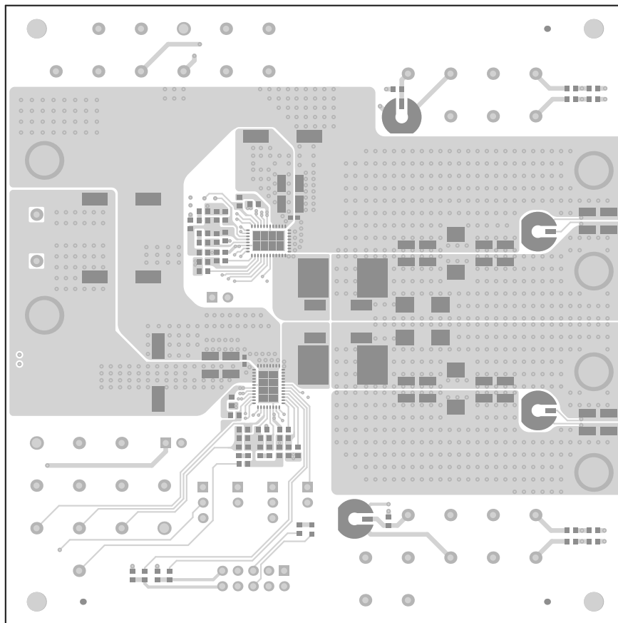
图 8-4. TPS546C23EVM2-746 EVM 顶层铜 ( 顶视图 )
