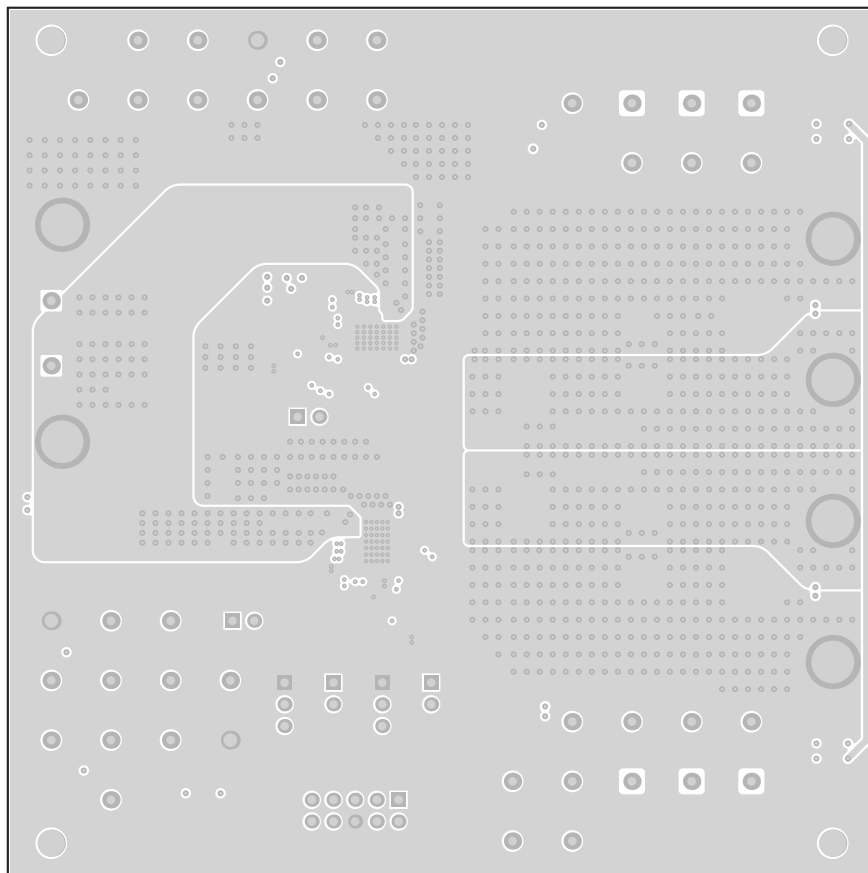
图 8-8. TPS546C23EVM2-746 EVM 内层 4 (顶视图)
