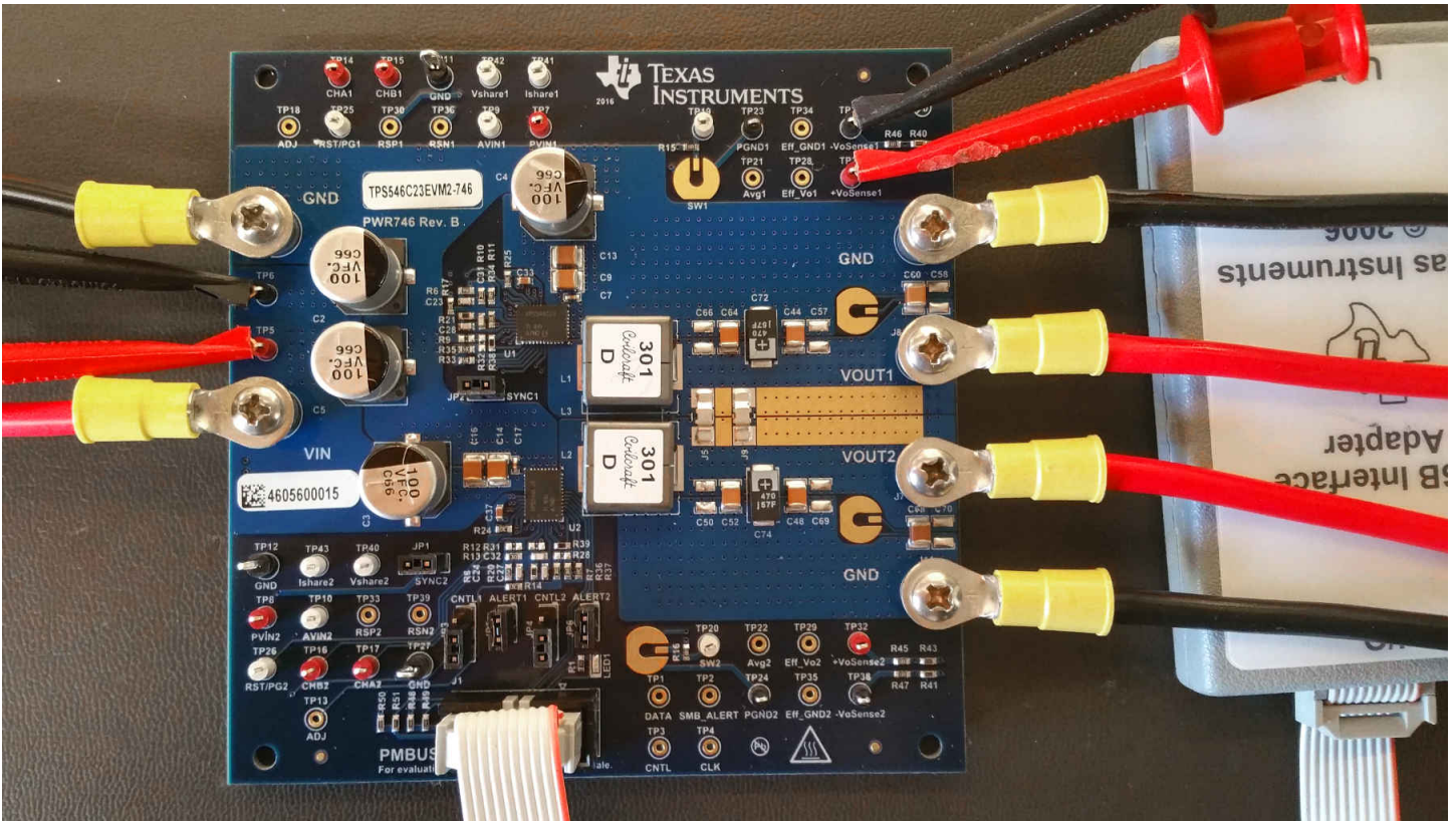
图 4-1. TPS546C23EVM2-746 建议使用的 EVM 测试设置
