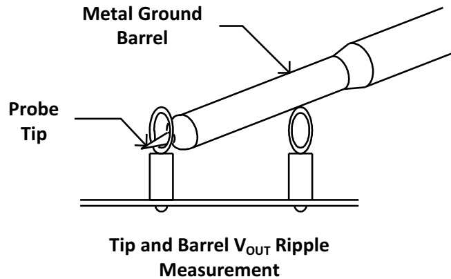
图 4-2. “尖头与桶”测量
