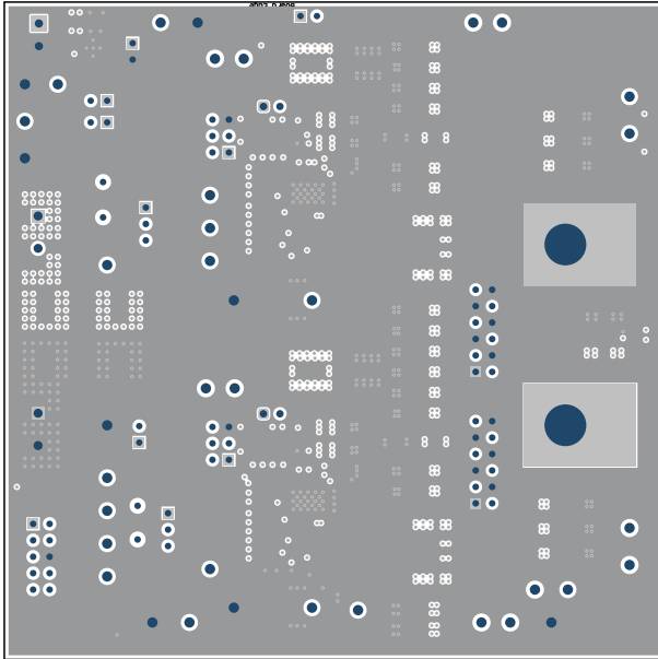
图 8-11. TPS546B24AEVM-2PH 内层 6 (顶视图)
