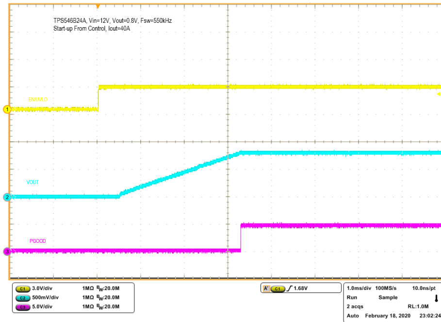
图 7-12. 通过控制器启动，40A 负载
