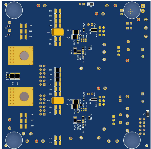
图 8-2. TPS546B24AEVM-2PH 3D (底视图)
