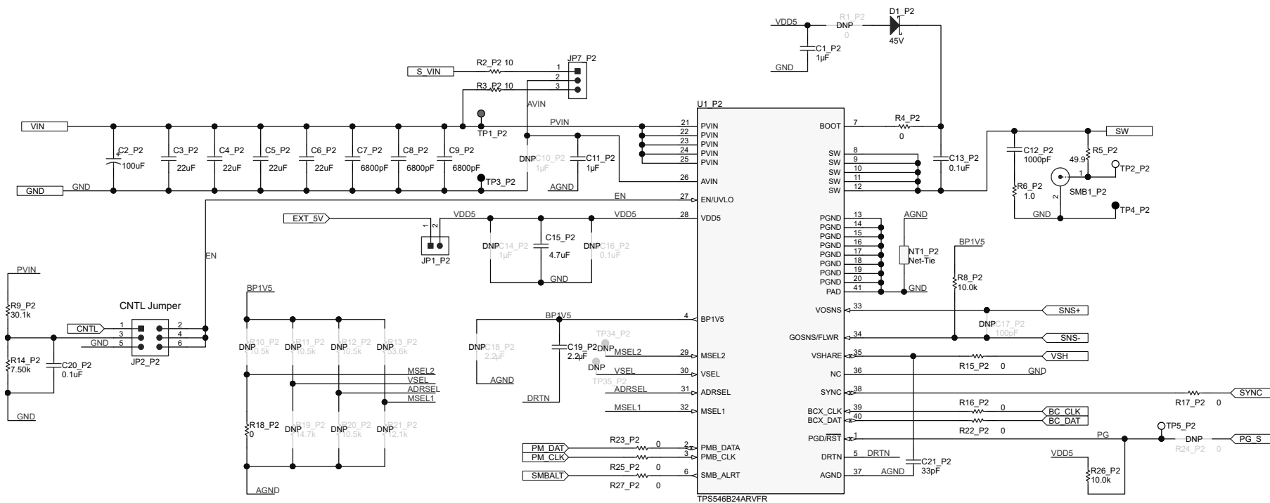
图 3-3. TPS546B24AEVM-2PH 原理图第 3 页 ( U1_P2 环路跟随器 )
