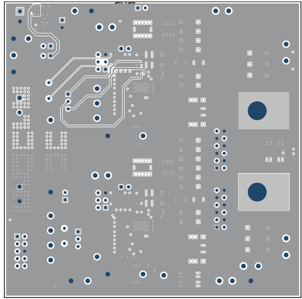
图 8-6. TPS546B24AEVM-2PH 内层 1 (顶视图)
