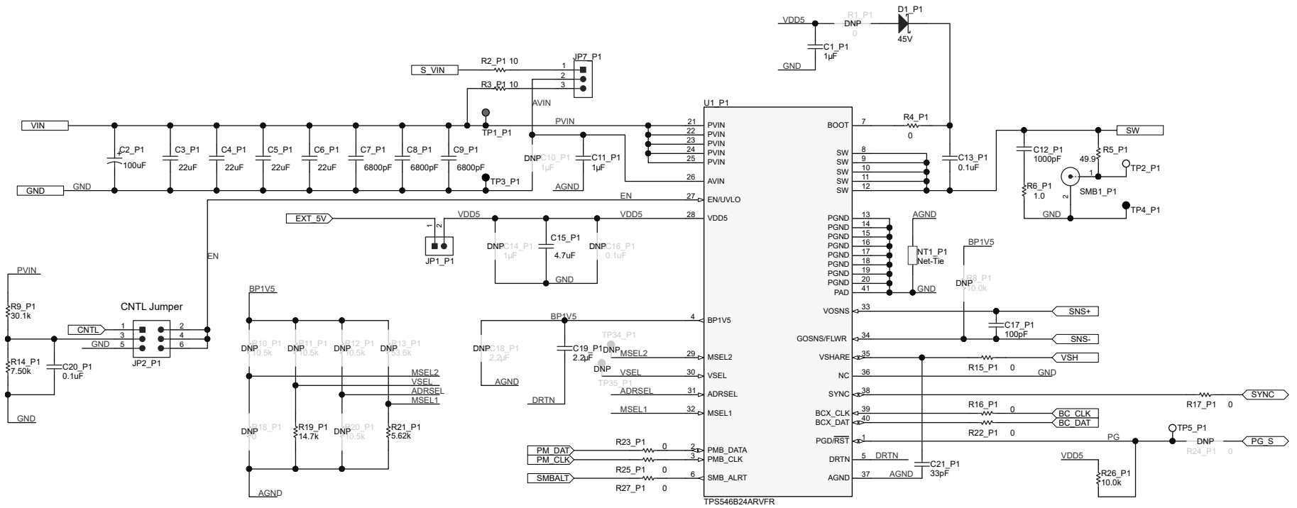
图 3-2. TPS546B24AEVM-2PH 原理图第 2 页 ( U1_P1 环路控制器 )
