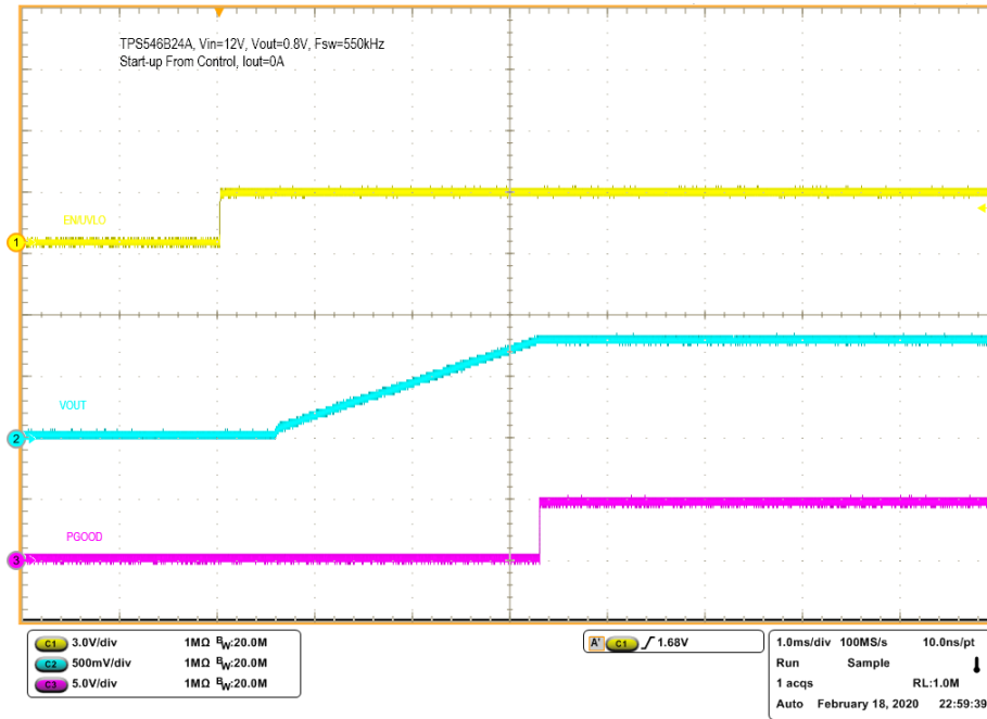
图 7-11. 通过控制器启动，0A 负载
