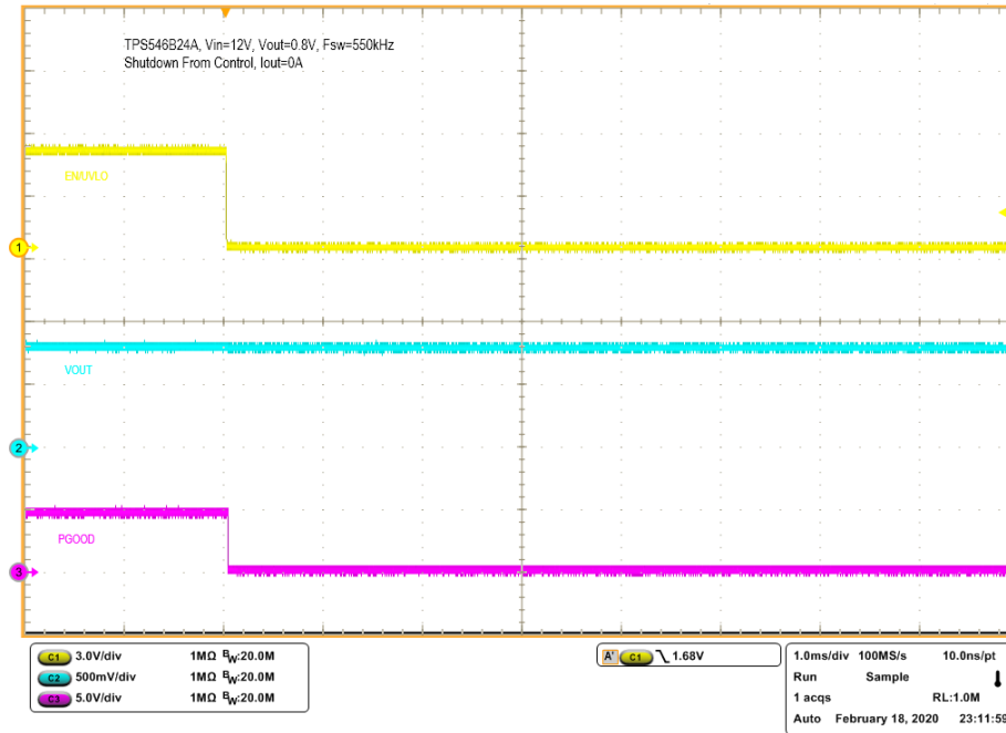
图 7-13. 通过控制器关断，0A 负载
