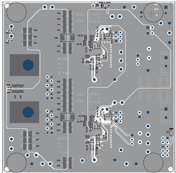
图 8-4. TPS546B24AEVM-2PH 底面元件视图 (底视图)
