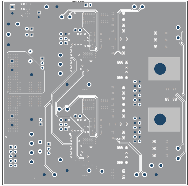
图 8-10. TPS546B24AEVM-2PH 内层 5 (顶视图)
