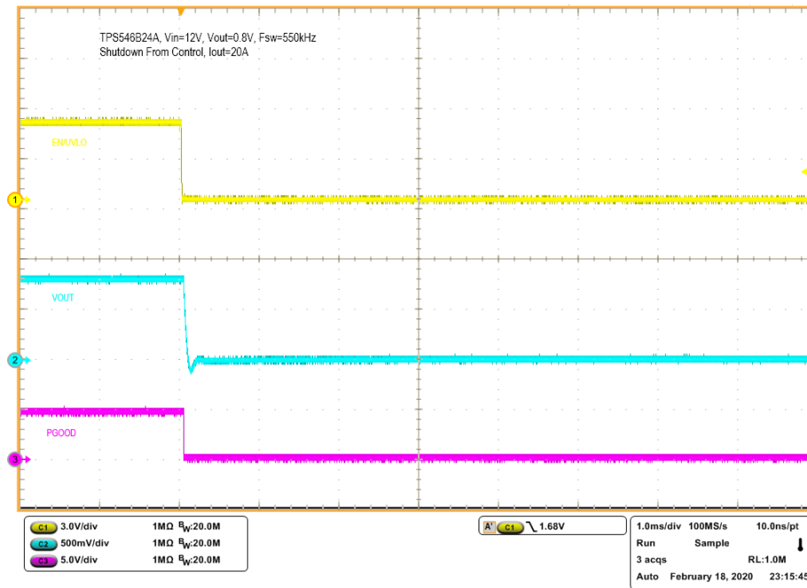
图 7-14. 通过控制器关断，20A CC 负载
