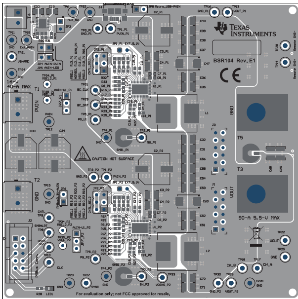
图 8-3. TPS546B24AEVM-2PH 顶面元件视图 (顶视图)
