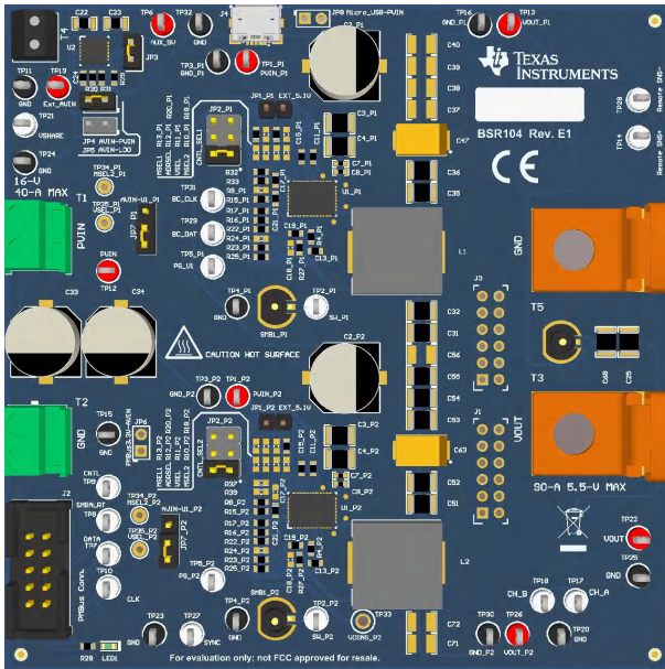
图 8-1. TPS546B24AEVM-2PH 3D (顶视图)
