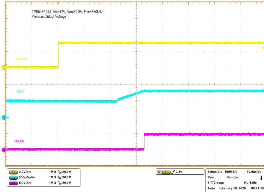
图 7-15. 通过具有预偏置输出的控制器进行启动
