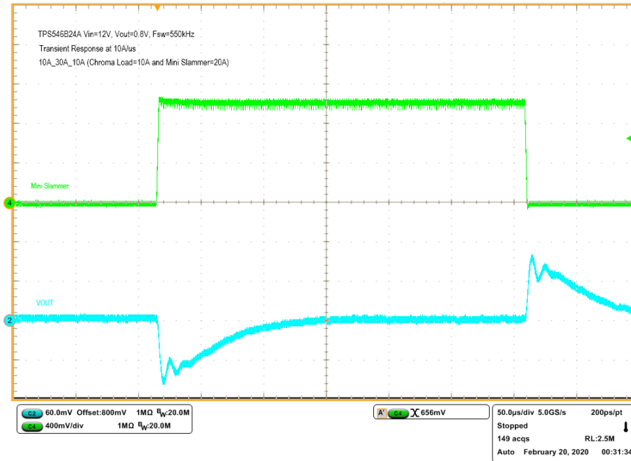
图 7-5. 瞬态响应
