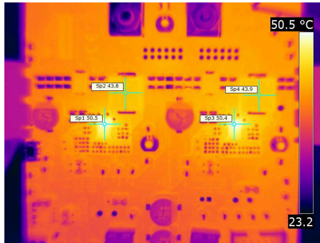
图 7-17. 热像图
