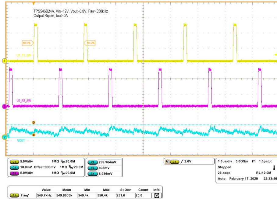
图 7-7. 0A 负载时的输出纹波
