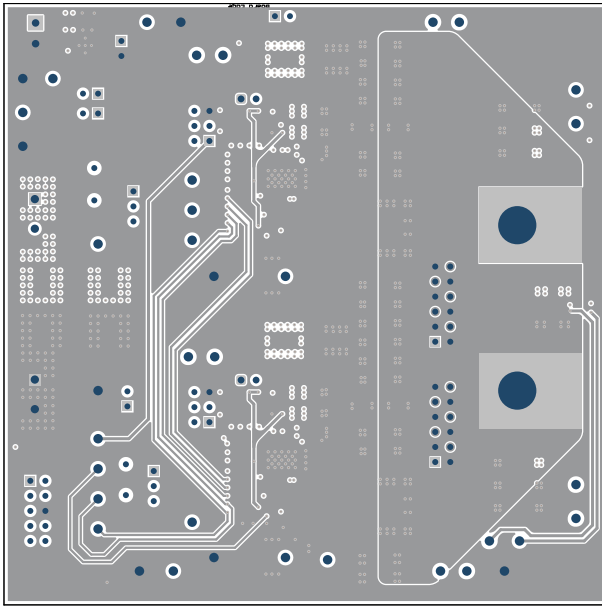
图 8-9. TPS546B24AEVM-2PH 内层 4 (顶视图)
