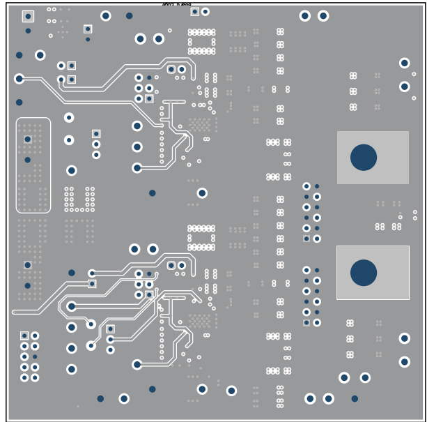
图 8-8. TPS546B24AEVM-2PH 内层 3 (顶视图)
