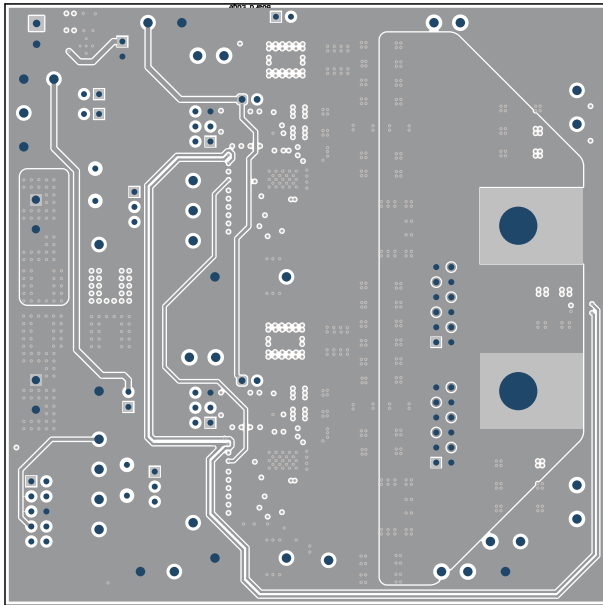
图 8-7. TPS546B24AEVM-2PH 内层 2 (顶视图)
