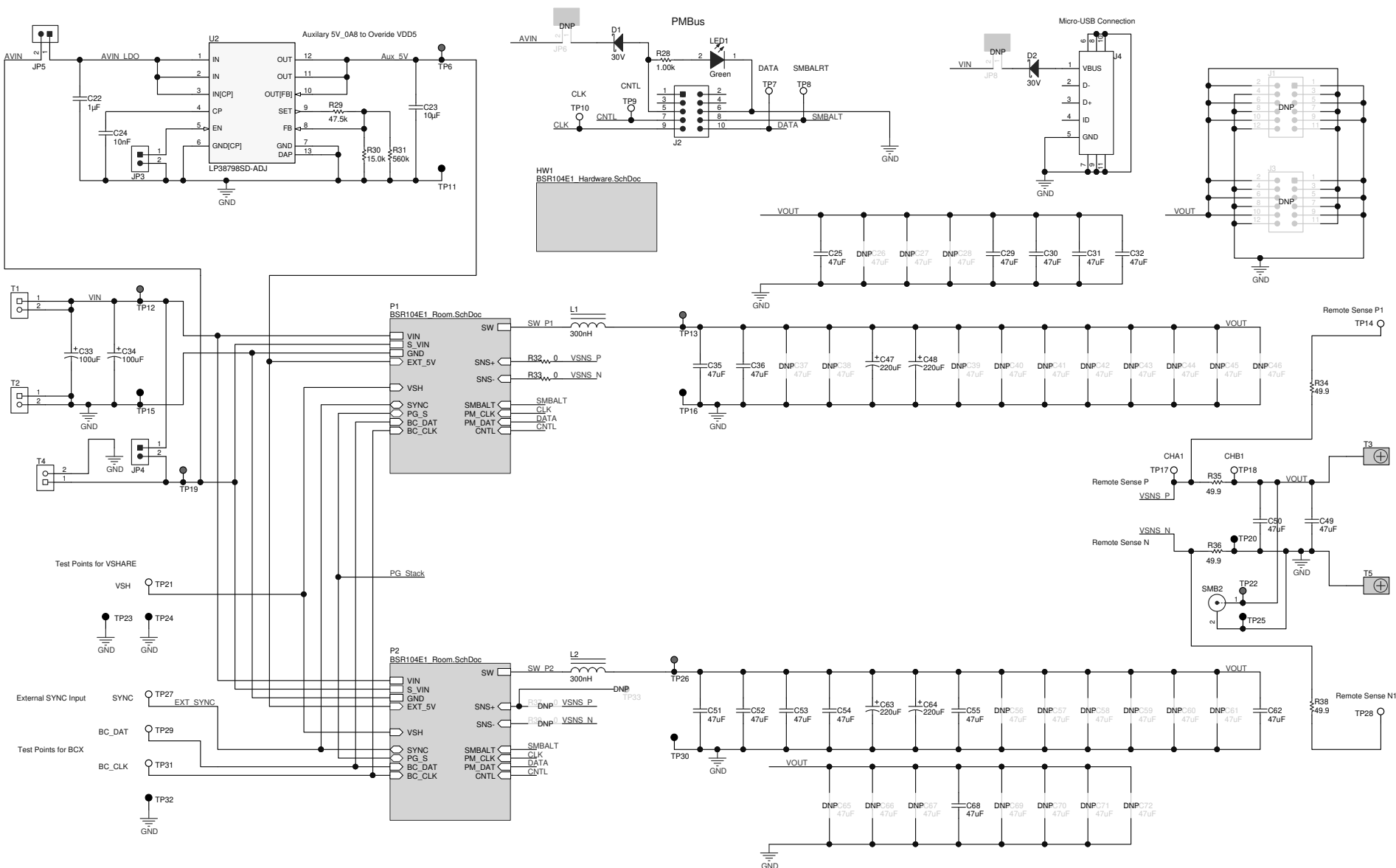
图 3-1. TPS546B24AEVM-2PH 原理图第 1 页
