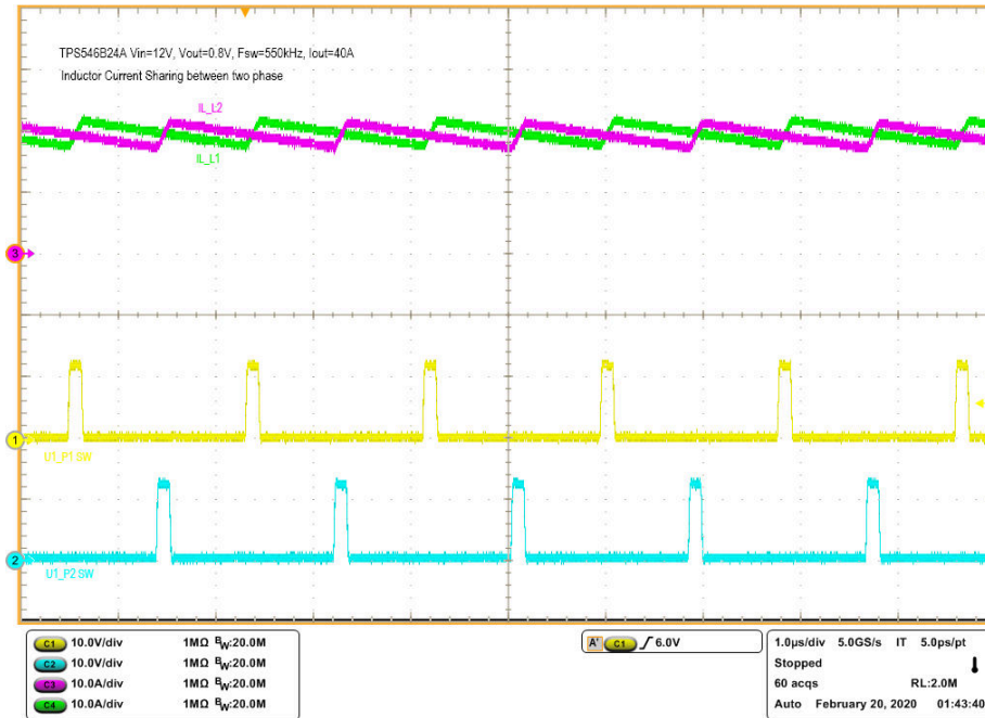
图 7-16. 电感电流和开关节点波形，40A 负载
