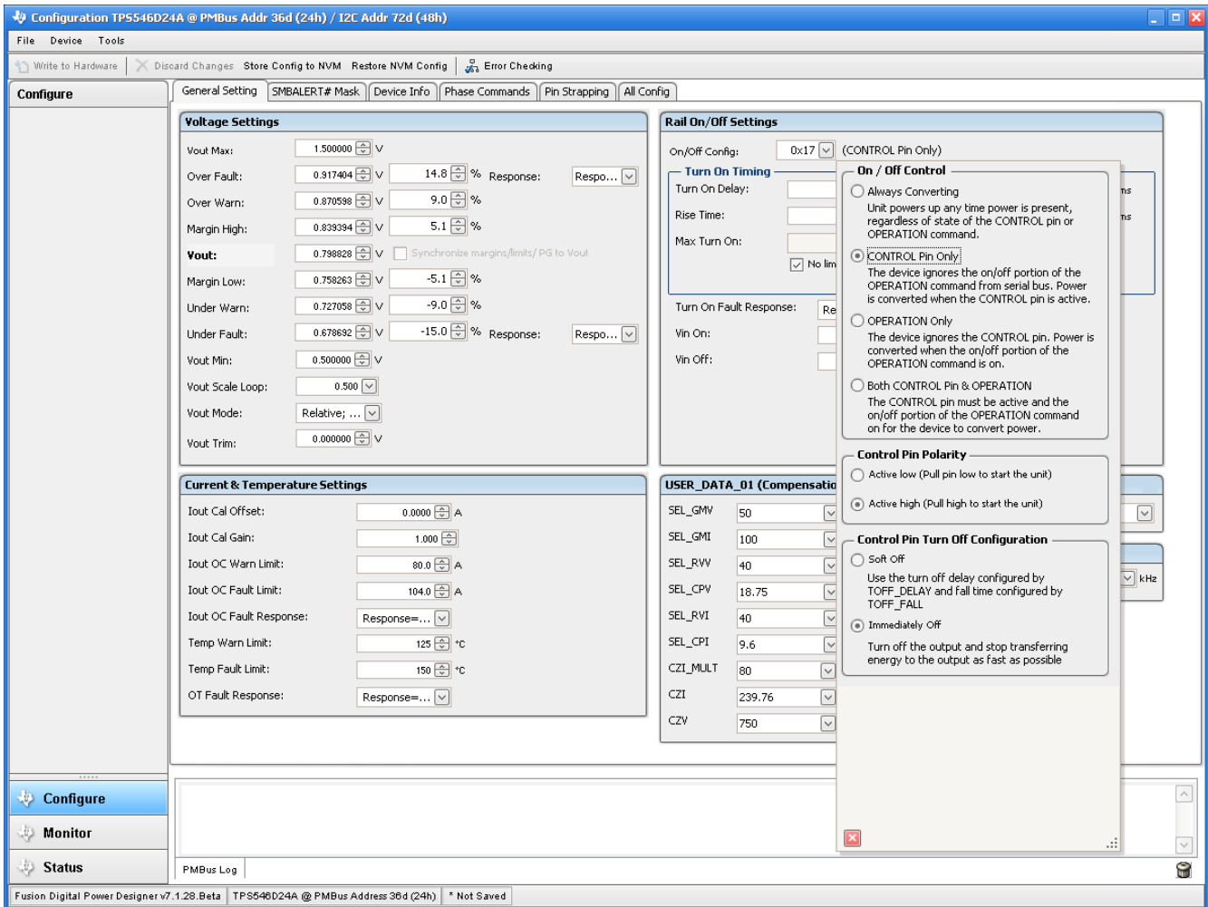
图 10-3. 配置 - ON_OFF_CONFIG
