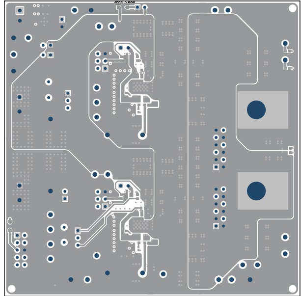
图 8-12. TPS546B24AEVM-2PH 内底层 (顶视图)
