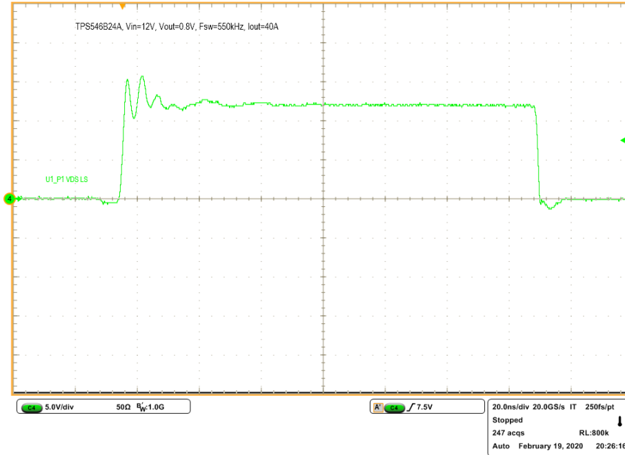
图 7-9. 低侧 MOSFET V_{DS}
