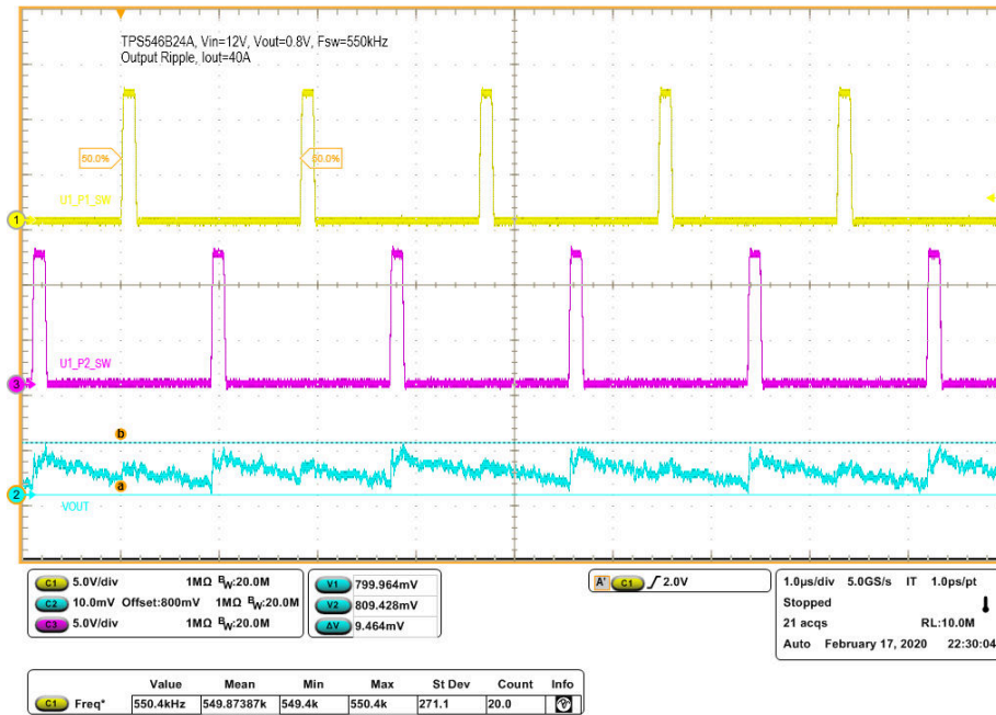
图 7-8. 40A 负载时的输出纹波
