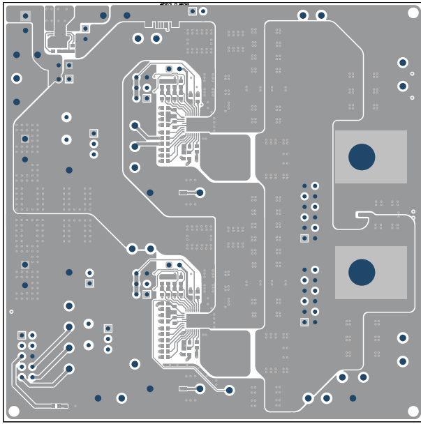
图 8-5. TPS546B24AEVM-2PH 顶层铜 (顶视图)
