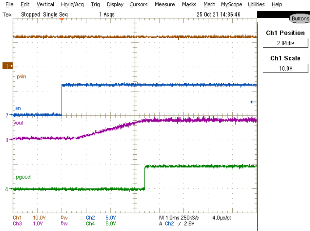
图 7-8. 控制的开启，70A CC 负载
