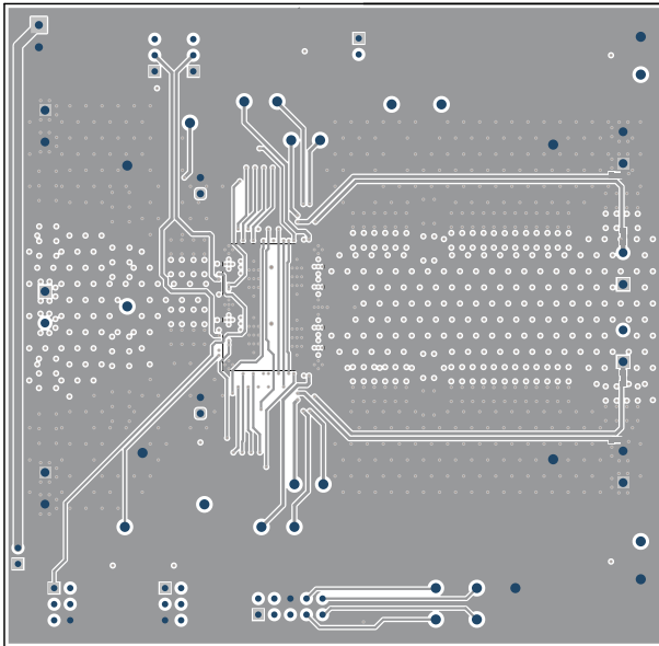
图 8-7. TPSM8D6C24EVM-2PH 内层 4 ( 顶视图 )
