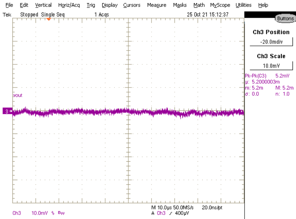
图 7-6. 输出纹波，空载
