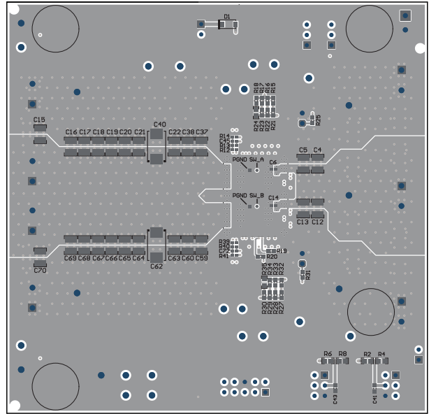
图 8-2. TPSM8D6C24EVM-2PH 底面元件视图 (底视图)
