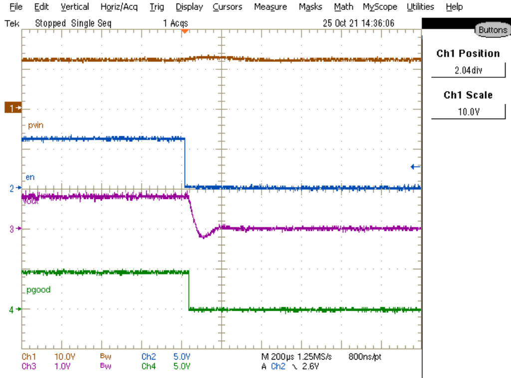
图 7-9. 关闭控制，70A CC 负载
