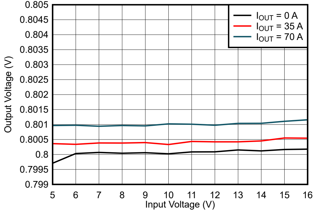
图 7-3. 线路调节
