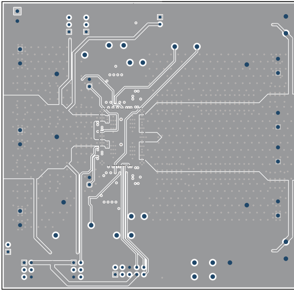
图 8-5. TPSM8D6C24EVM-2PH 内层 2 ( 顶视图 )
