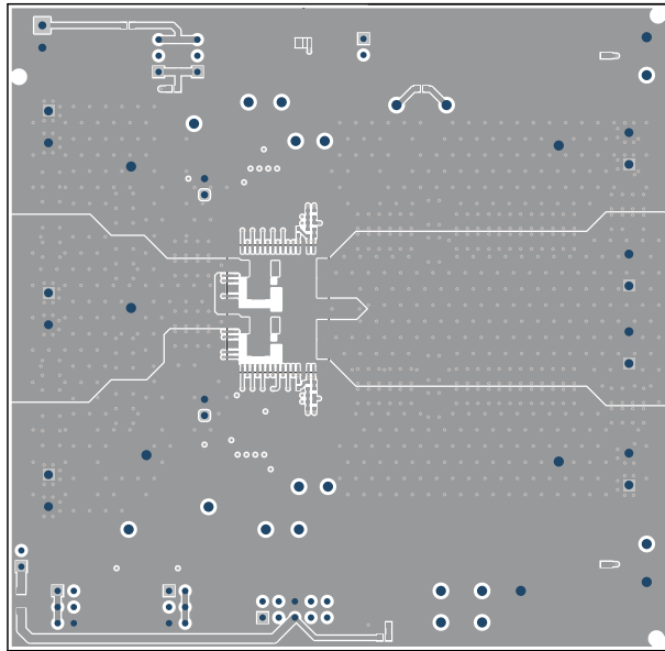
图 8-3. TPSM8D6C24EVM-2PH 顶层铜 (顶视图)
