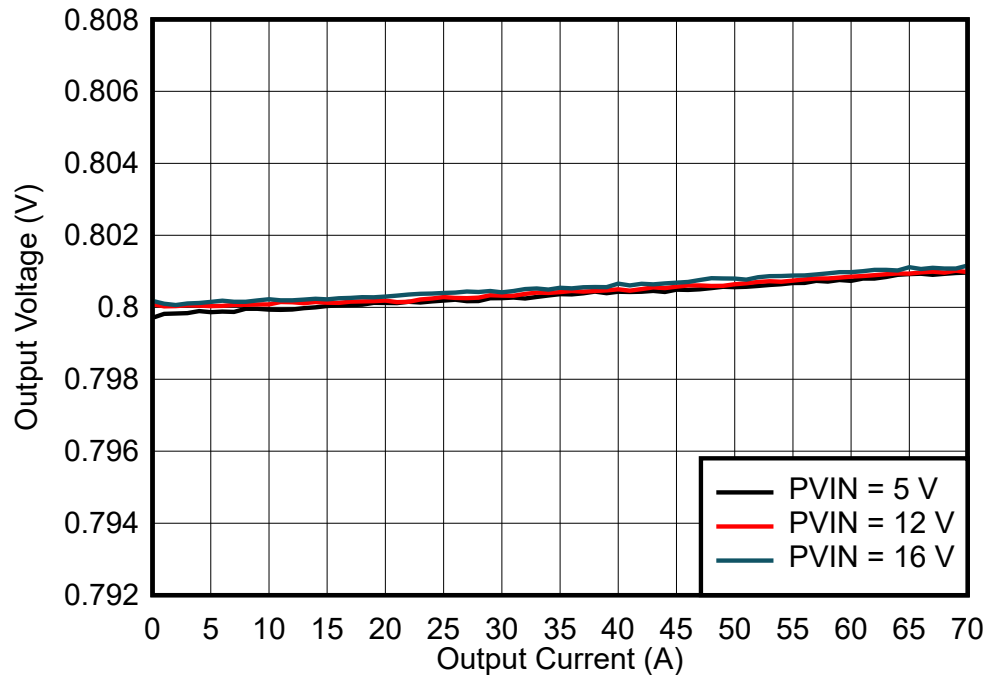
图 7-2. 负载调节
