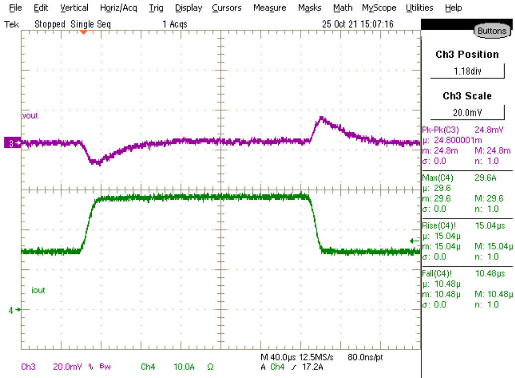
图 7-4. 瞬态响应
