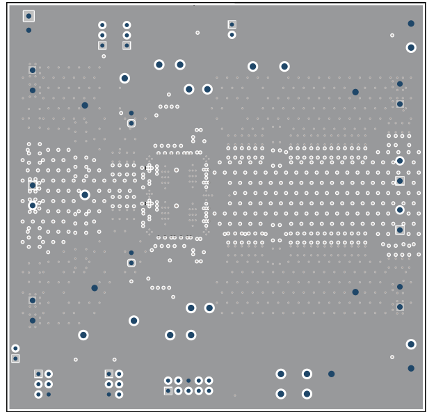
图 8-4. TPSM8D6C24EVM-2PH 内层 1 (顶视图)
