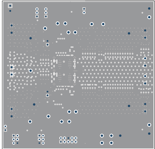
图 8-8. TPSM8D6C24EVM-2PH 内层 5 ( 顶视图 )
