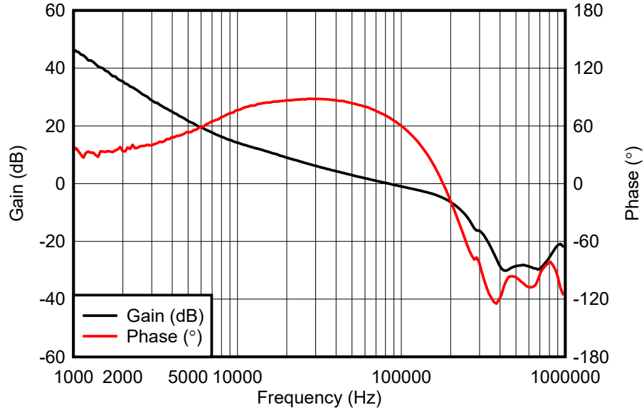
图 7-5. 波特图，70A 负载
