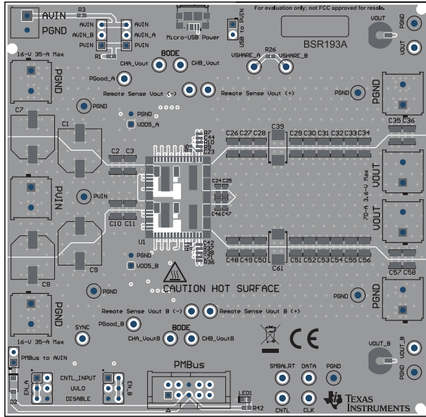
图 8-1. TPSM8D6C24EVM-2PH 顶面元件视图 (顶视图)
