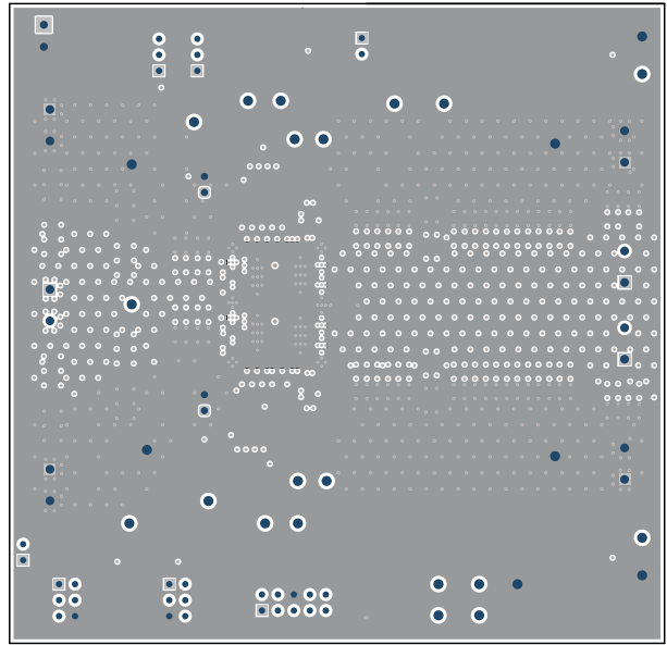
图 8-6. TPSM8D6C24EVM-2PH 内层 3 ( 顶视图 )
