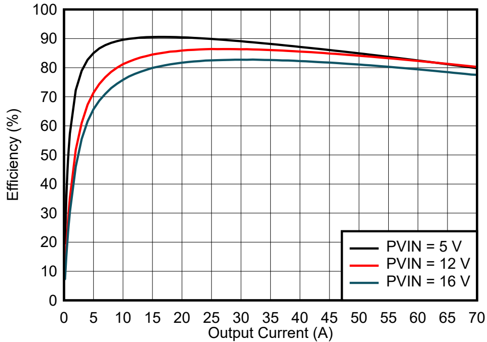
图 7-1. 效率
