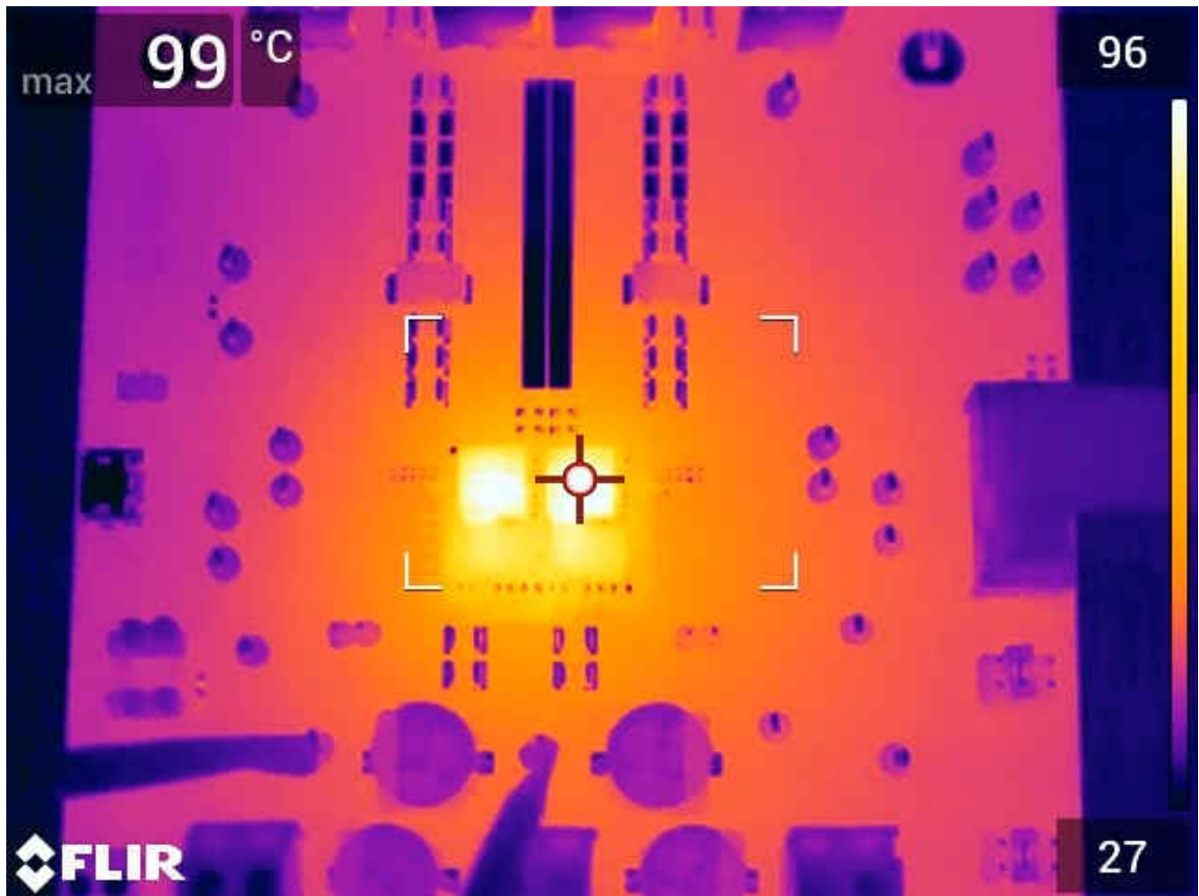
图 7-10. 热像图
