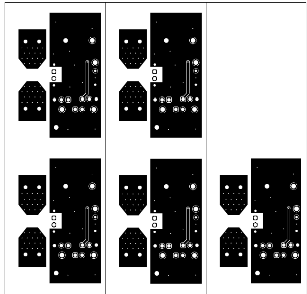
图 6-5. INA296EVM 底层
