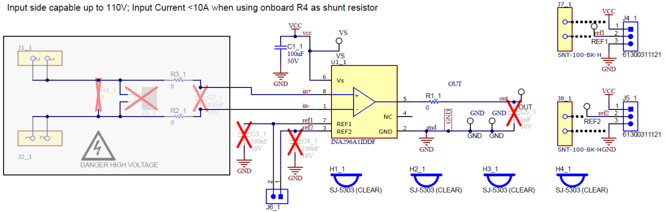
图 6-1. INA296EVM 原理图：增益选项 1 面板
