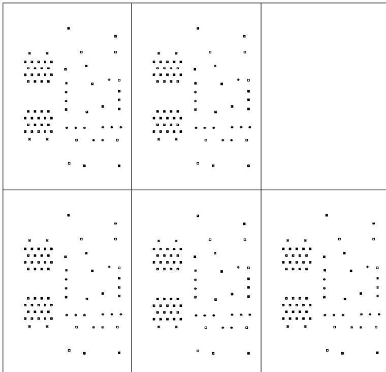
图 6-8. INA296EVM 钻孔图
