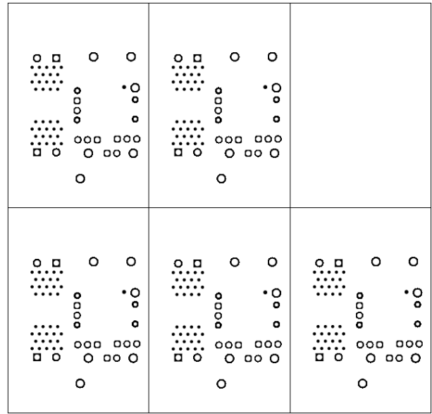
图 6-7. INA296EVM 底部阻焊层
