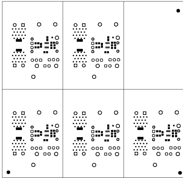
图 6-6. INA296EVM 顶部阻焊层
