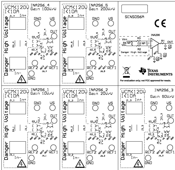
图 6-2. INA296EVM 顶部覆盖层
