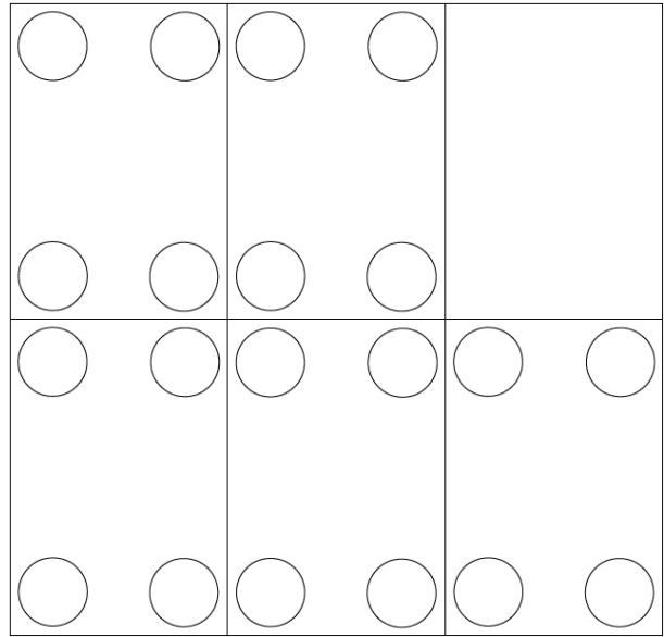
图 6-3. INA296EVM 底部覆盖层
