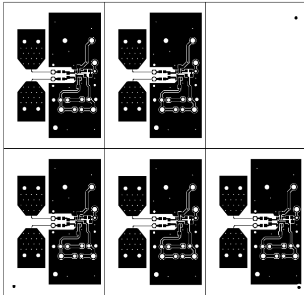
图 6-4. INA296EVM 顶层
