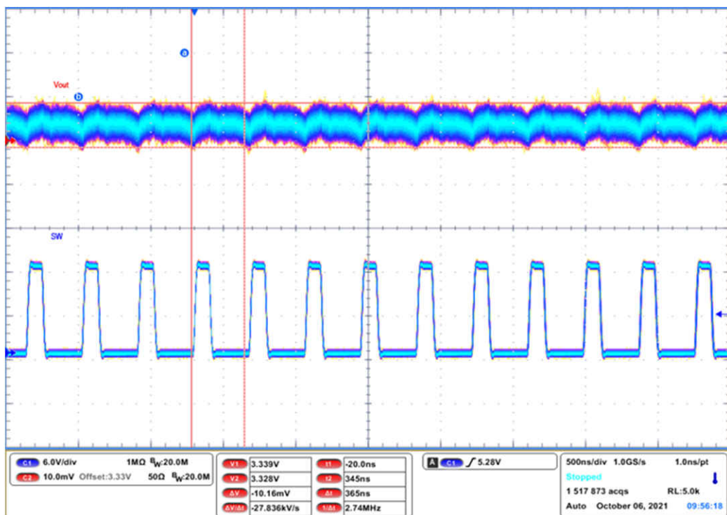
图 5-6. 输出电压纹波，强制 PWM ( V_{IN} = 12V , V_{OUT} = 3.3V , I_{OUT} = 300mA )
