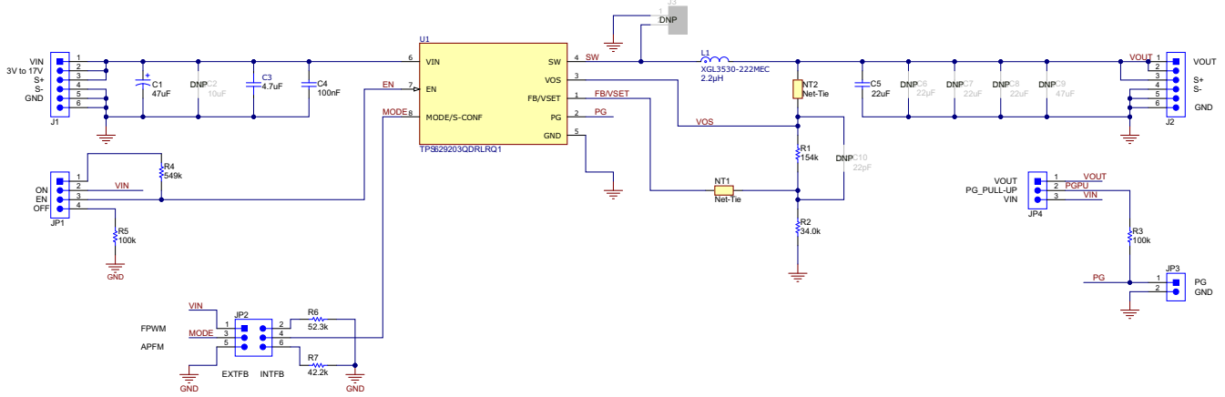
图 7-1. TPS629203-Q1EVM 原理图
