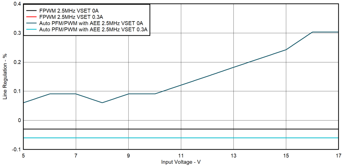
图 5-3. 线路调节 ( V_{IN} = 5V - 17V , V_{OUT} = 3.3V , I_{OUT} = 0A 和 300mA , F_{SW} = 2.5MHz )
