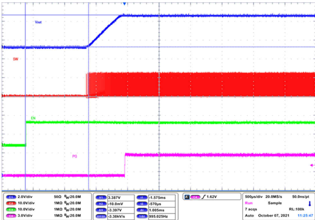
图 5-8. 启用启动，强制 PWM ( V_{IN} = 12V , V_{OUT} = 3.3V , I_{OUT} = 300mA )
