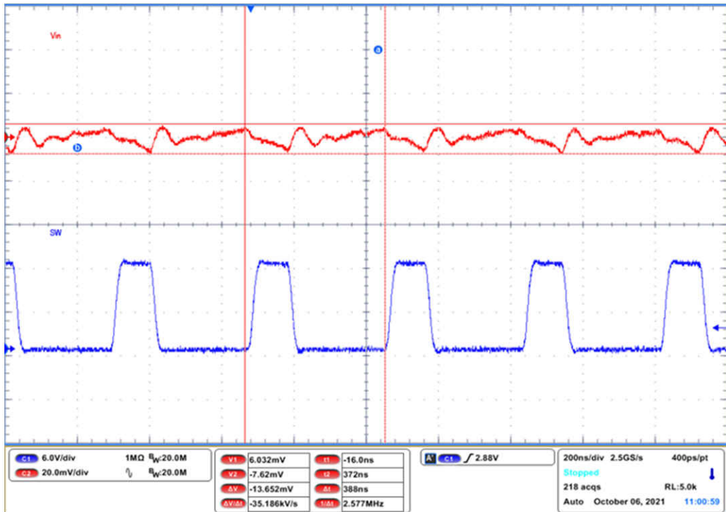
图 5-7. 输入电压纹波，强制 PWM ( V_{IN} = 12V , V_{OUT} = 3.3V , I_{OUT} = 300mA )
