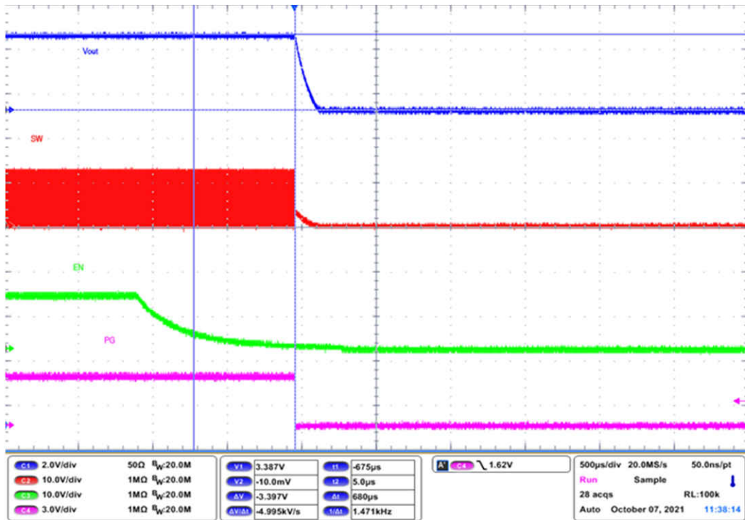
图 5-9. 启用关断，强制 PWM ( V_{IN} = 12V , V_{OUT} = 3.3V , I_{OUT} = 300mA )
