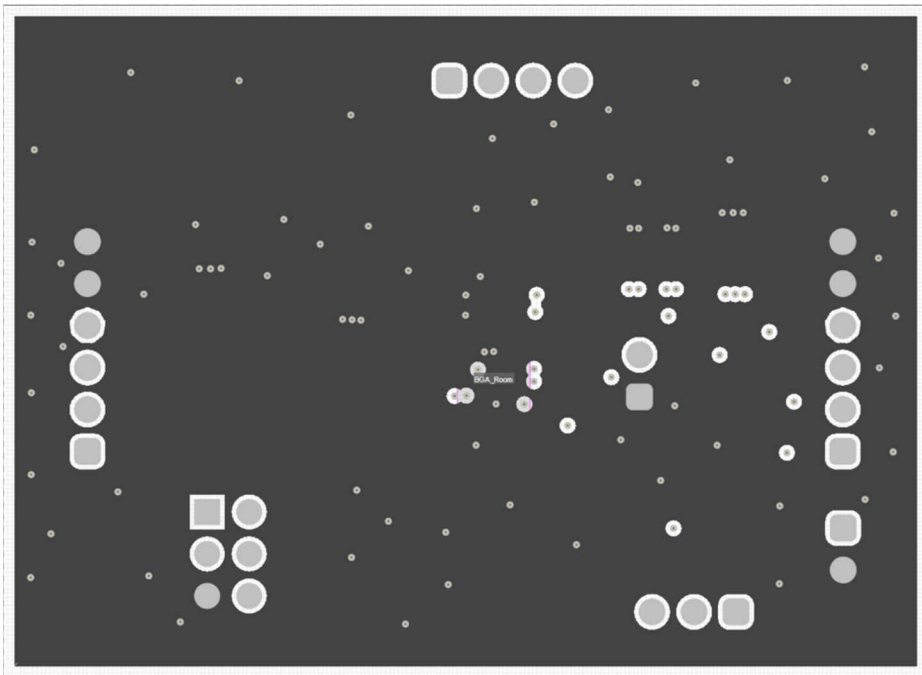
图 6-3. 内层 1
