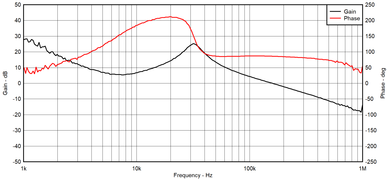
图 5-4. 环路响应，强制 PWM VSET ( V_{IN} = 12V , V_{OUT} = 3.3V , I_{OUT} = 300mA )
