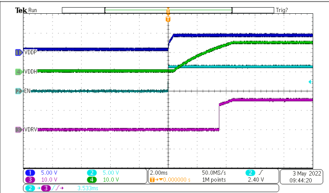
图 3-4. 两线模式开启
