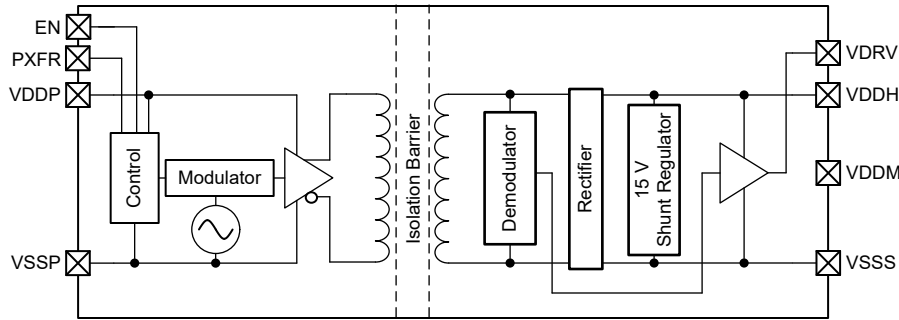
图 1-2. TPSI3052-Q1 功能方框图
