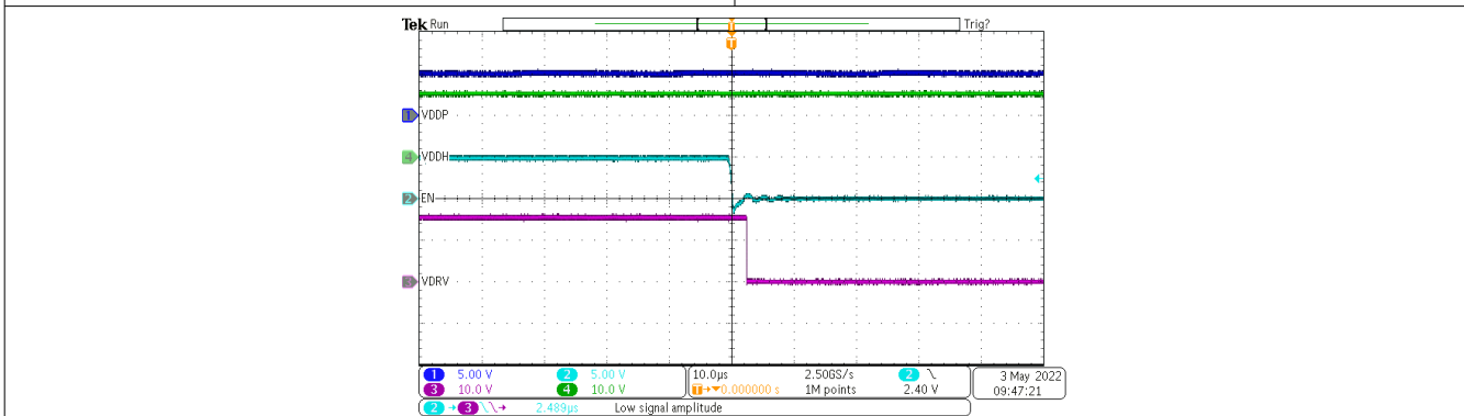
图 3-11. 三线模式关闭
