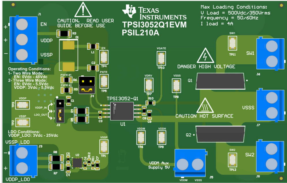
图 1-1. PCB 视图
