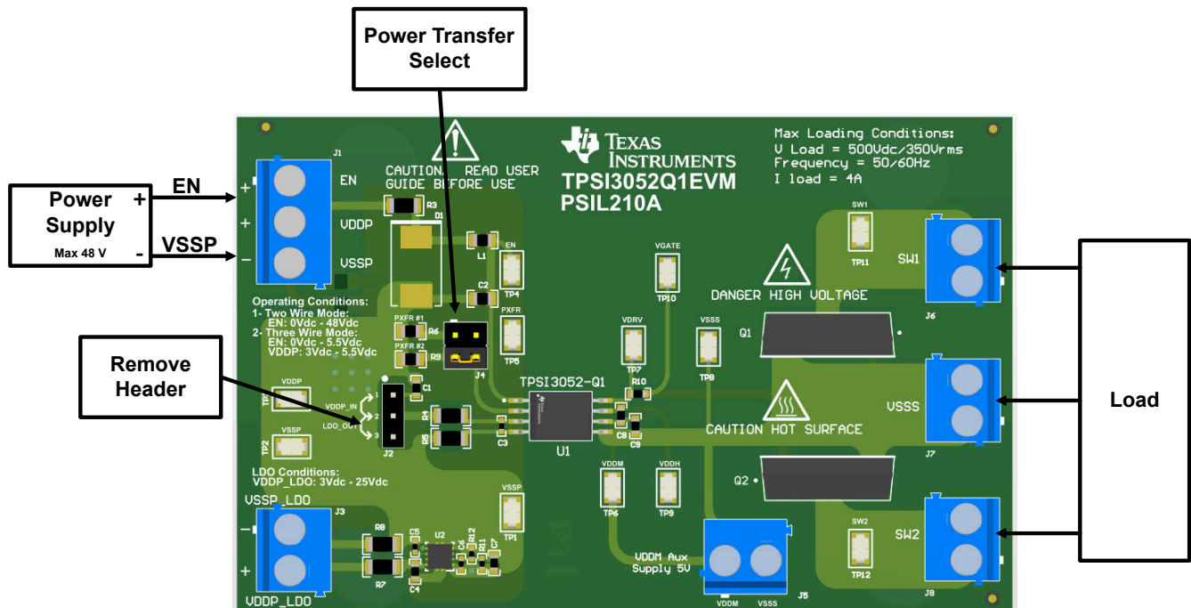
图 3-2. 两线模式设置
