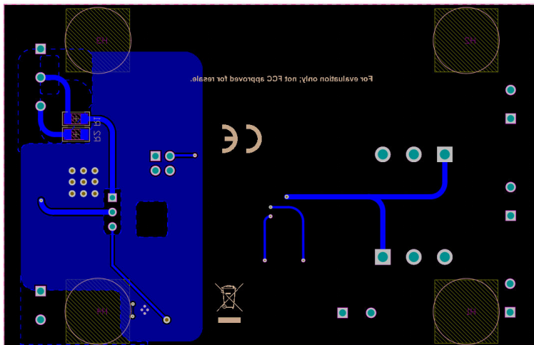
图 6-3. PCB 底层
