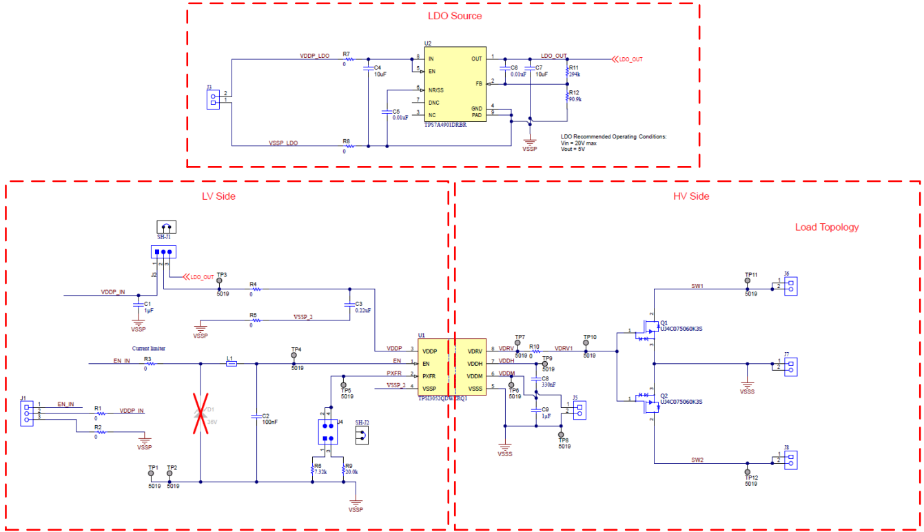
图 5-1. PSIL210 原理图
