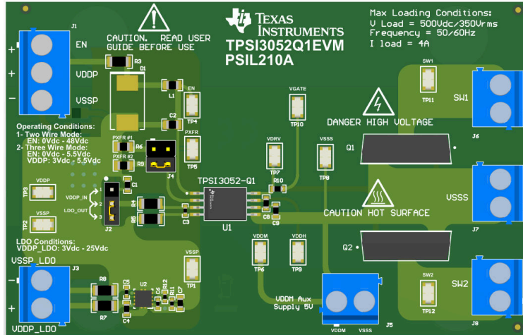
图 6-1. 3D 视图
