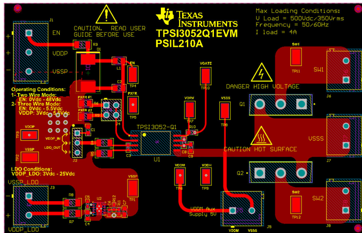
图 6-2. PCB 顶层
