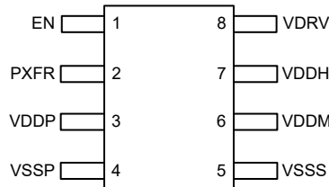
图 1-3. TPSI3052-Q1、TPSI3052S-Q1 DWZ 封装 8 引脚 SOIC 顶视图
