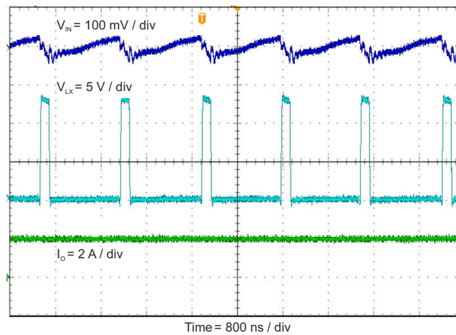
图 4-9. 输入电压纹波, I OUT = 2A
