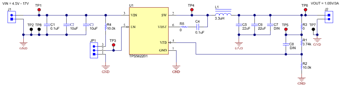
图 6-1. TPS562201EVM-715 原理图
