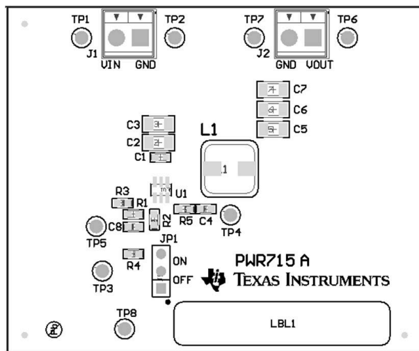
图 5-1. 顶层装配图
