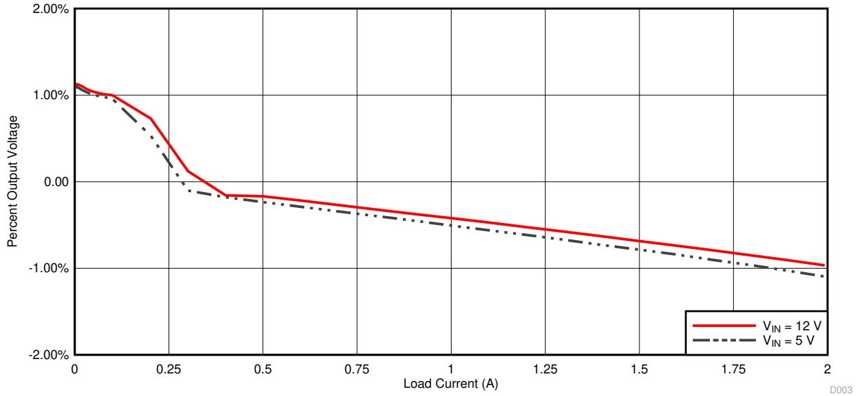
图 4-3. 负载调节
