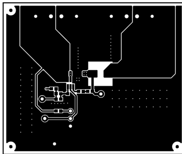
图 5-2. 顶层
