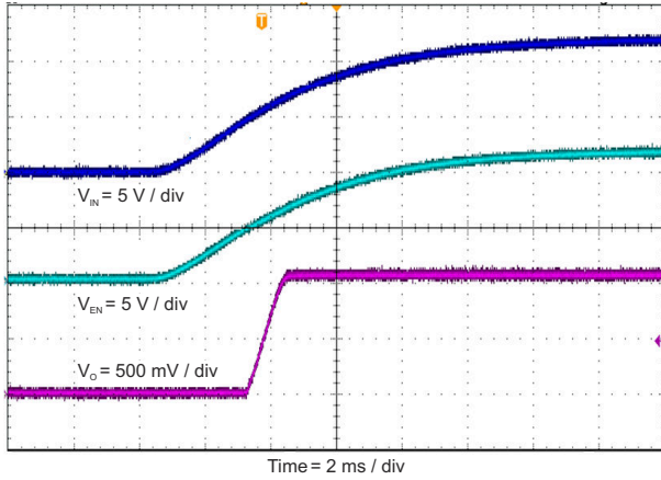
图 4-10. 相对于输入电压的启动
