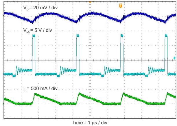
图 4-7. 输出电压纹波， I_{OUT} = 250 mA
