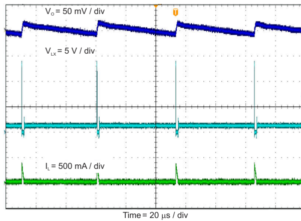
图 4-8. 输出电压纹波, I OUT = 10mA
