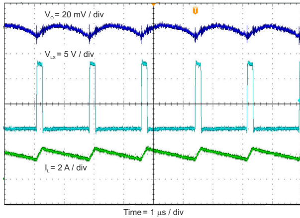
图 4-6. 输出电压纹波， I_{OUT} = 2A
