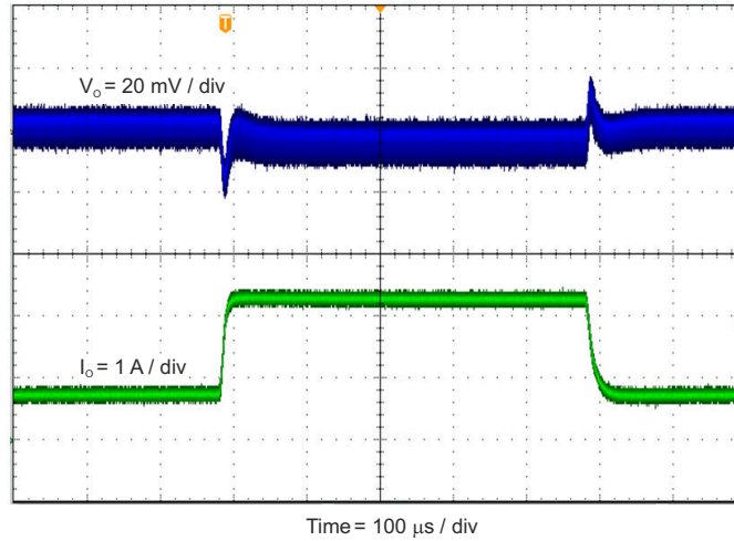
图 4-5. 负载瞬态响应，25% 至 75% 负载阶跃
