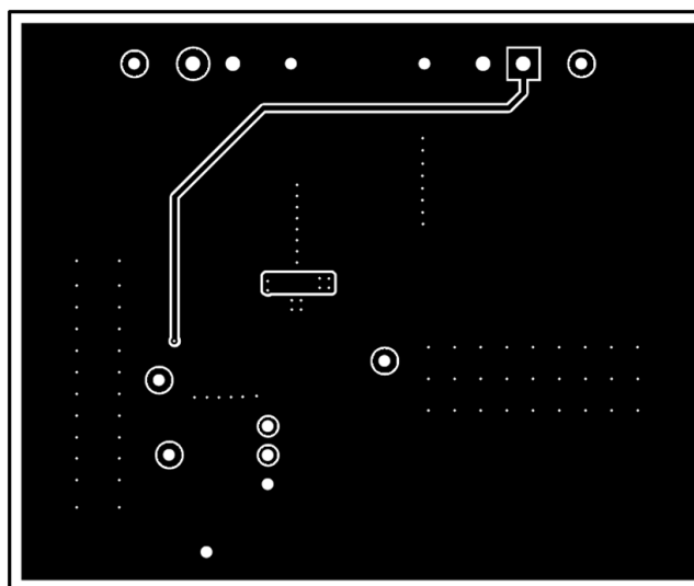
图 5-3. 底层
