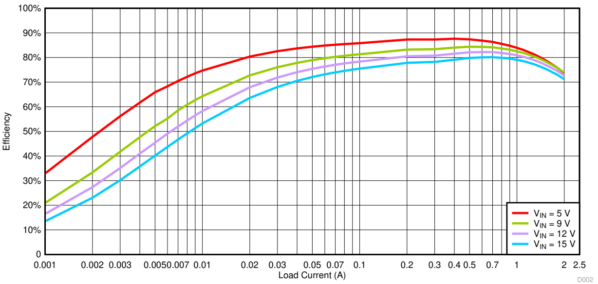
图 4-2. 轻负载效率
