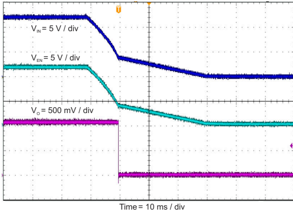
图 4-12. 相对于输入电压的关断
