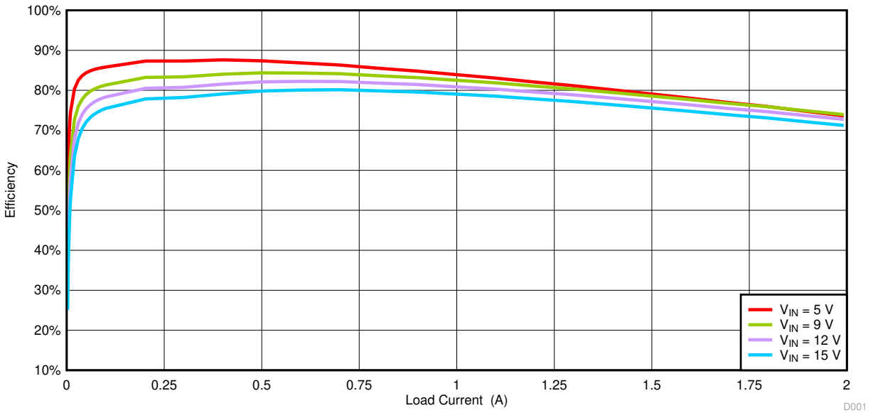
图 4-1. 效率
