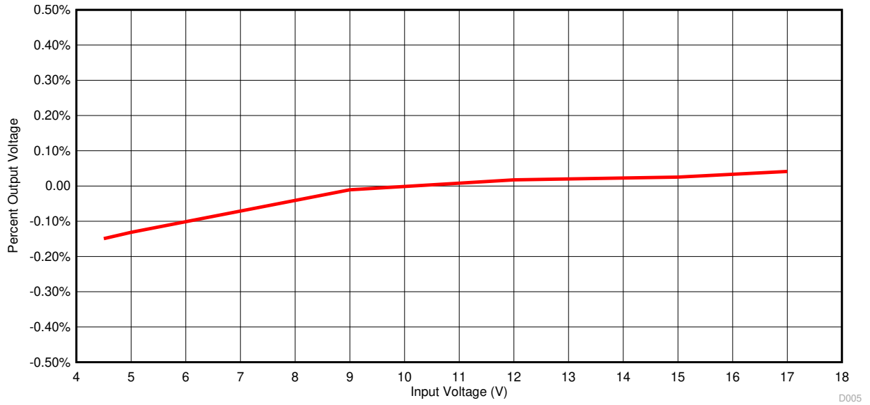
图 4-4. 线路调节
