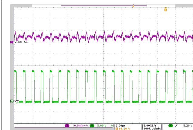
图 3-21. U2 输入纹波，空载
