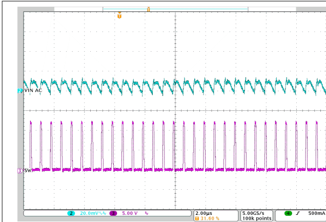
图 3-19. U1 输入纹波，空载
