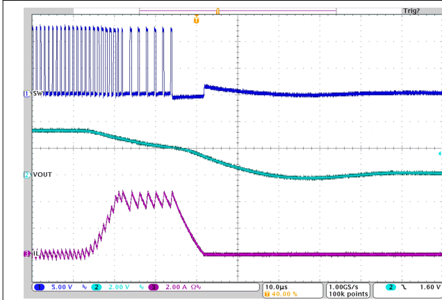
图 3-30. U2 输出过流保护 -
