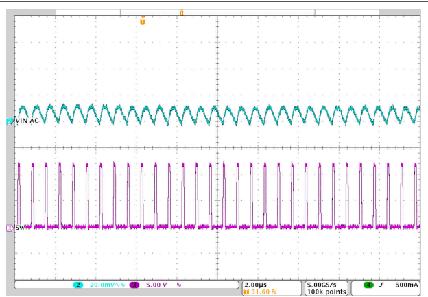
图 3-20. U1 输入纹波，3A 负载
