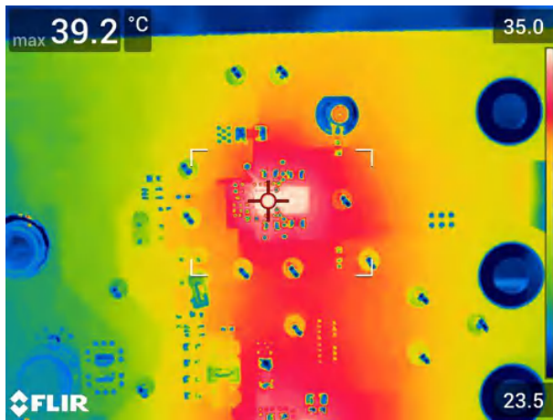
图 3-36. U1 热性能，两个 3A 负载
