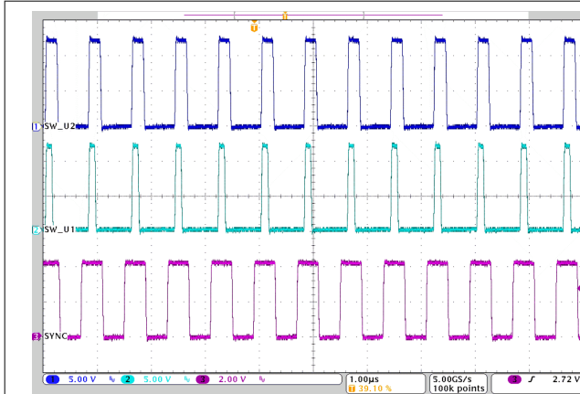
图 3-23. U1 和 U2 同步到时钟
