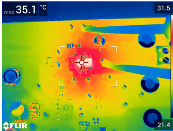
图 3-34. U1 热性能，3A 负载和 U2 关闭
