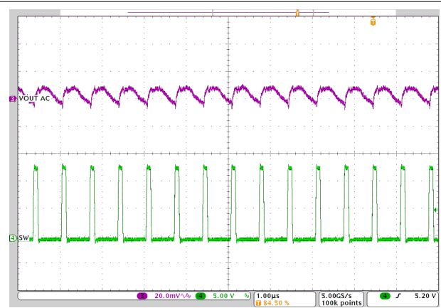
图 3-16. U1 输出纹波，3A 负载
