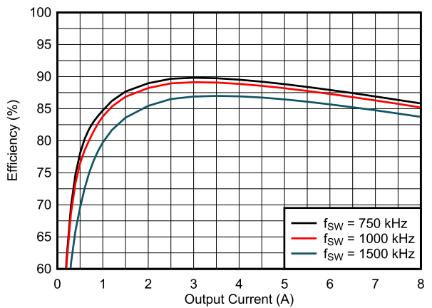
图 3-2. U2 效率 - 默认配置
