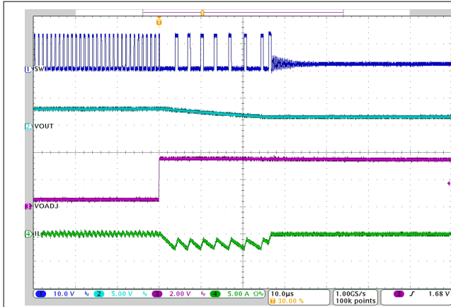
图 3-32. U2 过压保护
