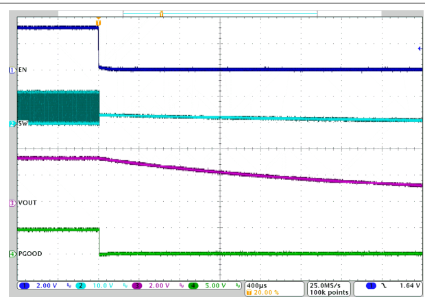
图 3-26. 通过 EN 关断 U2，空载
