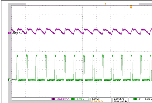
图 3-15. U1 输出纹波，空载
