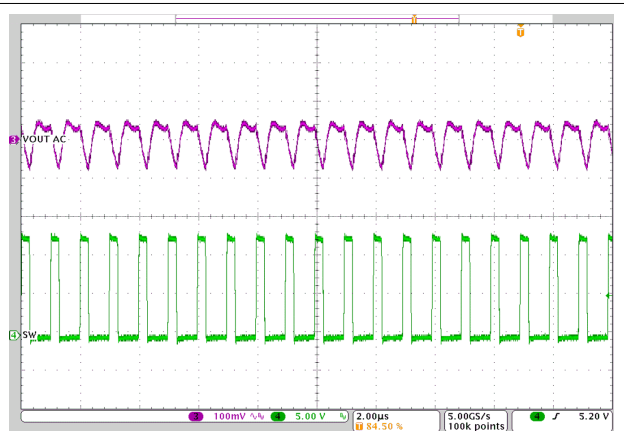
图 3-22. U2 输入纹波，3A 负载
