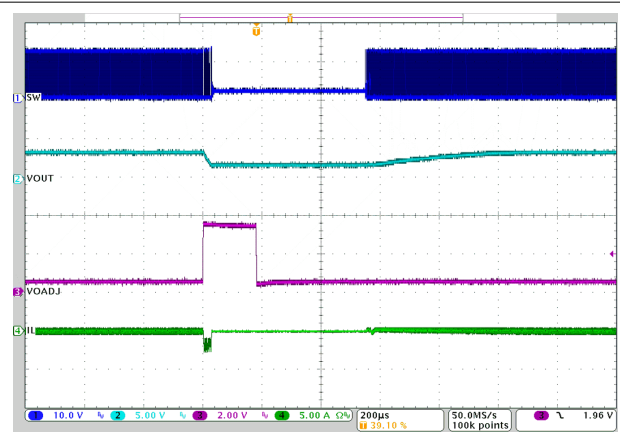
图 3-33. U2 OVP 和恢复
