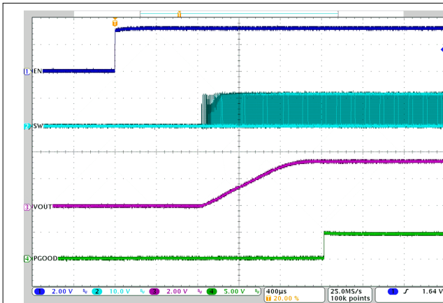
图 3-25. 通过 EN 启动 U2，空载
