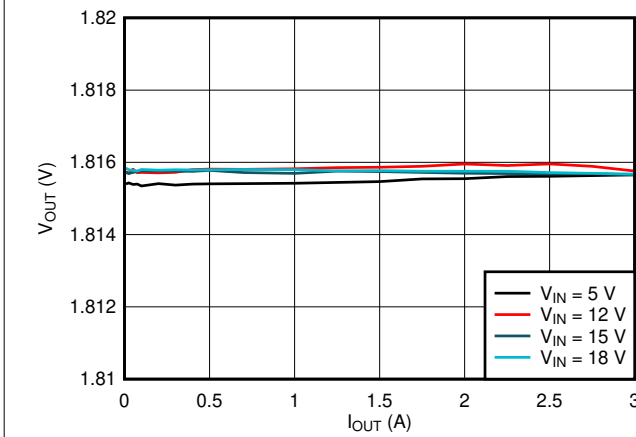
图 3-5. U1 负载调节
