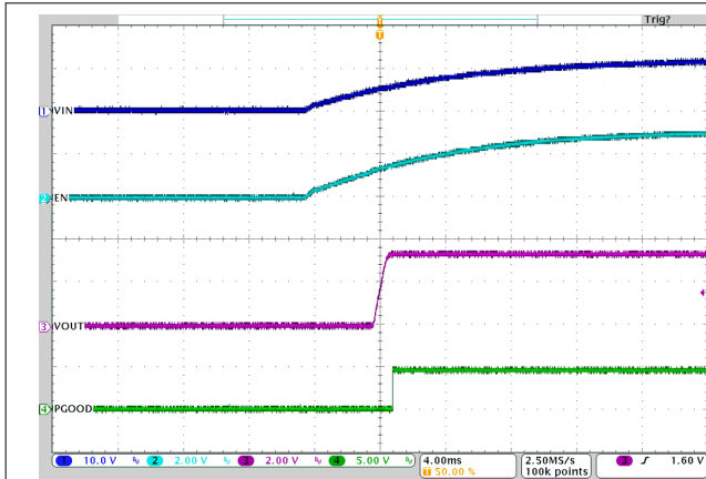
图 3-28. U2 在 VIN 1.5A 负载时启动
