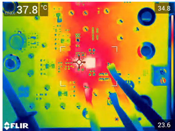
图 3-37. U2 热性能，两个 3A 负载
