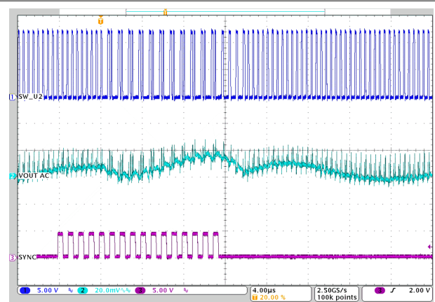
图 3-24. U2 时钟同步转换
