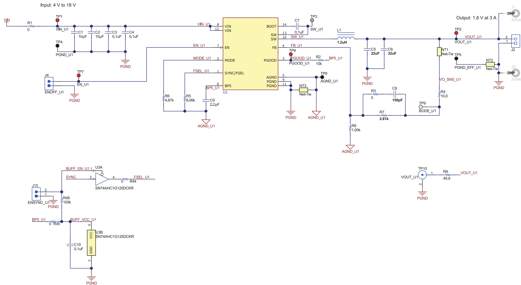
图 5-1. U1 原理图
