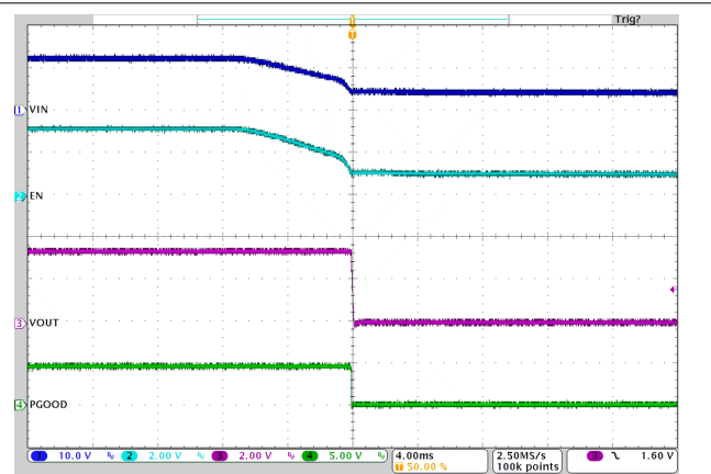
图 3-29. 在 1.5A 负载时通过 VIN 关断 U2
