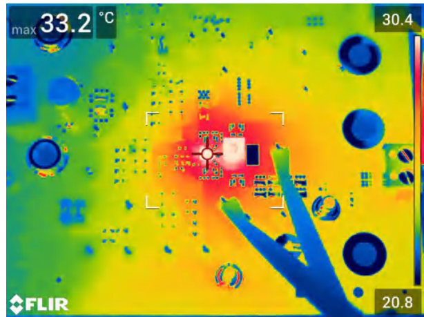
图 3-35. U2 热性能，3A 负载和 U1 关闭
