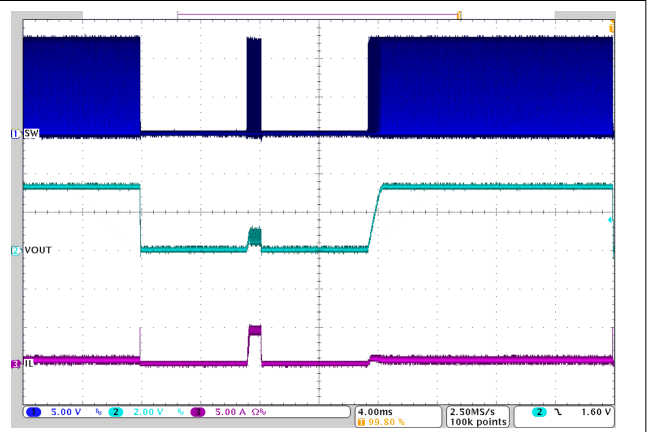
图 3-31. U2 OCP 断续和恢复
