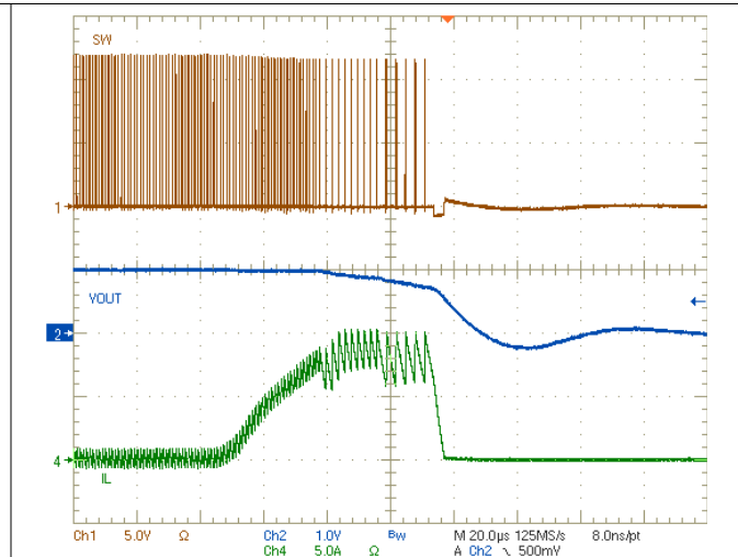
图 3-34. U2 输出过流保护 - 在低电流限制设置下过载
