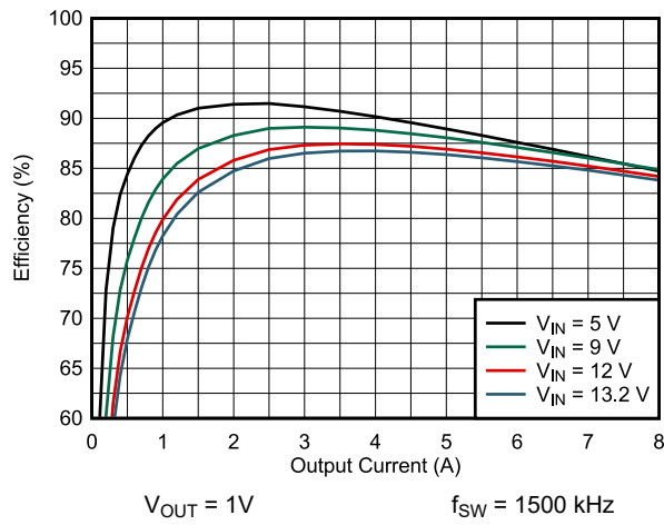
图 3-1. U1 效率
