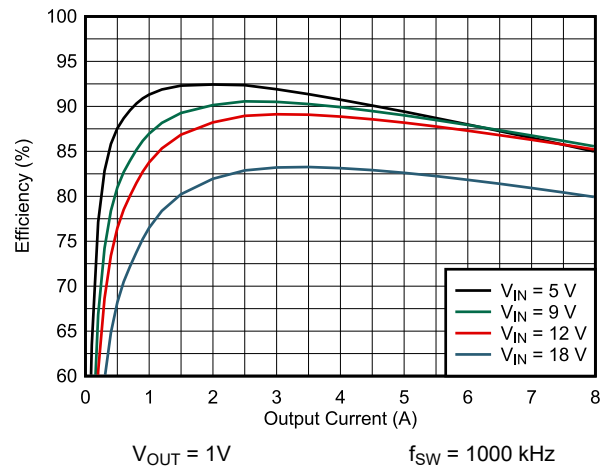
图 3-2. U2 效率 - 默认配置
