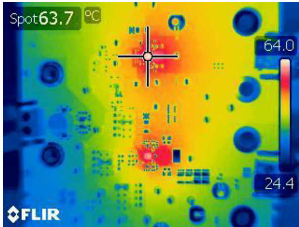
图 3-42. U1 热性能，两个 8A 负载
