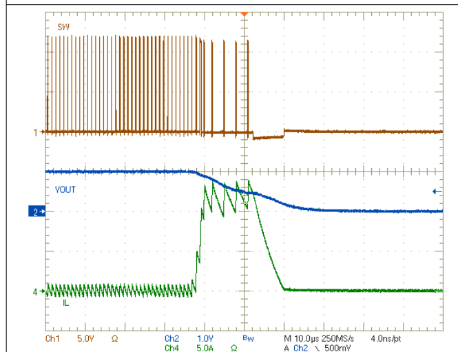
图 3-35. U2 输出过流保护 - 在高电流限制设置下短路
