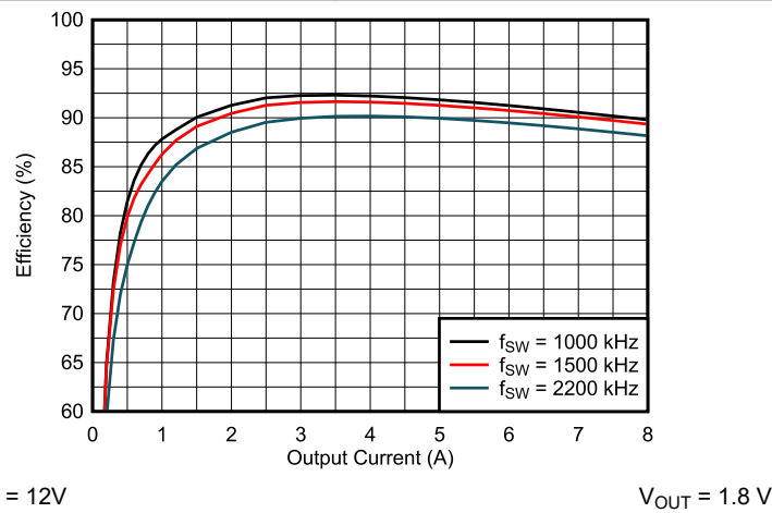
图 3-5. U2 效率 - 不同开关频率的 1.8V 输出
