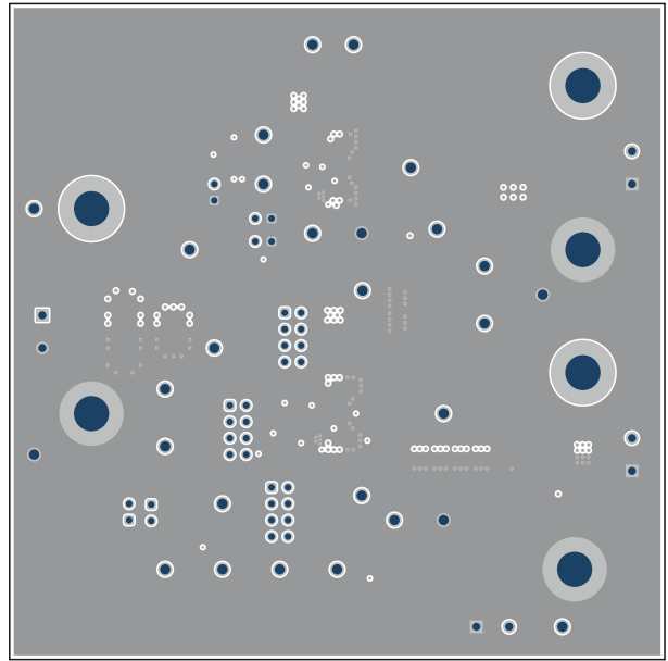
图 4-4. 中间层 1 布局
