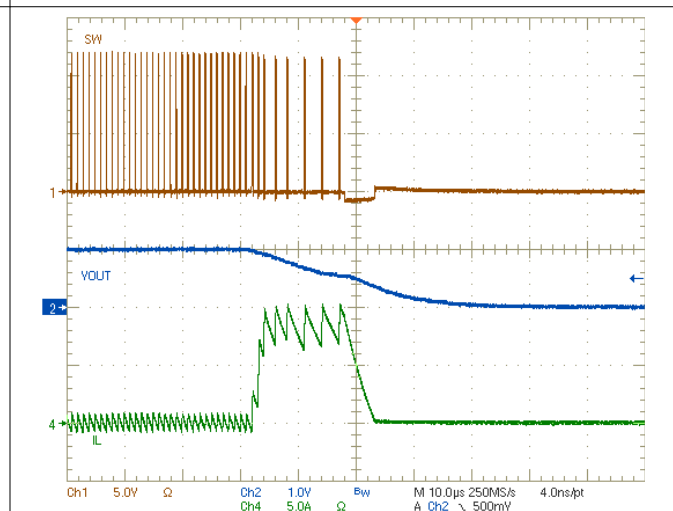
图 3-36. U2 输出过流保护 - 在低电流限制设置下短路
