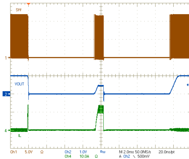
图 3-37. U2 OCP 断续和恢复 - 高电流设置
