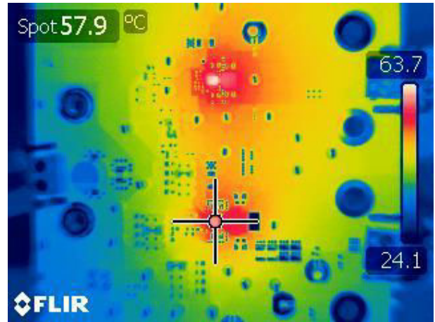
图 3-43. U2 热性能，两个 8A 负载
