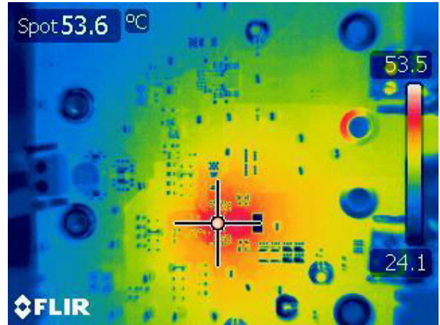
图 3-41. U2 热性能，8A 负载和 U1 关闭
