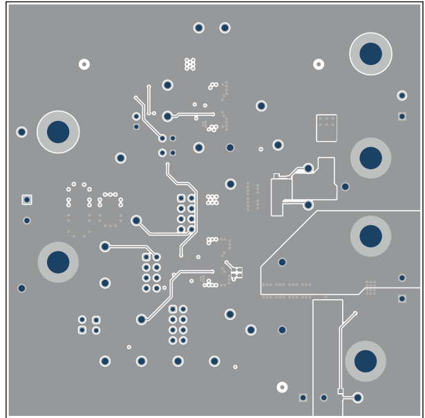
图 4-6. 底层布局
