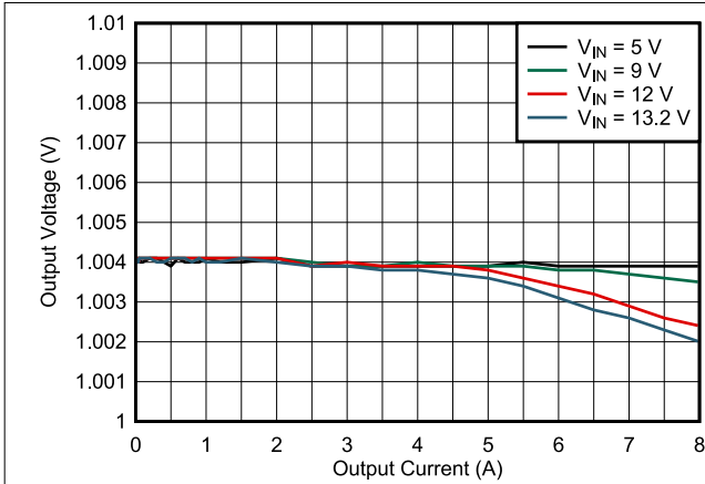
图 3-6. U1 负载调节
