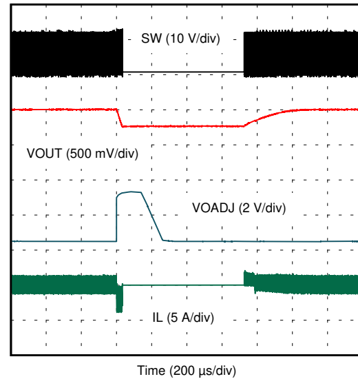
图 3-39. U2 OVP 和恢复
