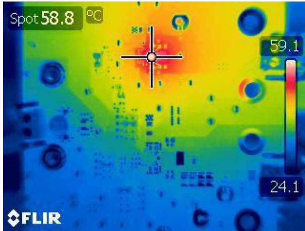
图 3-40. U1 热性能，8A 负载和 U2 关闭
