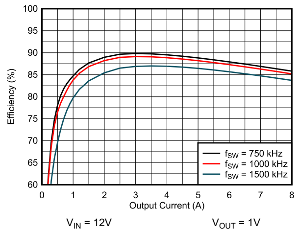
图 3-4. U2 效率 - 具有不同开关频率的 1V 输出
