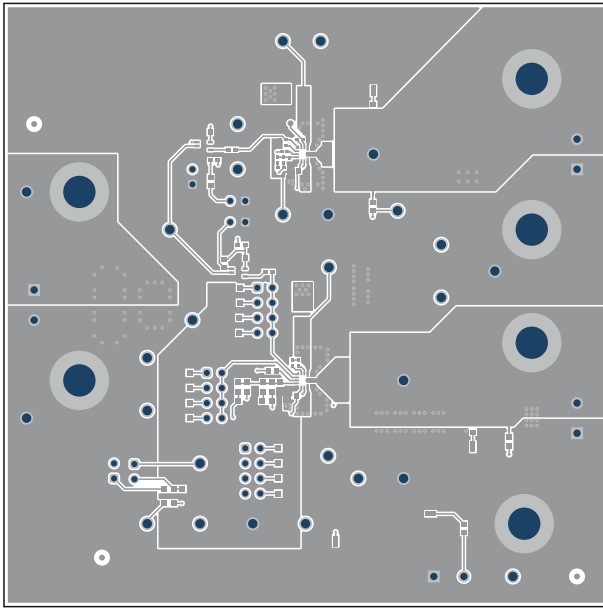
图 4-3. 顶层布局
