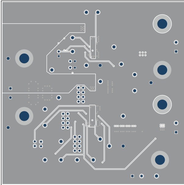
图 4-5. 中间层 2 布局
