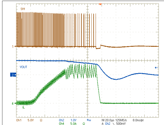
图 3-33. U2 输出过流保护 - 在高电流限制设置下过载
