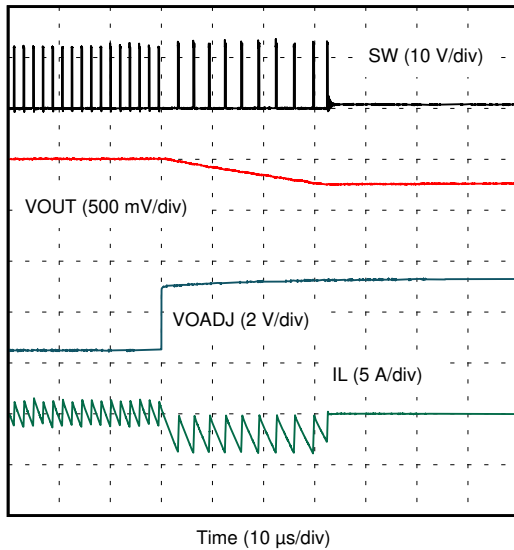
图 3-38. U2 过压保护
