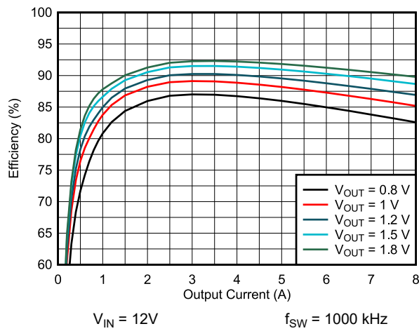
图 3-3. U2 效率 - 具有不同输出电压的 1000kHz 开关频率
